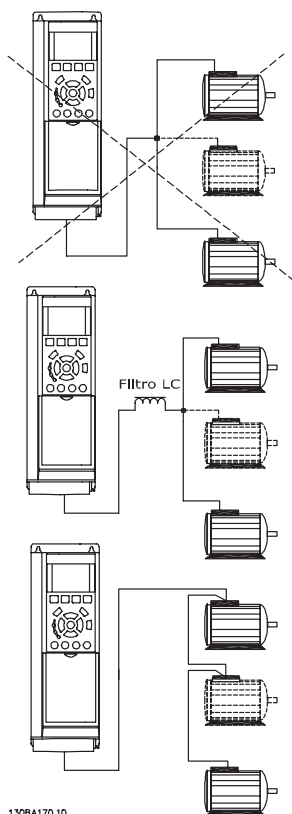
Illustration 4.45 Instalações com cabos conectados em uma junta comum.
