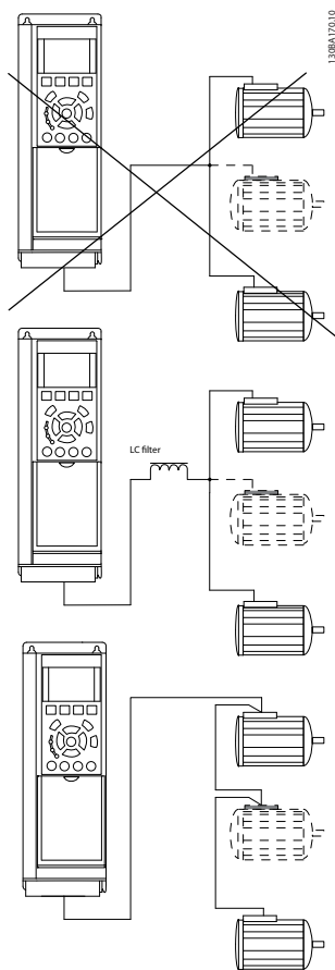
Illustration 4.45 공통 조인트에 연결된 케이블을 사용하여 설치한 경우
