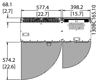
Illustration 4.10 IP21/IP54 외함 유형, 프레임 용량 D13 전면의 여유 공간.
