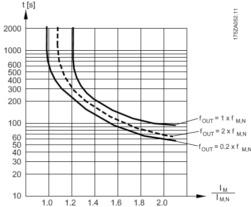
Illustration 6.6 ETR 프로파일
