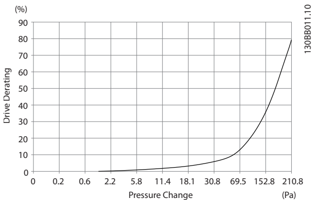
Illustration 4.16 E 프레임 용량 감소와 압력 변화 간 비교(대형 팬), P355-P450 인버터 통풍량: 850 cfm (1445 m 3 /h)
