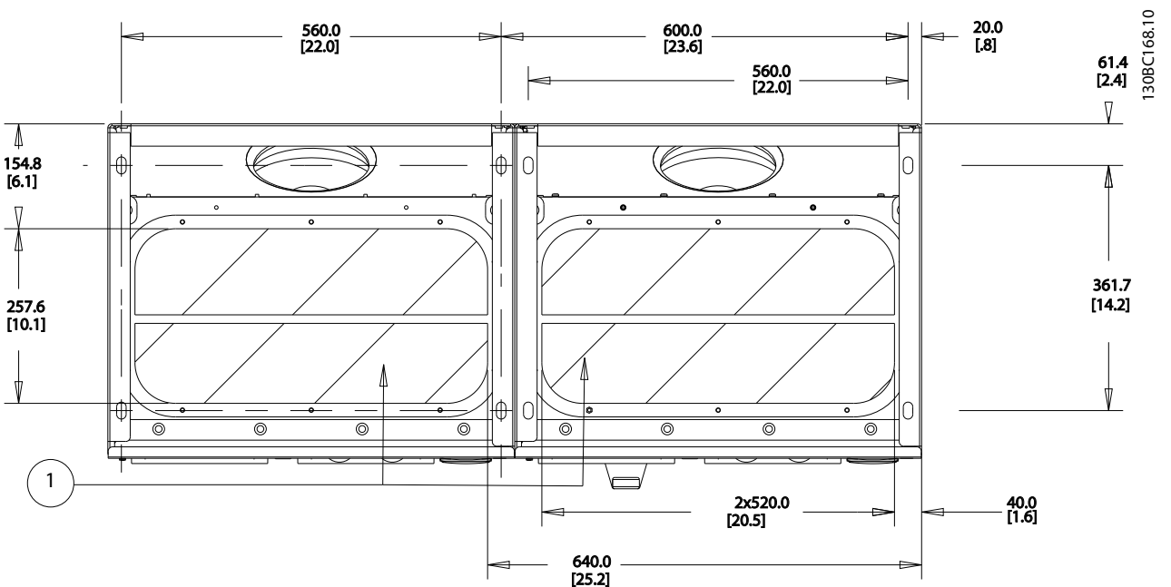
Illustration 4.20 프레임 용량 E9
