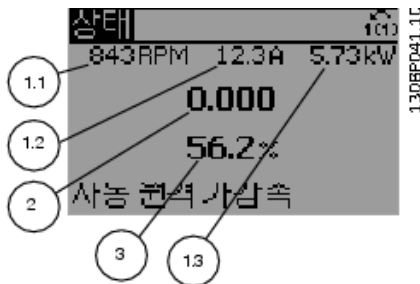
Illustration 5.2 상태 표시 I - 운전 변수
