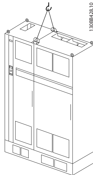
Illustration 4.5 들어 올리는 방법(권장), 프레임 용량 F18 - 인버터부
