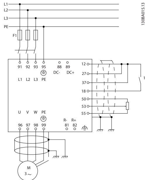
Illustration 4.1 주전원, 모터, 기동/정지 키 및 속도 조절용 가변 저항기 등 기본 설치를 나타내는 다이어그램.
