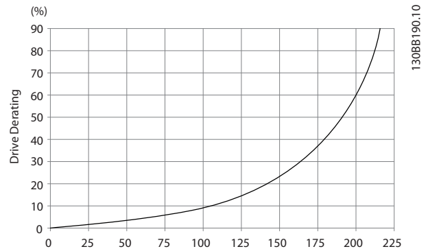
Illustration 4.17 F 프레임 용량 감소와 압력 변화 간 비교 인버터 통풍량: 580 cfm (985 m 3 /h)
