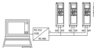
Illustration 5.16 연결 예.
