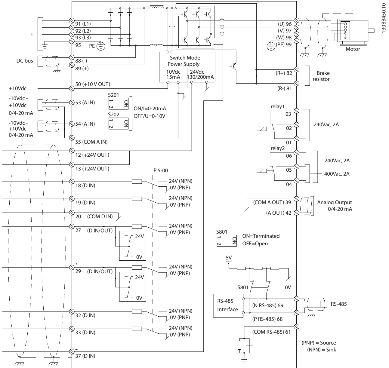
Illustration 4.39 옵션을 제외한 모든 전기 단자를 나타내는 다이어그램.
