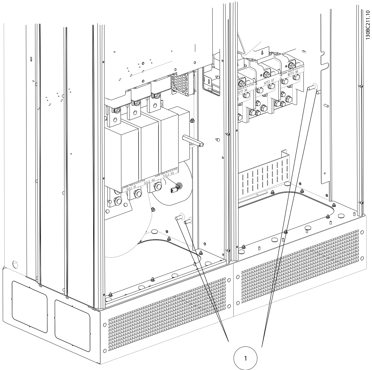
Illustration 4.28 접지 단자 위치
