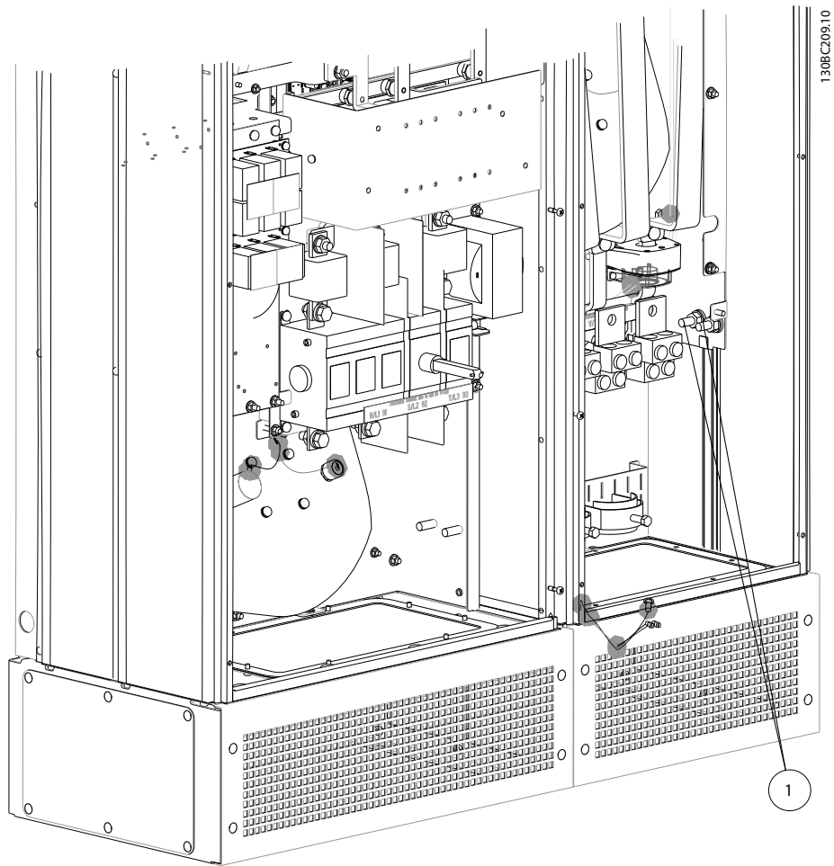
Illustration 4.26 접지 단자 위치
