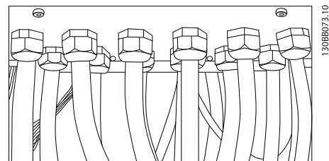
Illustration 4.18 글랜드 플레이트의 올바른 설치 예
