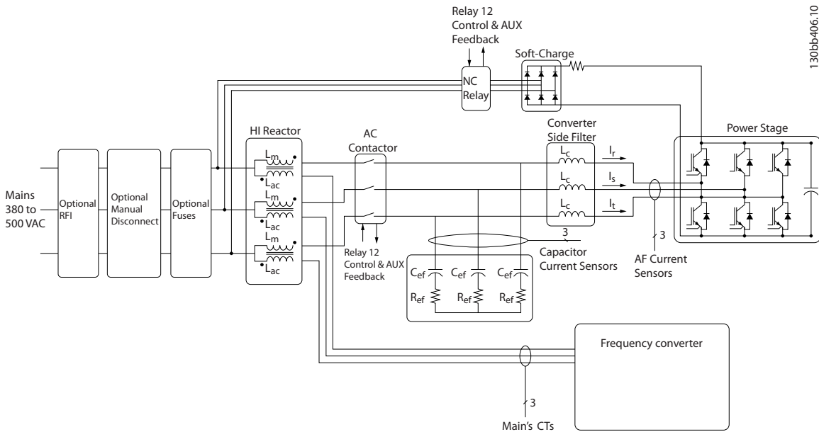
Illustration 3.1 최소 고조파 인버터를 위한 기본 설계
