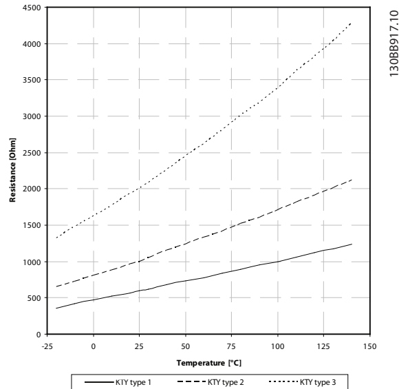
Illustration 6.5 KTY 유형 선택
