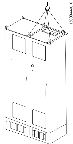
Illustration 4.4 들어 올리는 방법(권장), 프레임 용량 F18 - 필터부
