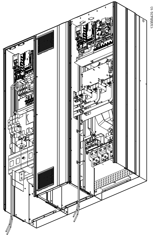
Illustration 4.33 E9의 제어 카드 배선 경로
