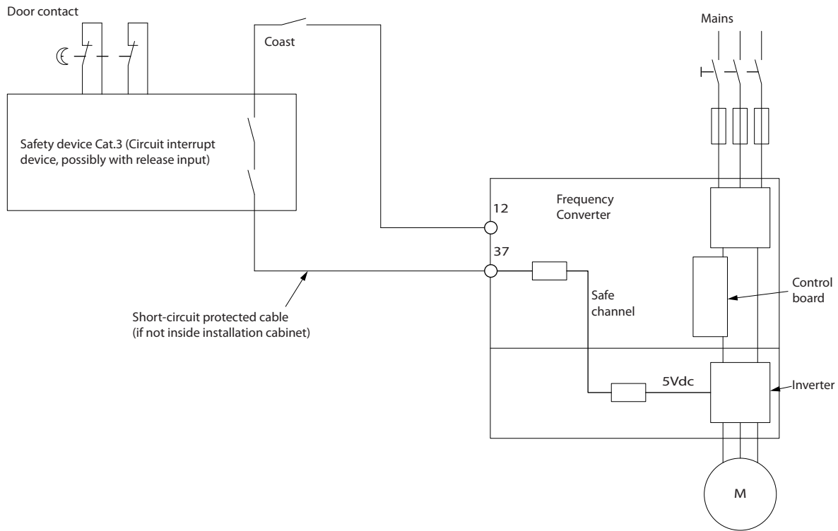
Illustration 2.2 안전 부문 3(EN 954-1)에 의거, 정지 부문 0(EN 60204-1)을 만족시키기 위한 설비의 필수 요소 그림.
