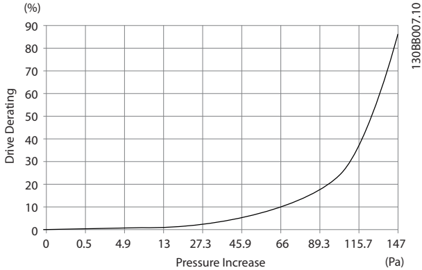
Illustration 4.14 D 프레임 용량 감소와 압력 변화 간 비교 인버터 통풍량: 450 cfm (765 m 3 /h)
