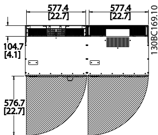
Illustration 4.11 IP21/IP54 외함 유형, 프레임 용량 E9 전면의 여유 공간.
