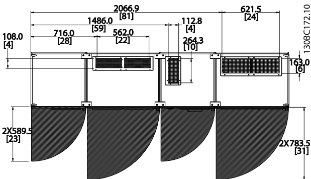
Illustration 4.12 IP21/IP54 외함 유형, 프레임 용량 F18 전면의 여유 공간.
