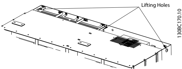
Illustration 4.3 들어 올리는 방법(권장), 프레임 용량 E9
