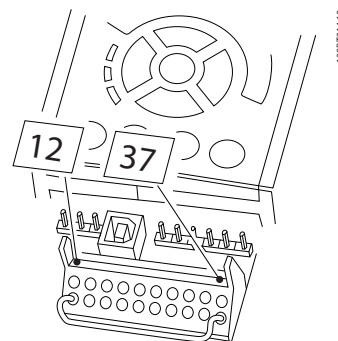
Illustration 2.1 단자 37 과 24V DC 간의 브리지 점퍼
