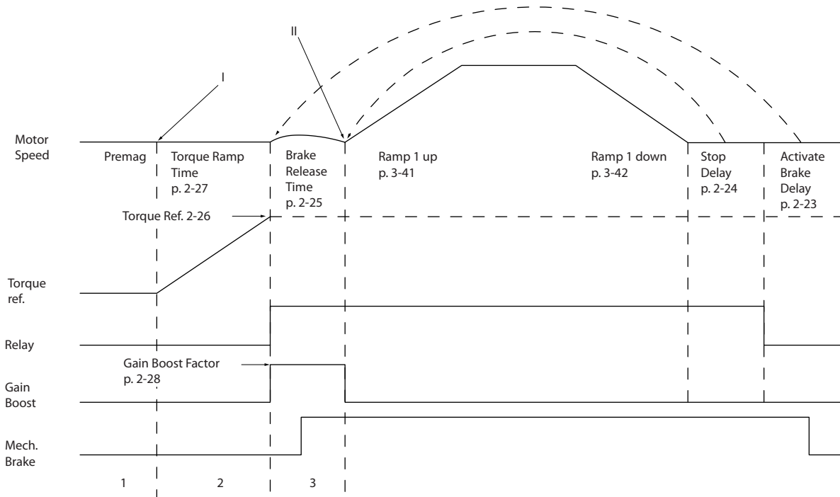
Illustration 6.9 호이스트 기계식 제동장치 제어를 위한 제동 해제 시퀀스
