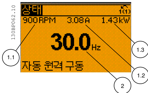
Illustration 5.3 상태 표시 II - 운전 변수
