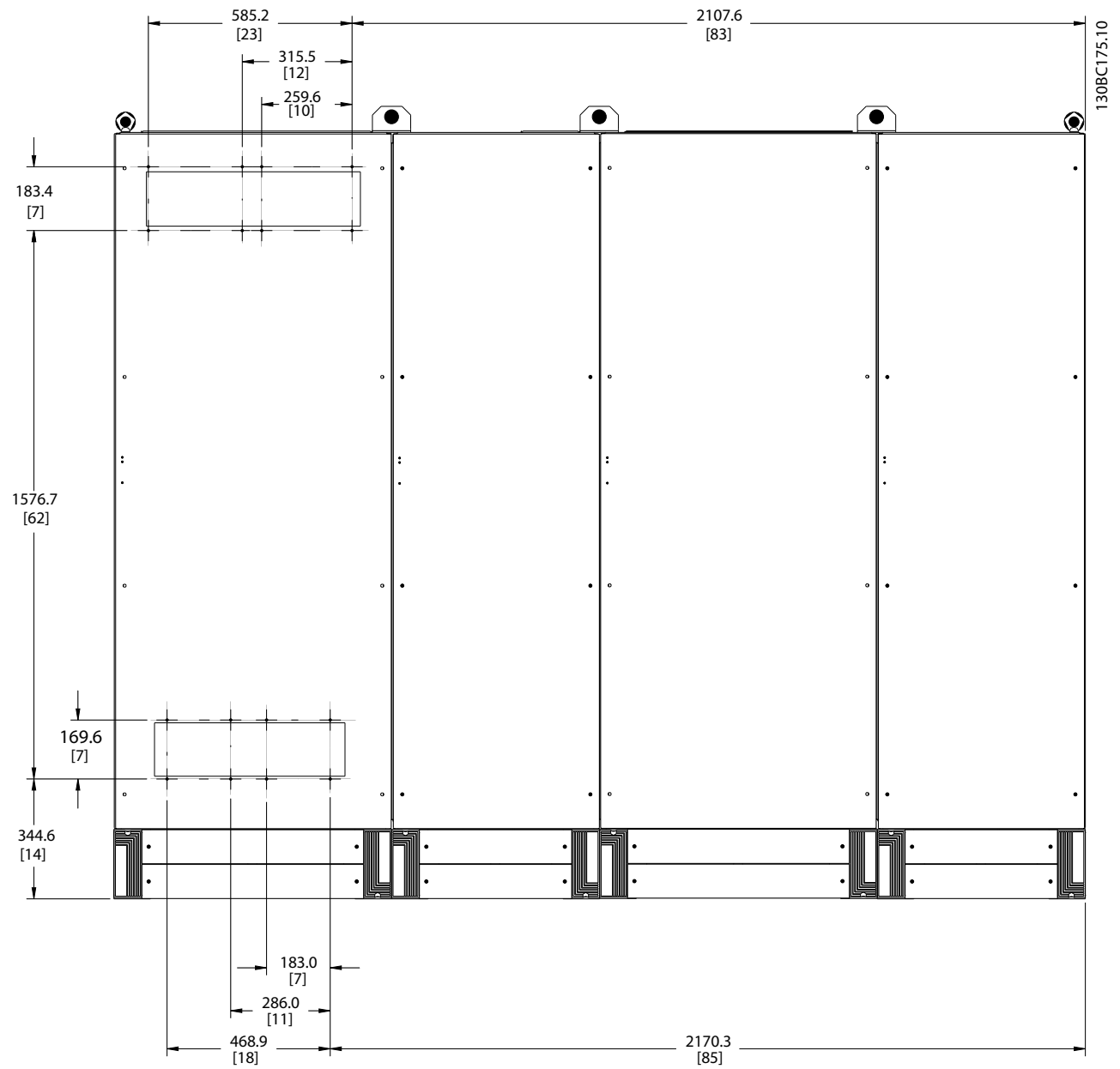
Illustration 4.9 프레임 용량 F18, 뒷면 보기
