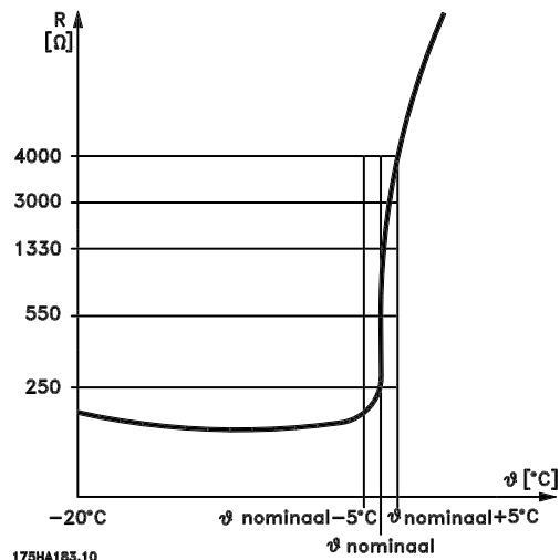
Illustration 6.2 PTC 프로파일
