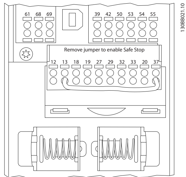
Illustration 7.2 제어카드 단자
