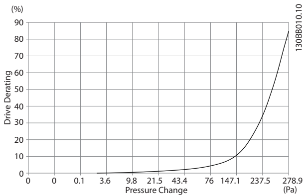
Illustration 4.15 E 프레임 용량 감소와 압력 변화 간 비교(소형 팬), P315 인버터 통풍량: 650 cfm (1105 m 3 /h)
