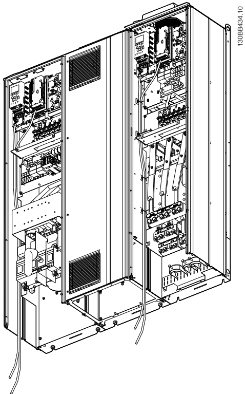
Illustration 4.32 D13의 제어 카드 배선 경로
