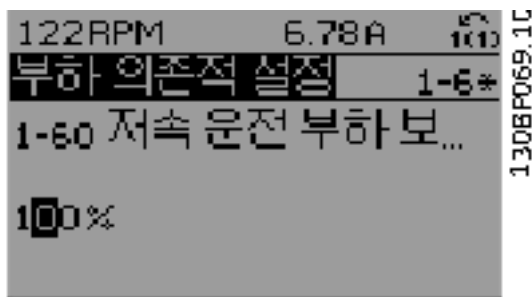
Illustration 5.14 표시 예.
