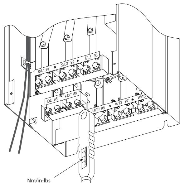
Illustration 4.29 볼트를 조일 때는 반드시 토크 측정용 렌치를 사용하십시오.
