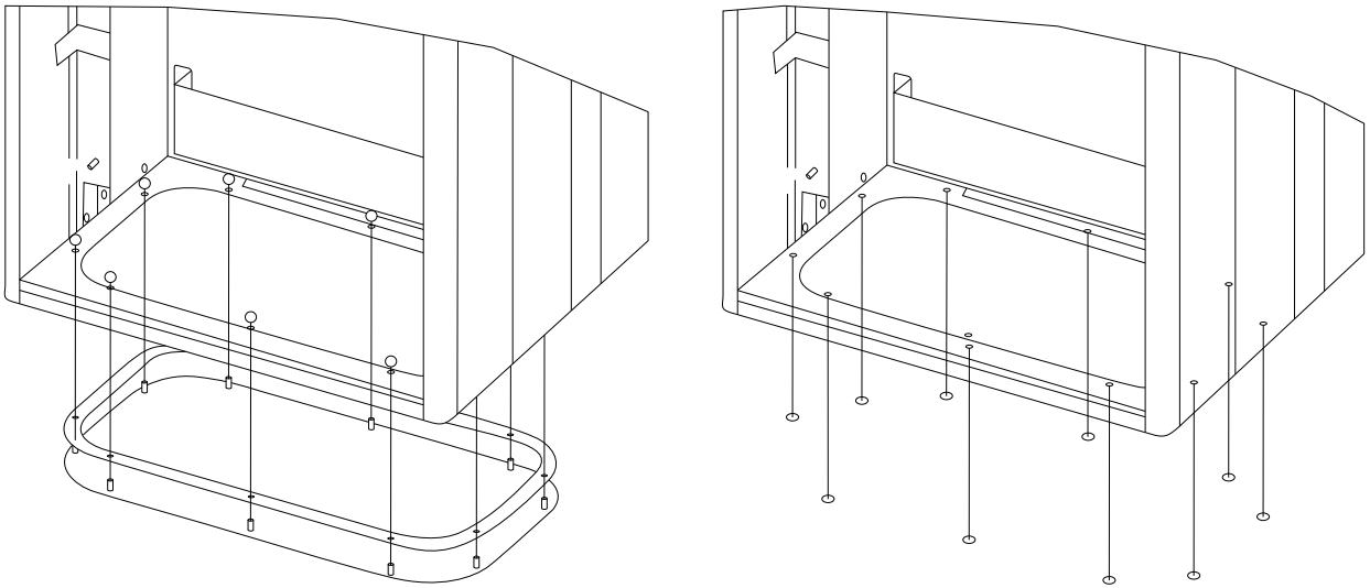
Illustration 4.21 하단 플레이트 장착, 프레임 용량 E9
