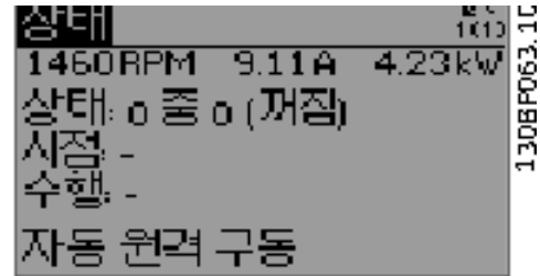
Illustration 5.4 상태 표시 III - 운전 변수
