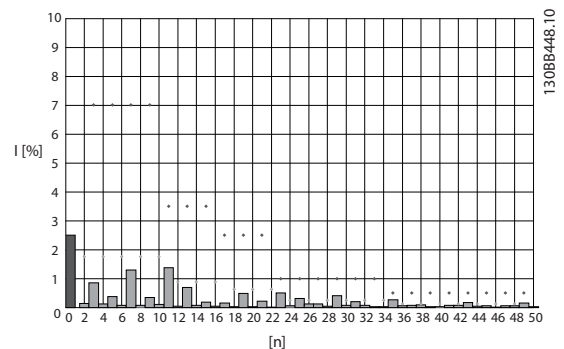
Illustration 3.2 인버터 주전원 단자에서의 일반 고조파 주파수 스펙트럼 및 THD 값
