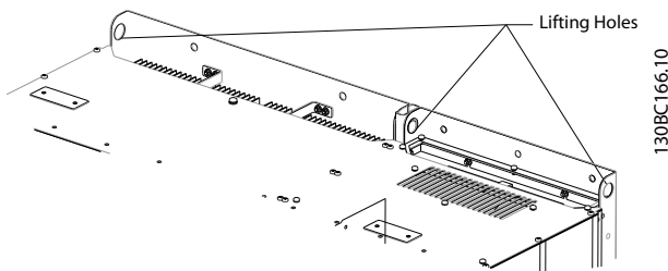
Illustration 4.2 들어 올리는 방법(권장), 프레임 용량 D13
