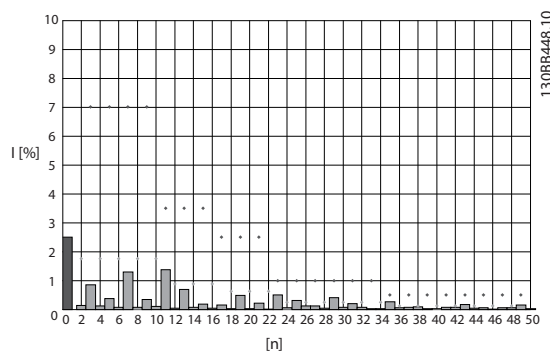
Illustration 3.2 变频器主电源端子处的通常谐波频谱和 THD 值 n = 谐波次数 ◇.....IEEE519 ( I_{sc}/I_L > 20 ) 规定的单个谐波极限
