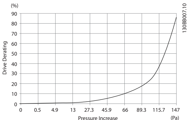
Illustration 4.14 D 机架的降容与 压力变化的关系 变频器气流 : 450 cfm (765 m 3 /h)
