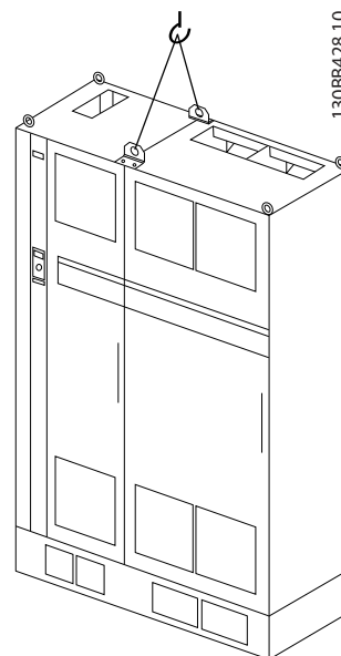
Illustration 4.5 机架规格 F18 的建议起吊方法 - 变频器单元。
