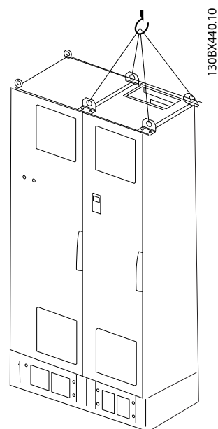
Illustration 4.4 机架规格 F18 的建议起吊方法 - 滤波器单元。
