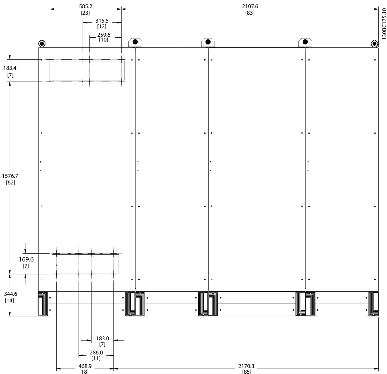
Illustration 4.9 机架规格 F18 (后视图)
