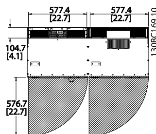
Illustration 4.11 IP21/IP54 型机箱、E9 规格机架的前方空间。
