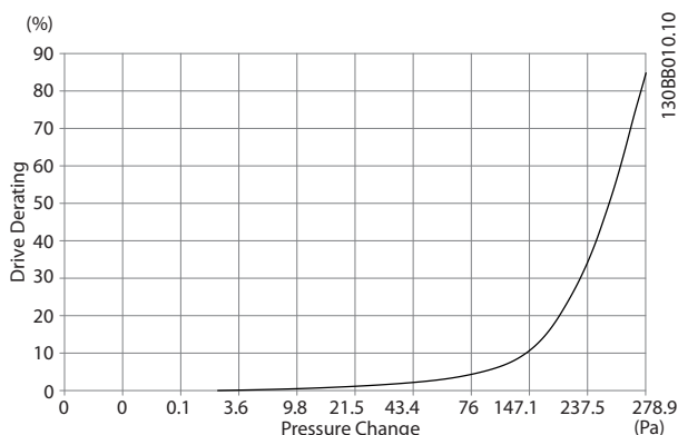
Illustration 4.15 E 机架的降容与 压力变化 (小风扇), P315 变频器气流 : 650 cfm (1105 m 3 /h)
