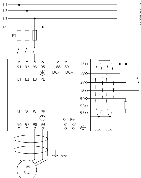
Illustration 4.1 此图显示了基本安装，其中包括主电源、电动机、启动/停止键以及用于调整速度的电位计。
