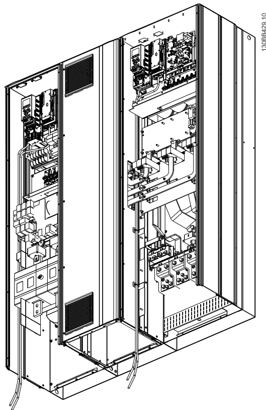
Illustration 4.33 E9 的控制卡接线路径
