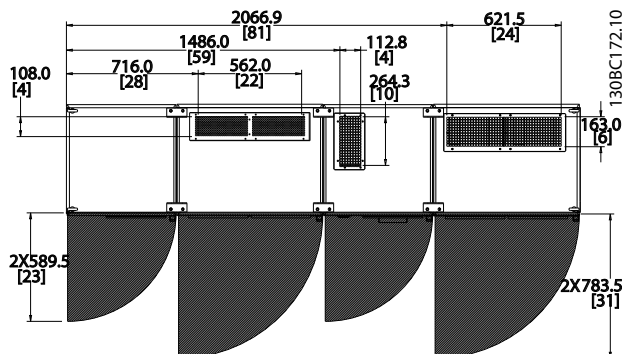
Illustration 4.12 IP21/IP54 型机箱、F18 规格机架的前方空间。
