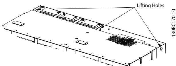
Illustration 4.3 机架规格 E9 的建议起吊方法
