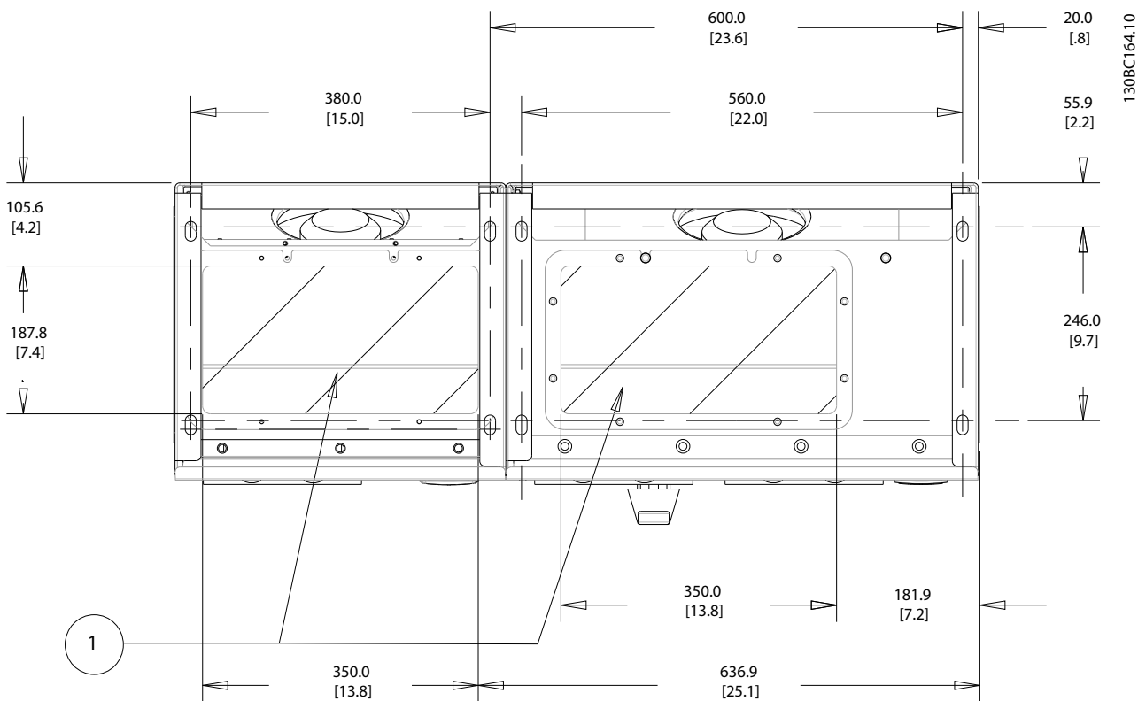
Illustration 4.19 机架规格 D13
