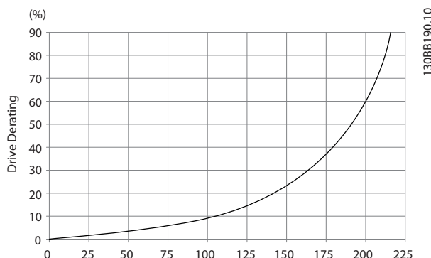
Illustration 4.17 F 机架的降容与 降容 变频器气流 : 580 cfm (985 m 3 /h)
