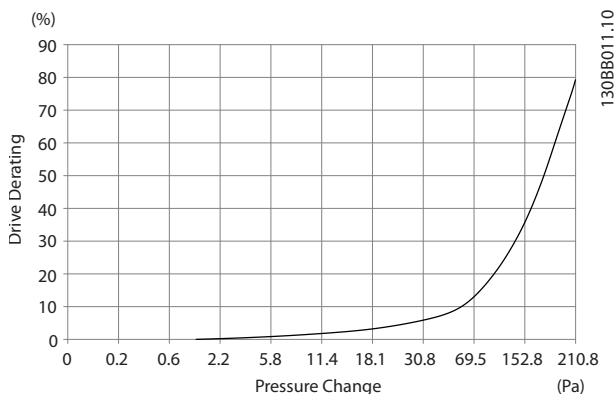
Illustration 4.16 E 机架的降容与 压力变化 (大风扇) P355-P450 变频器气流 : 850 cfm (1445 m 3 /h)
