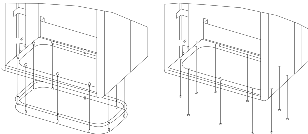
Illustration 4.21 底板安装，机架规格 E9
