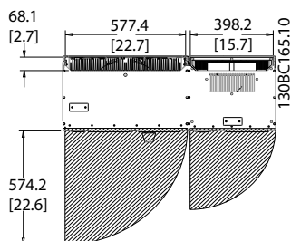
Illustration 4.10 IP21/IP54 型机箱、D13 规格机架的前方空间。
