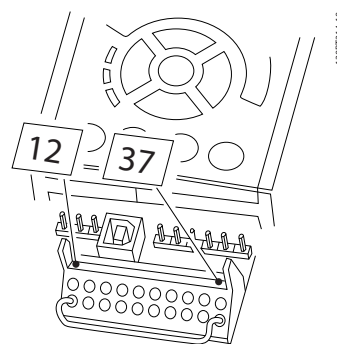
Illustration 2.1 端子 37 和 24 V 直流之间的桥接跳线
