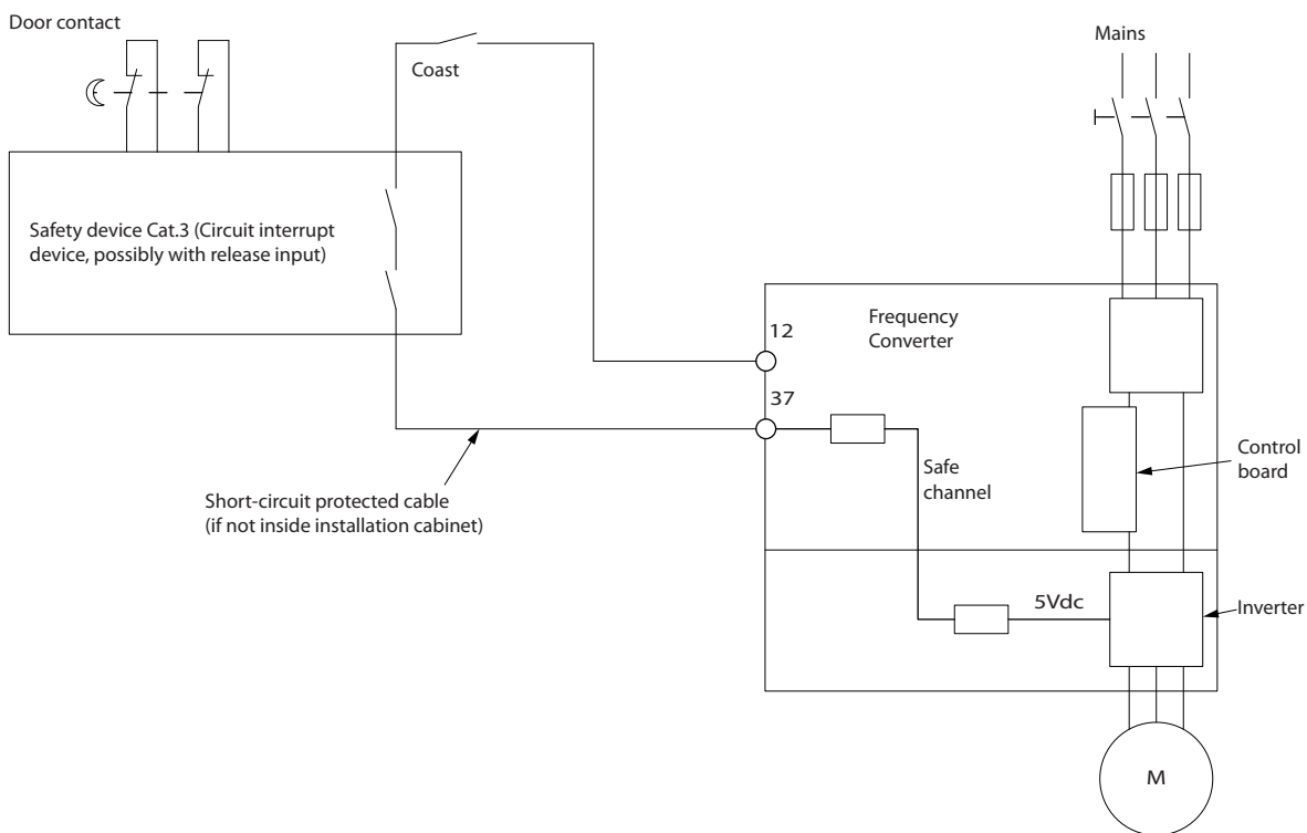
Illustration 2.2 符合停止类别 0 (EN 60204-1) 及安全类别 3 (EN 954-1) 要求的安装要点图示。
