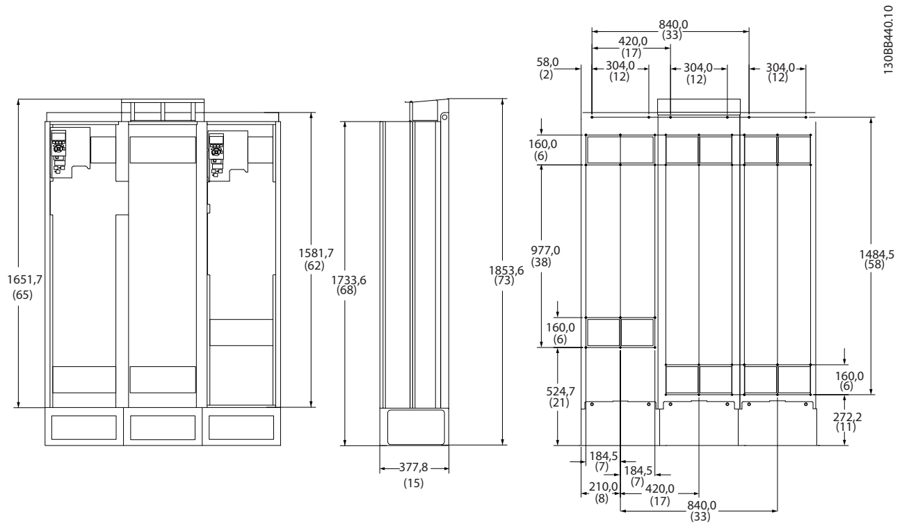
Illustration 4.6 机架规格 D13
