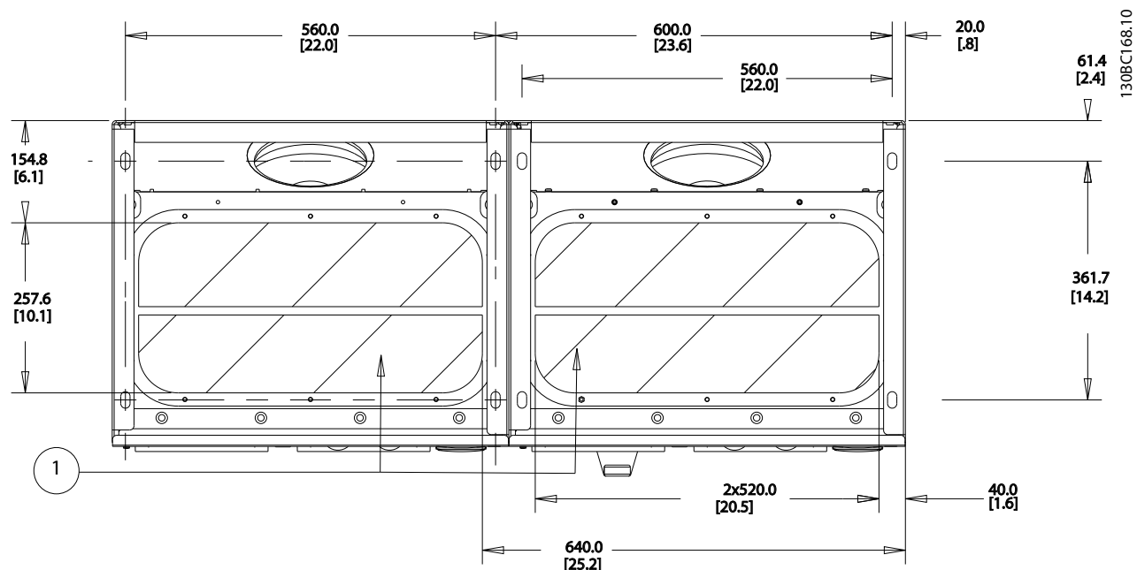
Illustration 4.20 机架规格 E9
