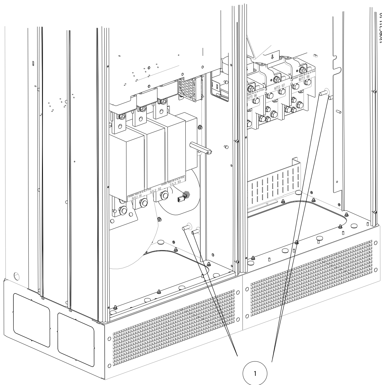
Illustration 4.28 接地端子位置
