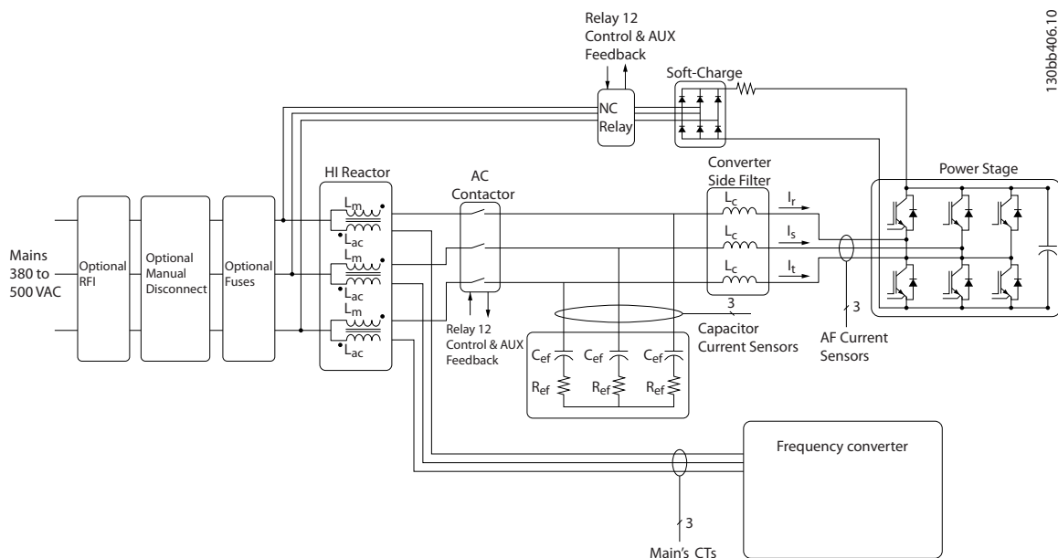
Illustration 3.1 低谐波变频器的基本布局
