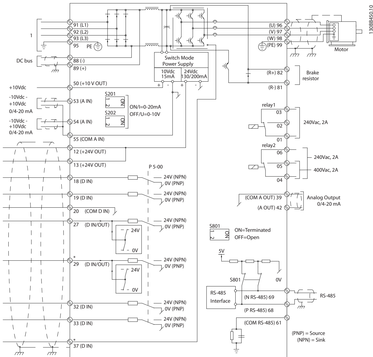
Illustration 4.39 图中显示了不带选件时的所有电气端子。
