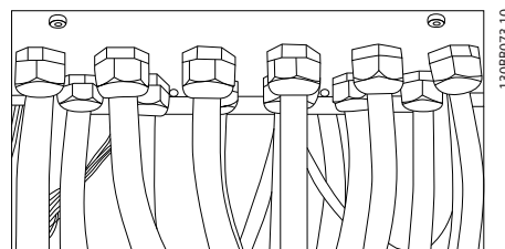
Illustration 4.18 正确安装密封板的示例。
