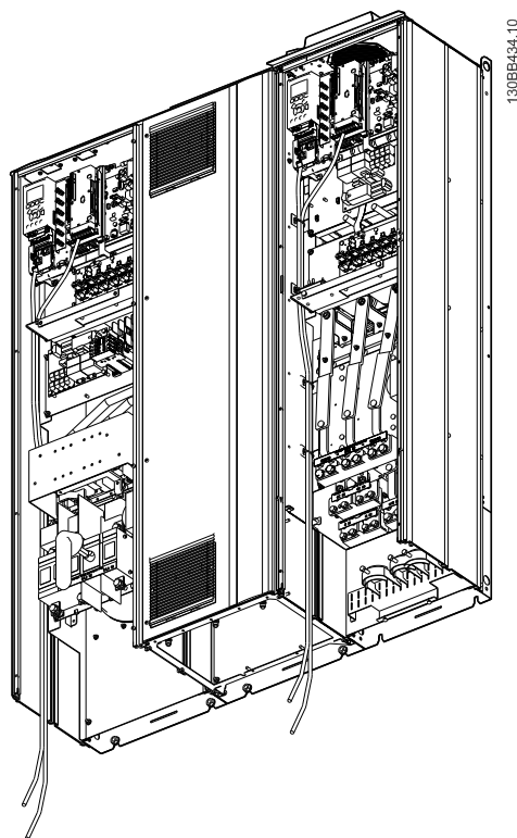
Illustration 4.32 D13 的控制卡接线路径
