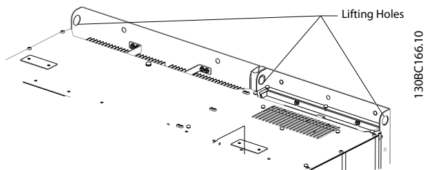
Illustration 4.2 机架规格 D13 的建议起吊方法
