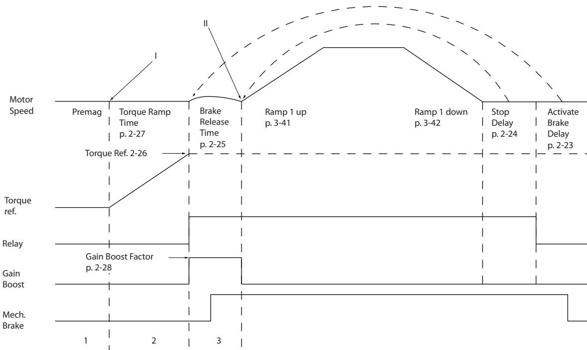
Illustration 6.9 起重机械制动控制的抱闸释放过程
