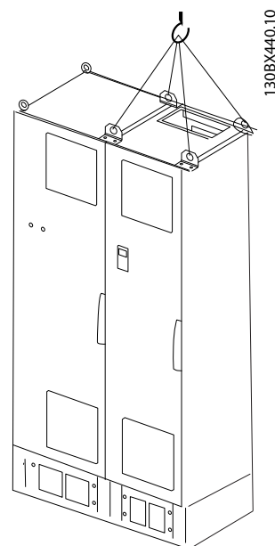
Illustration 4.4 Método de içamento recomendado, chassis de tamanho F18 - seção do filtro.
