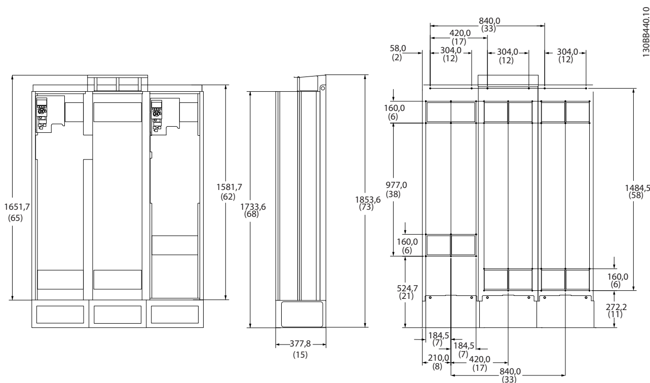
Illustration 4.6 Chassi de Tamanho D13
