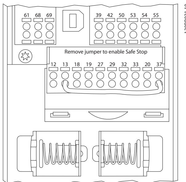
Illustration 7.2 Terminais do Cartão de Controle
