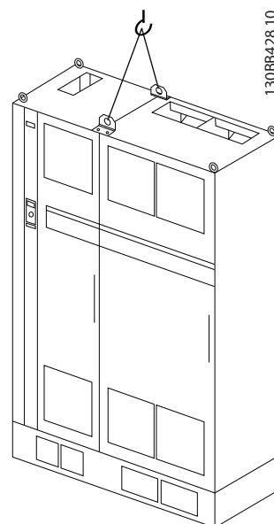
Illustration 4.5 Método de içamento recomendado, chassis de tamanho F18 - seção do drive.
