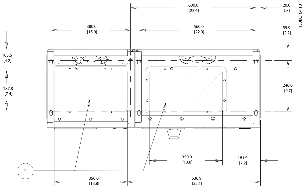
Illustration 4.19 Chassi de Tamanho D13
