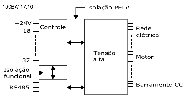
Ilustração 8.13 Isolamento PELV de Entradas Analógicas
