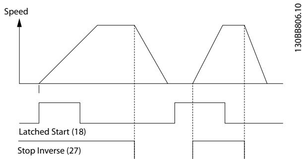
Ilustração 6.2 Partida por pulso/parada por inércia inversa
