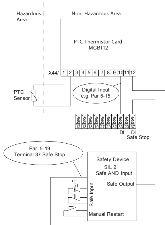
圖 3.3 結合安全轉矩關閉應用和 MCB 112 應用
