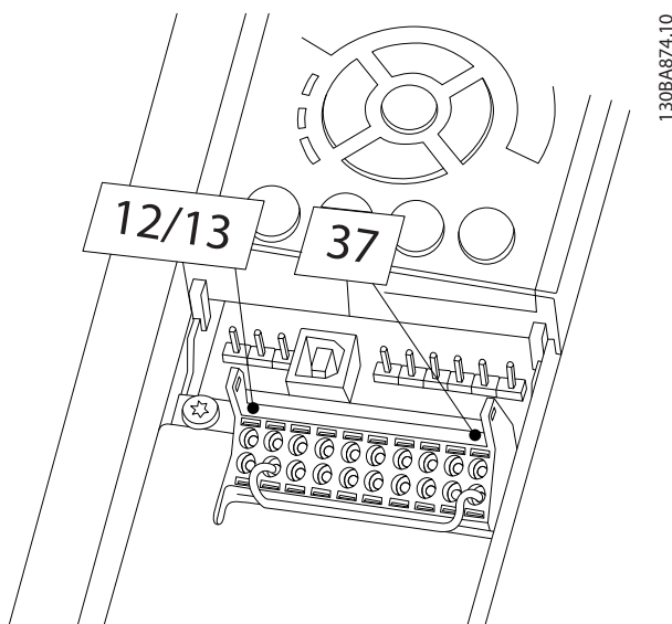
Ilustrația 3.1 Conductor de șuntare între borna 12/13 (24 V) și 37
