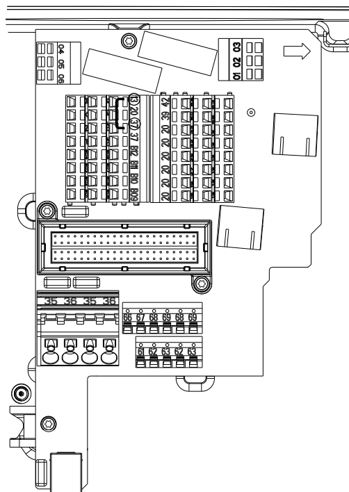
Afbeelding 3.2 Jumper tussen klem 13 (24 V) en klem 37 (FCD 302)
