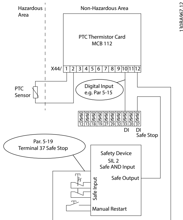
图 3.4 STO 与 MCB 112 的应用组合
