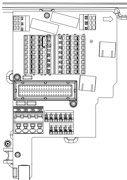
图 3.2 端子 13 (24 V) 与 37 之间的跳线 (FCD 302)
