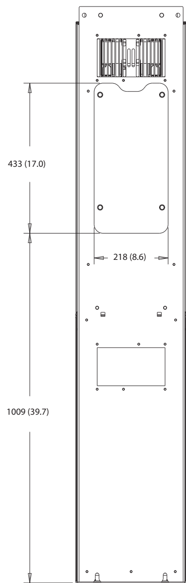
图 8.38 D6h 的散热片气流罩板尺寸
