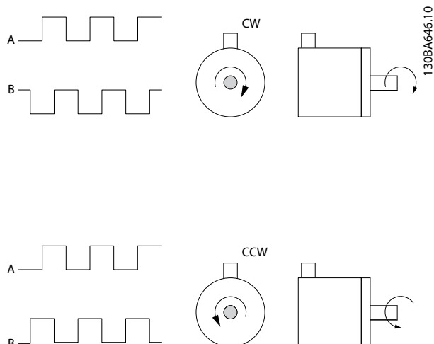
图 12.6 确定编码器方向
