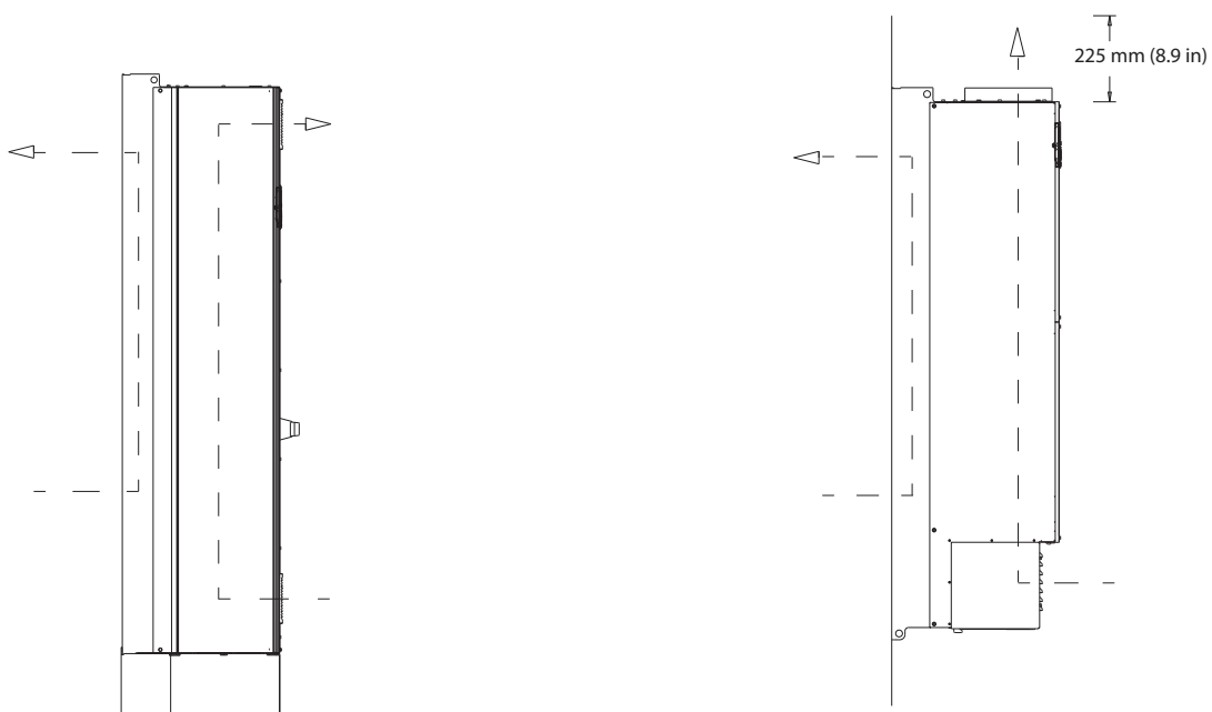
图 5.13 E1h/E2h (左) 和 E3h/E4h (右) 上通过后壁的可选气流配置
