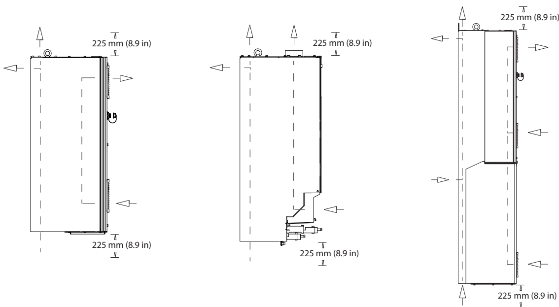
图 5.10 机箱 D1h/D2h (左)、D3h/D4h (中) 和 D5h - D8h (右) 的标准气流配置。
