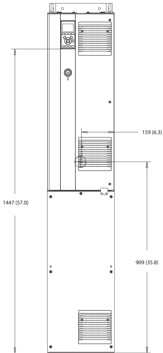
图 8.35 D6h 的正视图
