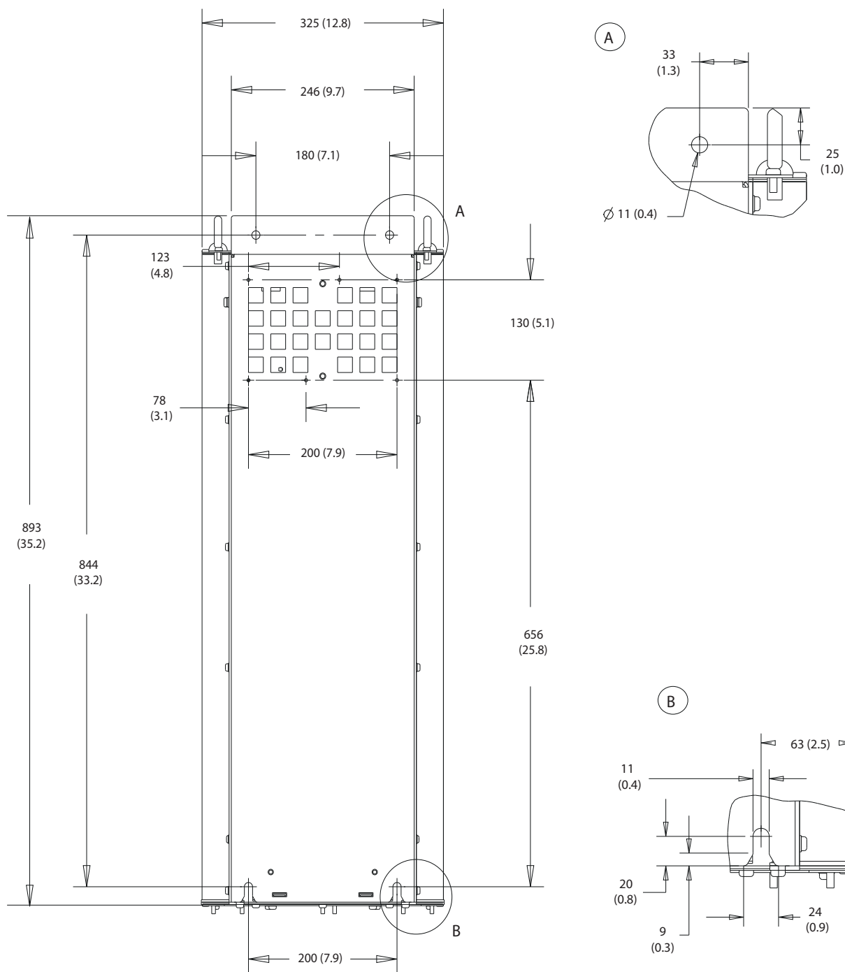
图 8.3 D1h 的后视图
