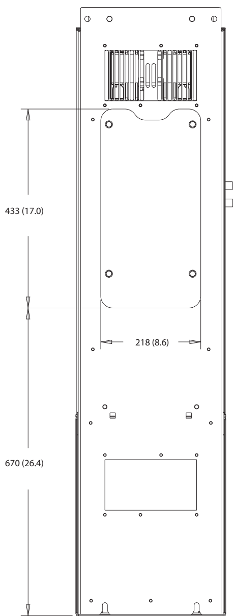
图 8.28 D5h 的散热片气流罩板尺寸
