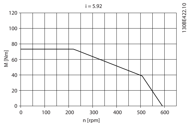
图 8.4 比率 i=5.92
