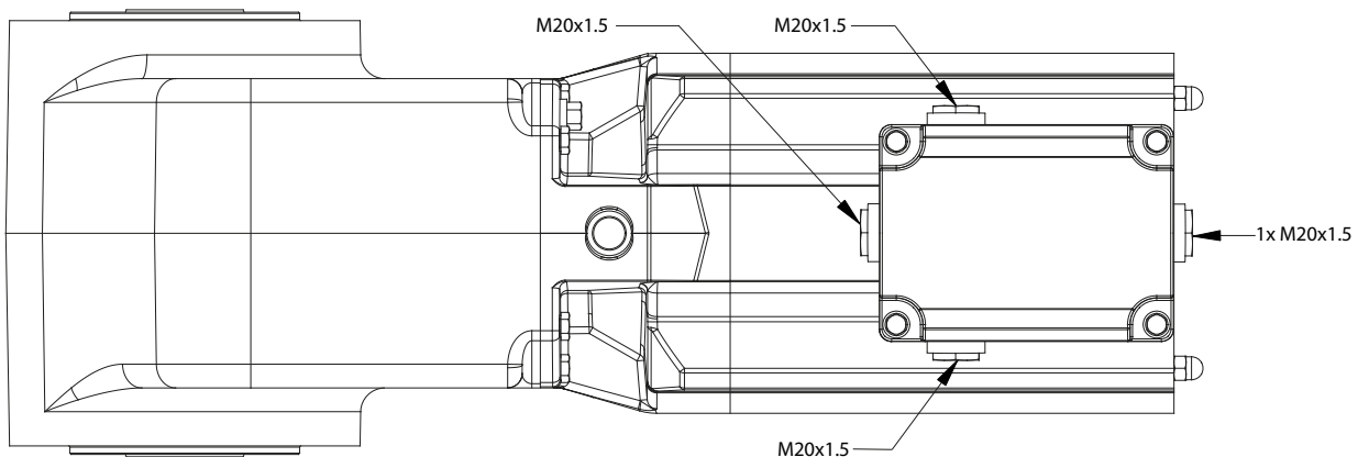
图 4.2 接线盒螺钉
