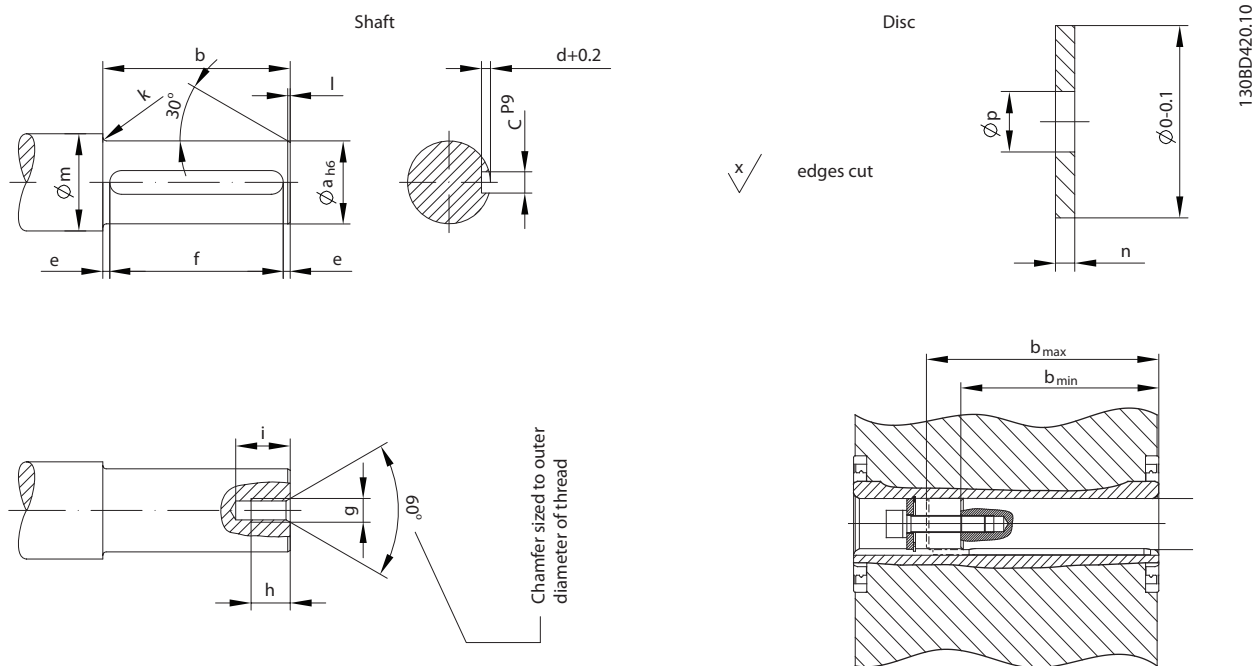
图 3.3 轴向紧固
