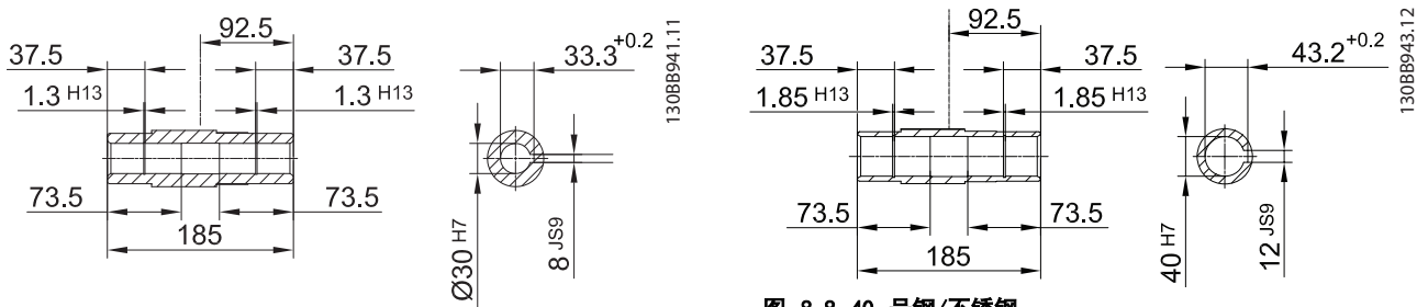
图 8.8 40 号钢/不锈钢
