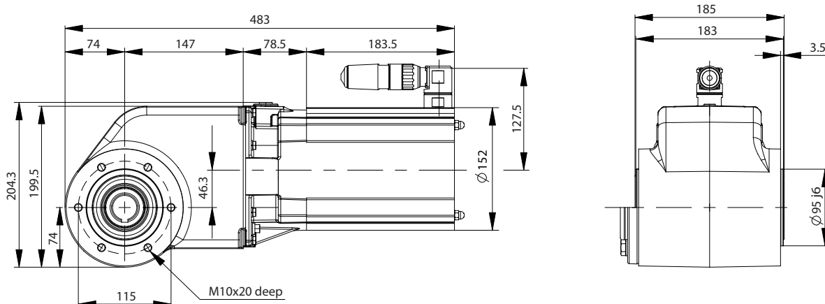
图 8.10 OneGearDrive 卫生型
