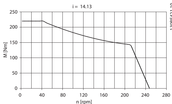
图 8.3 比率 i=14.13
