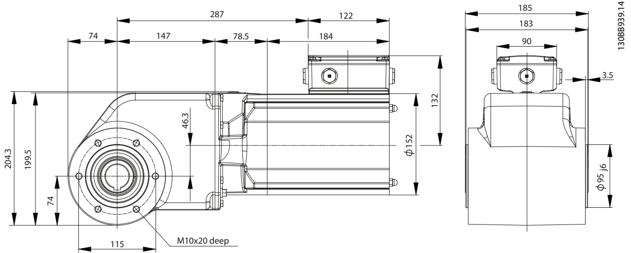
图 8.5 OneGearDrive 标准型
