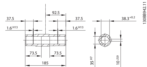
图 8.7 35 号钢/不锈钢
