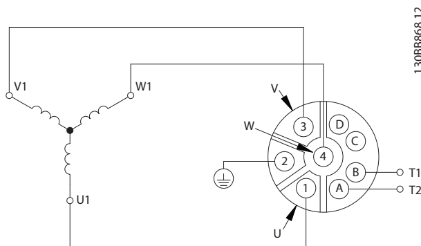
Илюстрация 4.4 Свързване на CleanConnect® OneGearDrive
