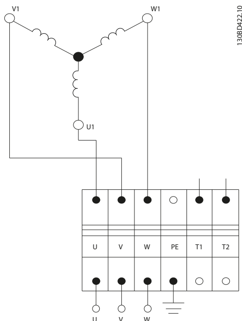
Илюстрация 4.3 Диаграма на свързване на SageClamp
