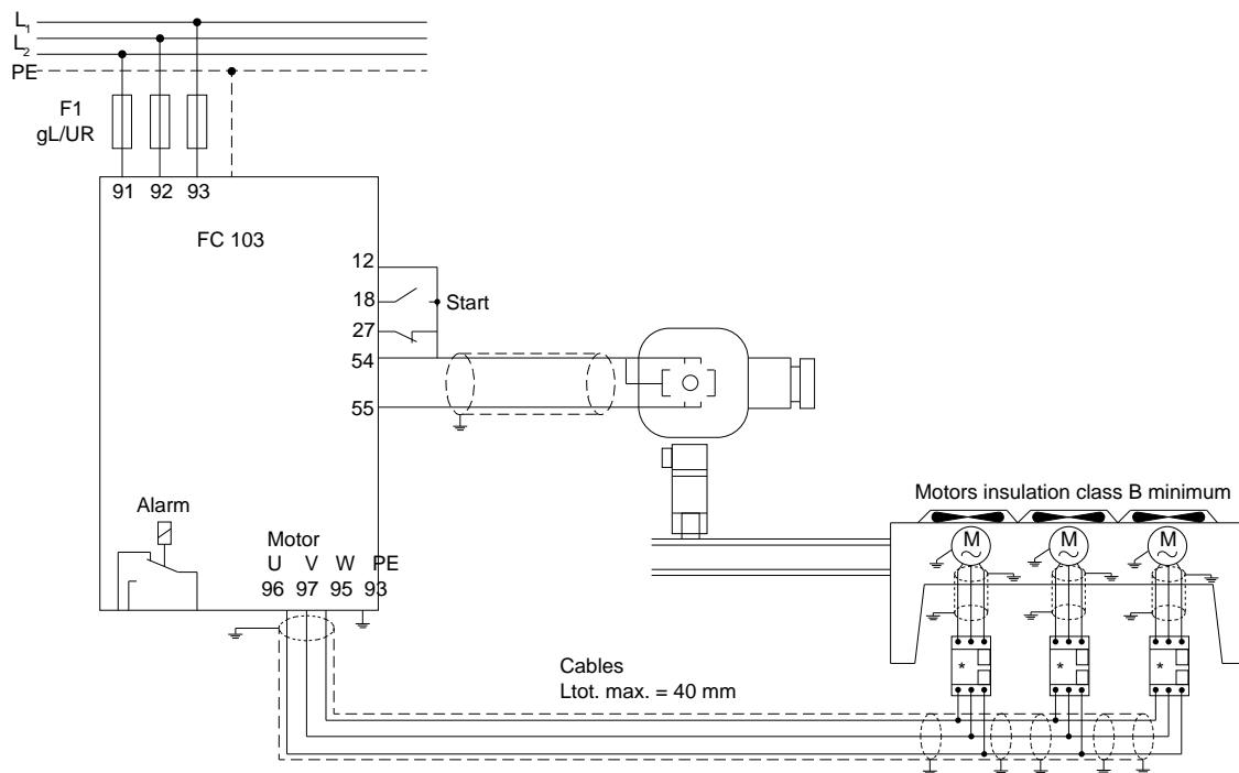
图解 65: 闭环压力控制 — 独立系统 — 单个风扇或泵/并联使用多个风扇或泵
