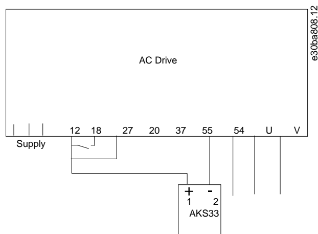
图解 67: 如何在闭环应用中连接 FC 103 和 AKS33
