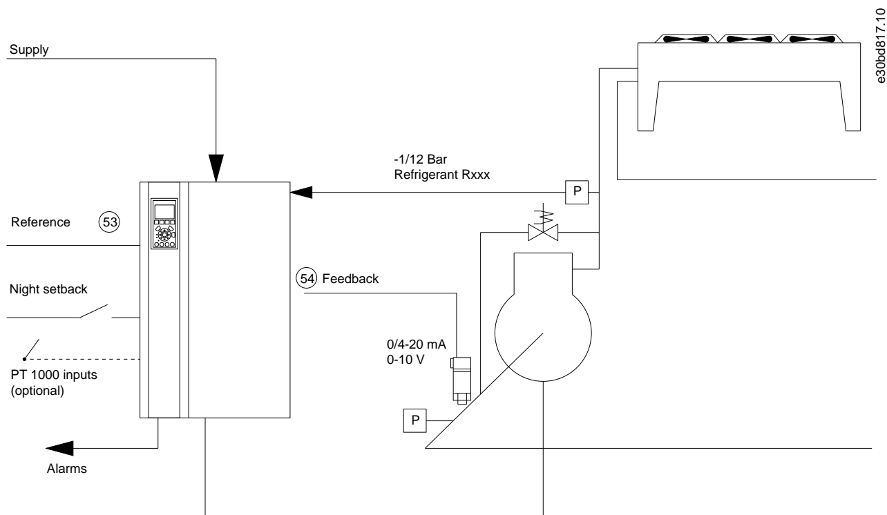
图解 63: “带内部控制的压缩机”的标准配置
