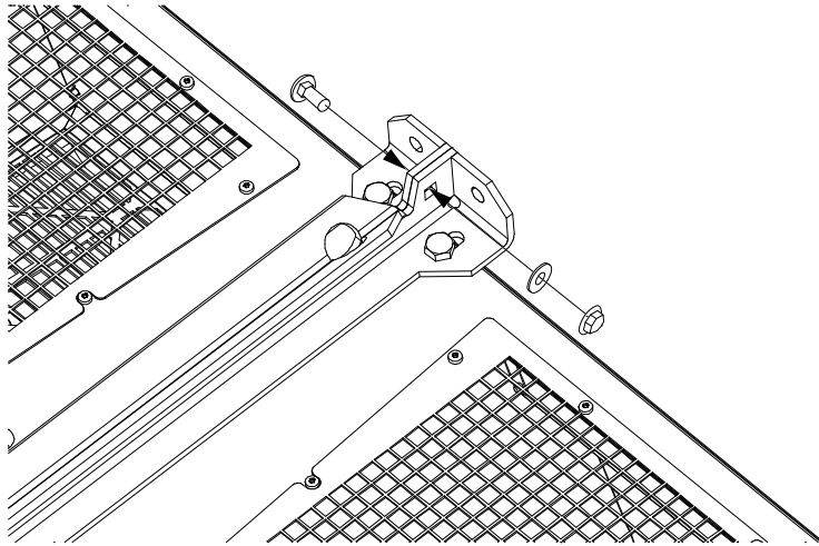
图解 15: 将机柜吊孔互连
