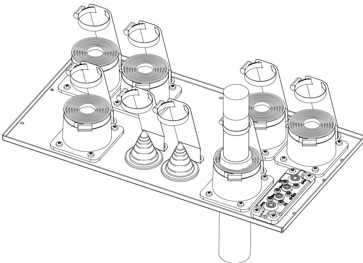
图解 17： 通过 IP54（IEC 型）电缆入口板安装电机和主电源电缆
