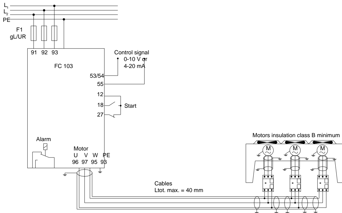
图解 64: 使用模拟参考值进行速度控制 (开环) — 单个风扇或泵/并联使用多个风扇或泵
