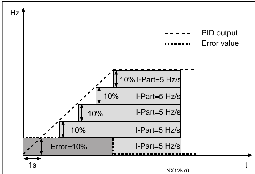
图 1-25. PID 控制器作为积分控制器的功能
