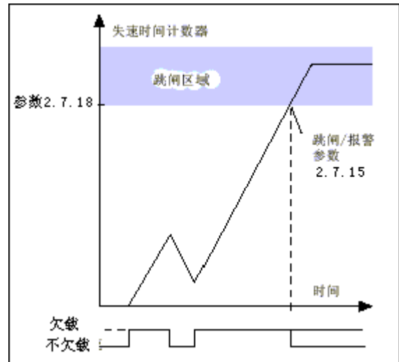
图 1-23 欠载时间计时功能
