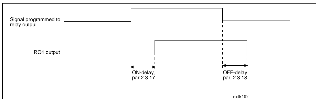
图1-9. 继电器输出1的开启和关闭延迟
