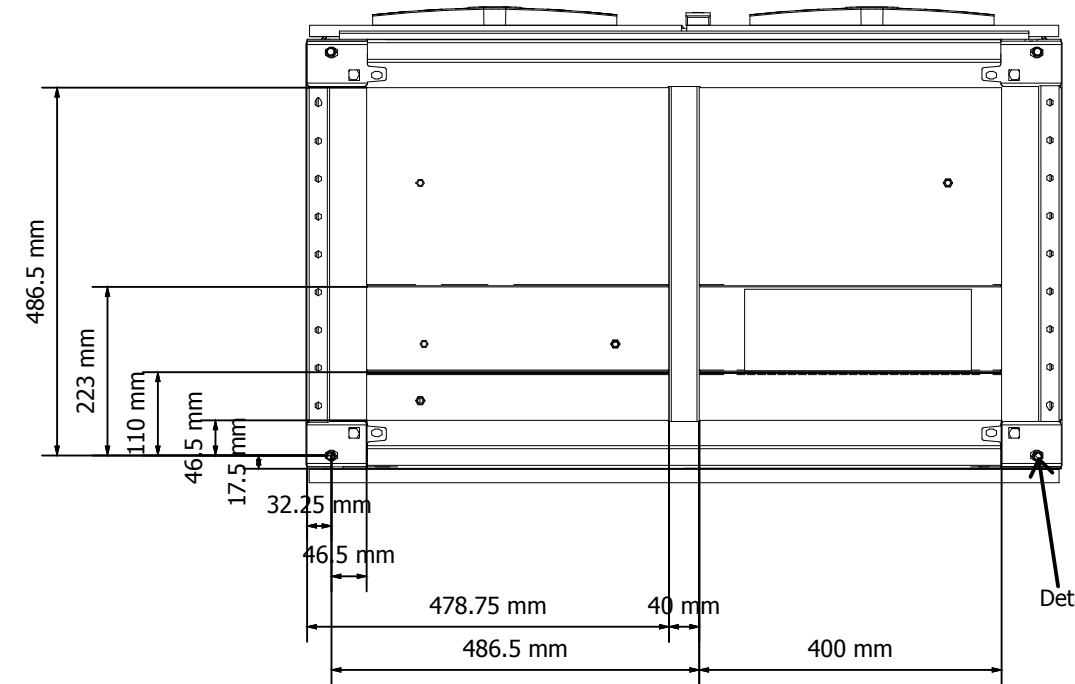
Bottom view Ansicht von unten
