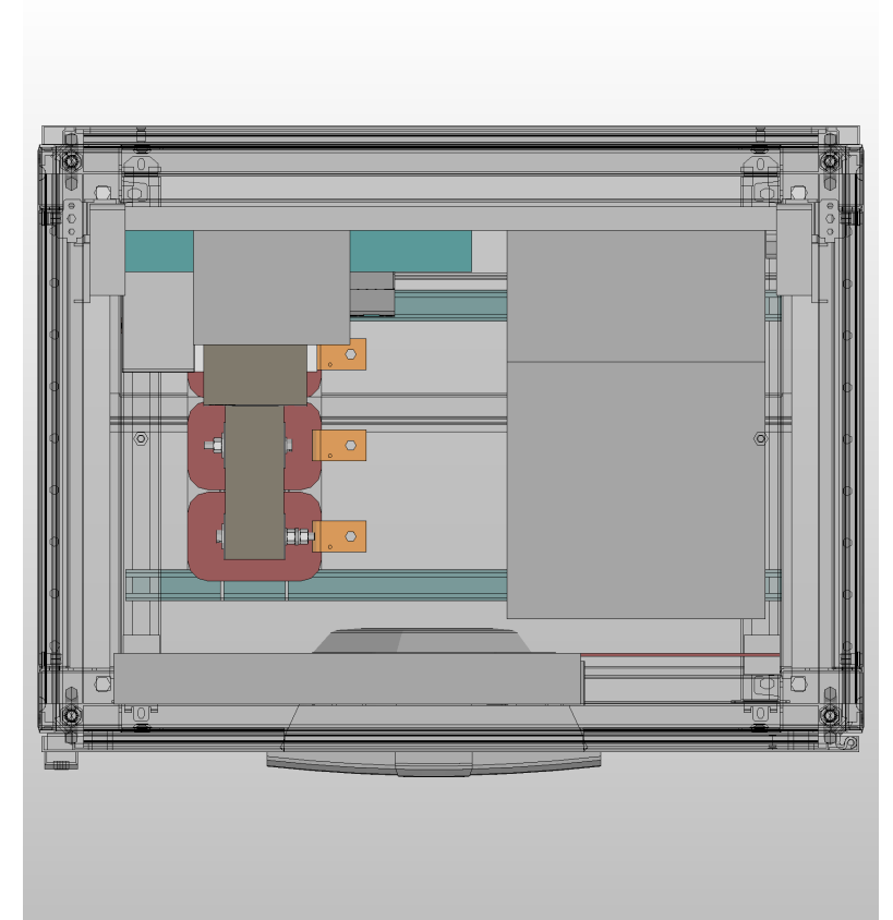
Top view Draufsicht
