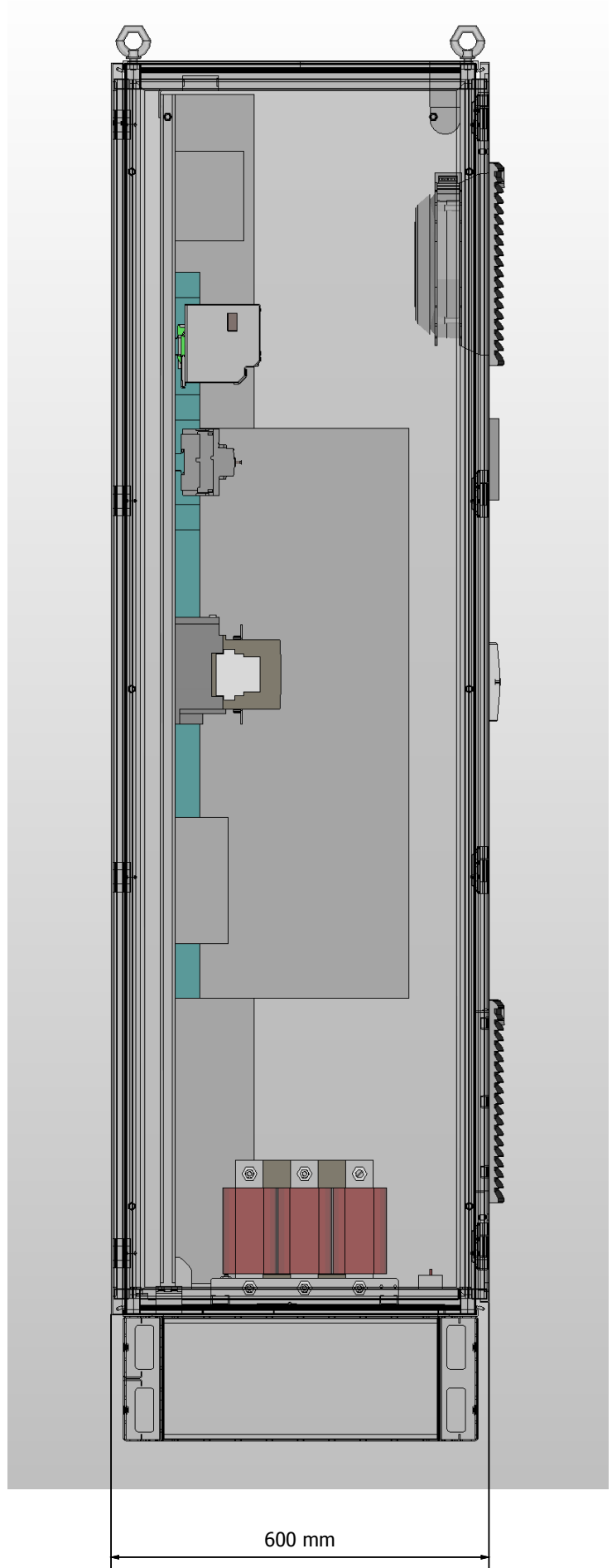
Side view Seitenansicht
