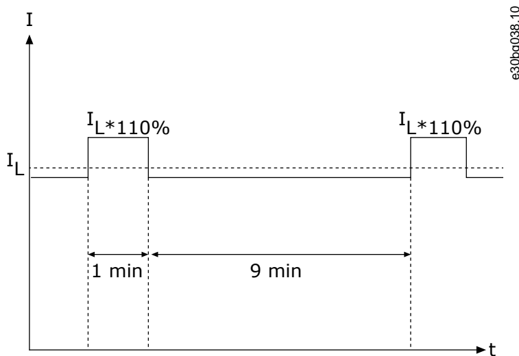
Bild 74: Låg överbelastning
