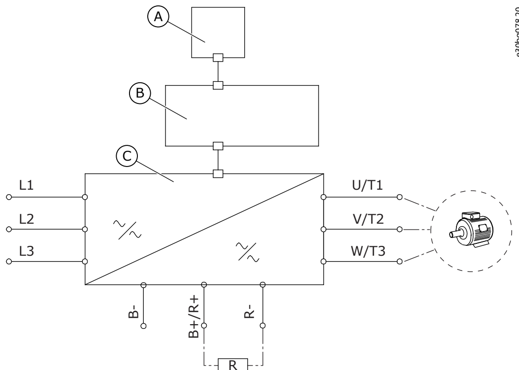
Bild 13: Kopplingsschema
