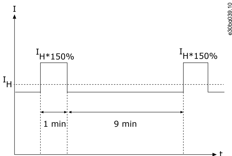
Bild 75: Hög överbelastning
