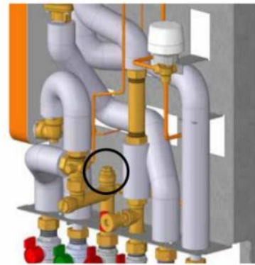
Doigt de gant
