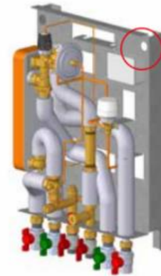
Orifice en forme de trou de serrure pour le montage.
