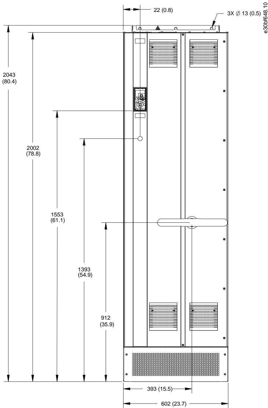
图解 53: E1h 的正视图
