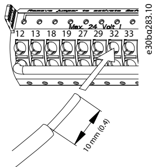
图解 36: 将实心控制电缆连接至接线盒
