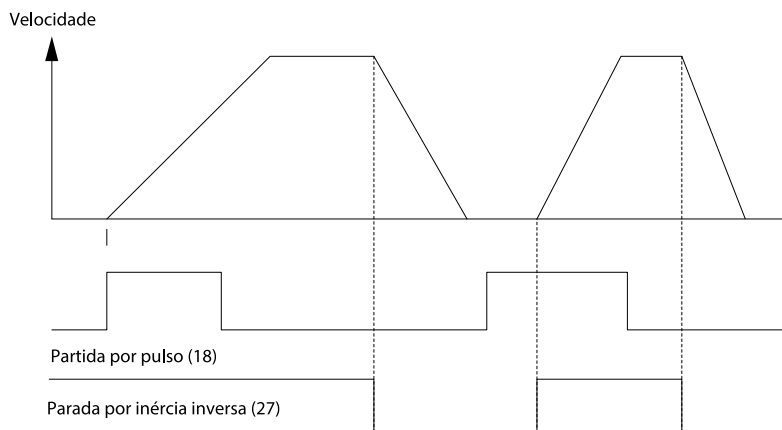
Ilustração 43: Partida por pulso/Parada por inércia inversa
