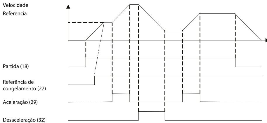
Ilustração 41: Aceleração/Desaceleração
