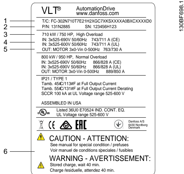
Ilustração 8: Plaqueta de identificação do produto para Gabinete E2h (exemplo)
