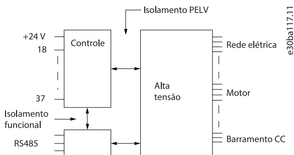
Ilustração 52: Isolamento PELV
