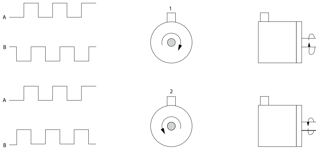
Ilustração 45: Determinação do sentido do encoder
