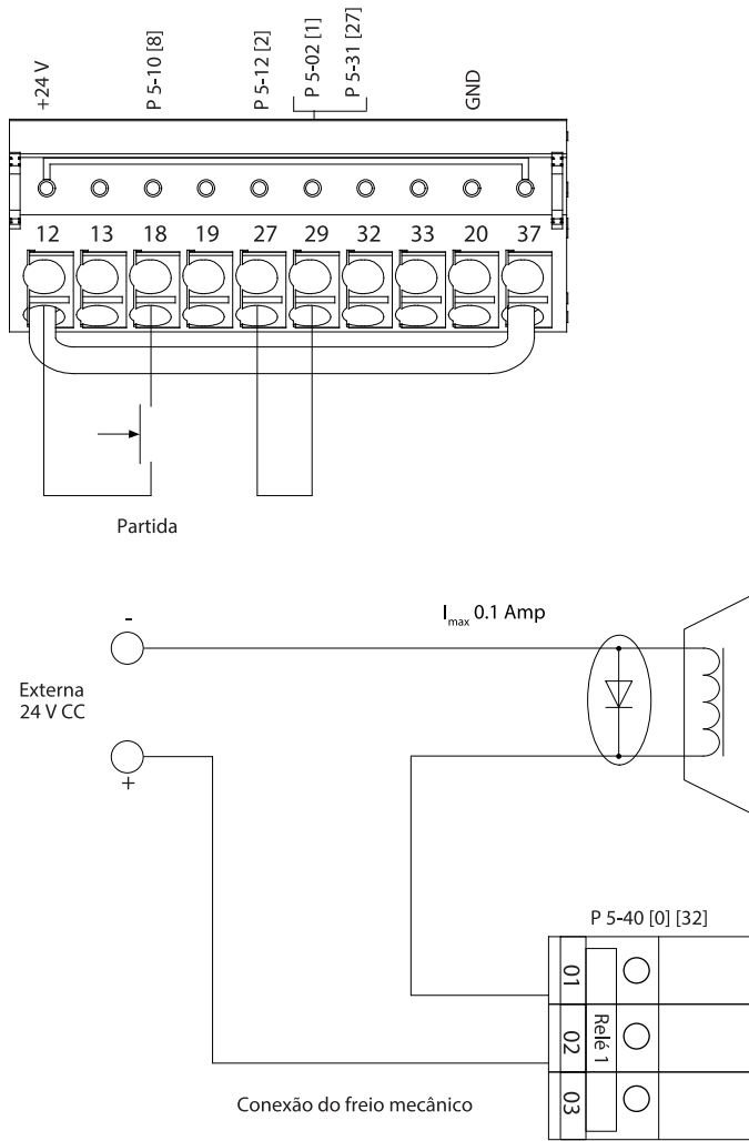
Ilustração 47: Configuração de fiação para limite de parada e torque
