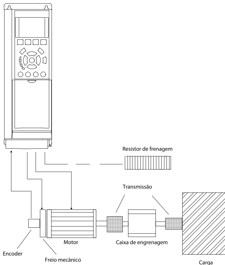
Ilustração 40: Programação básica para controle de velocidade da malha fechada
