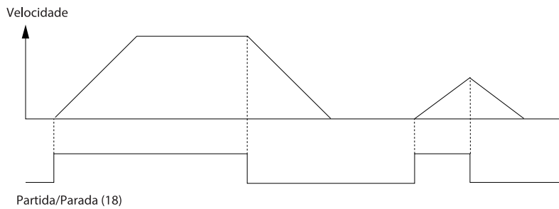
Ilustração 42: Comando de partida/parada com Safe Torque Off
