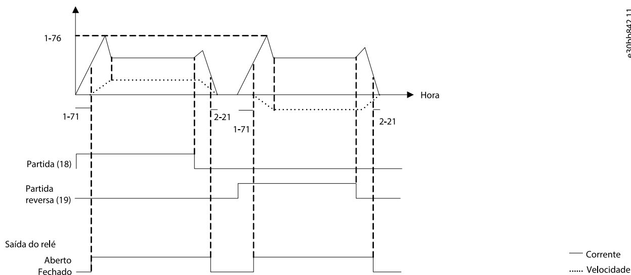
Ilustração 44: Controle do Freio Mecânico
