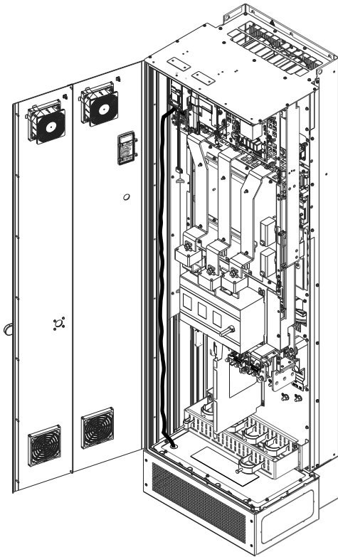
Ilustração 32: Roteamento do cabo do cartão de controle
