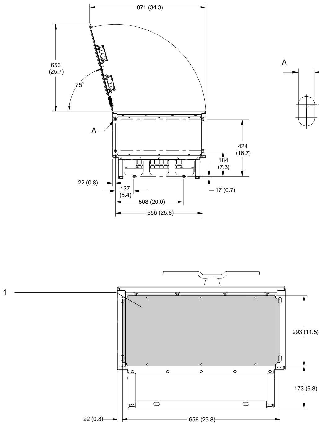
图解 60: E2h 的门间隙和电缆入口板尺寸
