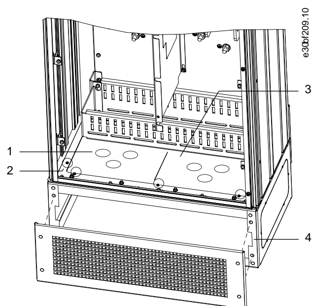
图解 13: 安装电缆入口板
