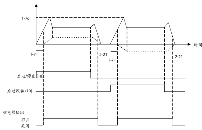
图解 44: 机械制动控制
