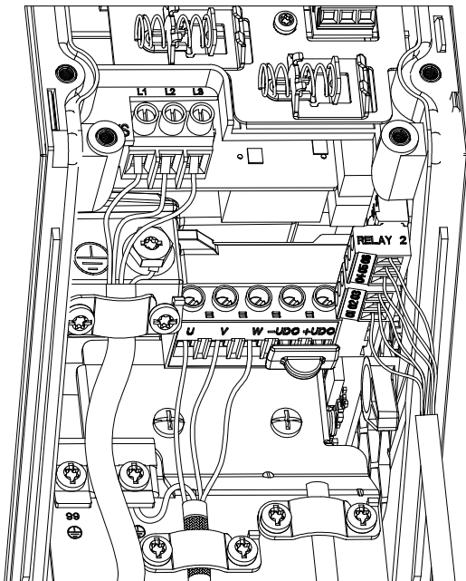
Abbildung 17: IP54 Baugrößen I2, I3, I4
