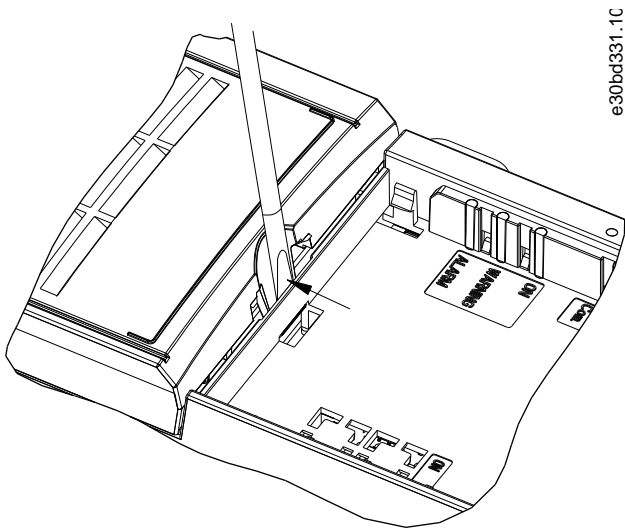
Ilustración 23: Extracción de la tapa de terminal
