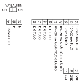
Kuva 24: Ohjausliittimet
