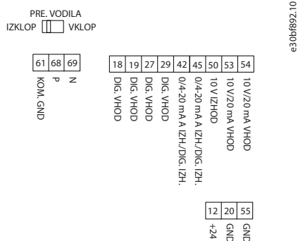
Ilustracija 24: Krmilne sponke
