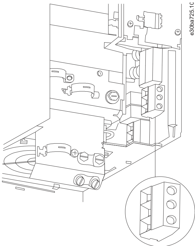
Ілюстрація 13: Корпус розміру Н10, IP20, 600 В, 11–15 кВт (15–20 кс)
