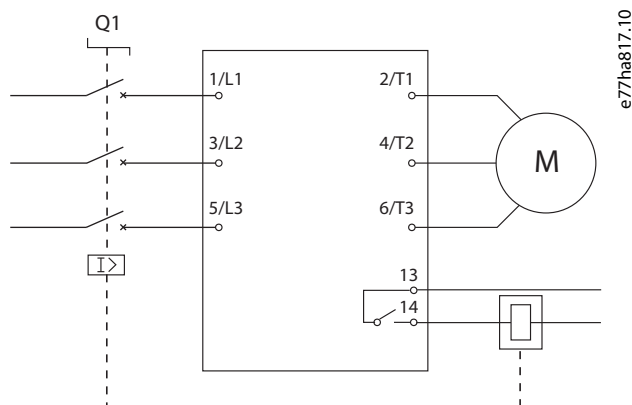
Illustration 11: Démarreur progressif installé avec un relais de déclenchement et un disjoncteur
