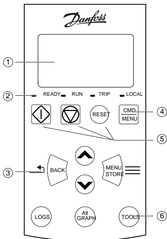
Illustration 25: LCP à distance
