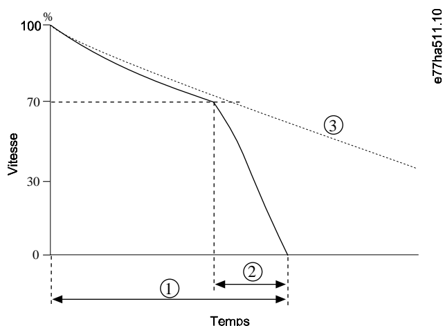
Illustration 36: Exemple de durée de freinage
