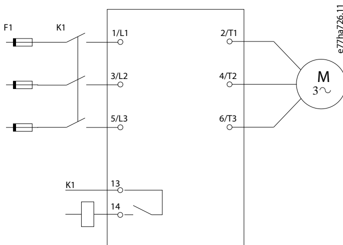
Illustration 14: Câblage d'une installation en ligne
