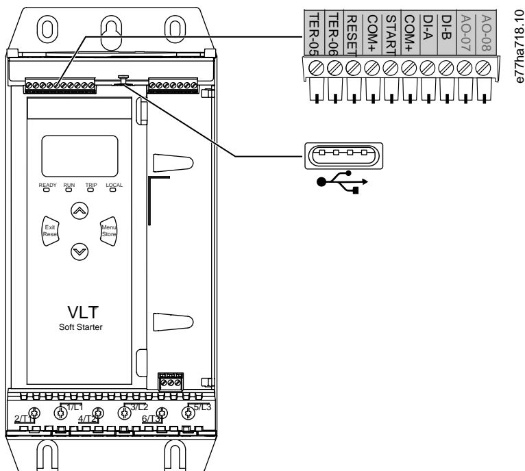
Illustration 7: Bornes d'entrée
