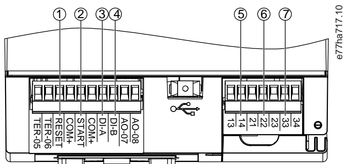
Illustration 21: Emplacement des E/S digitales
