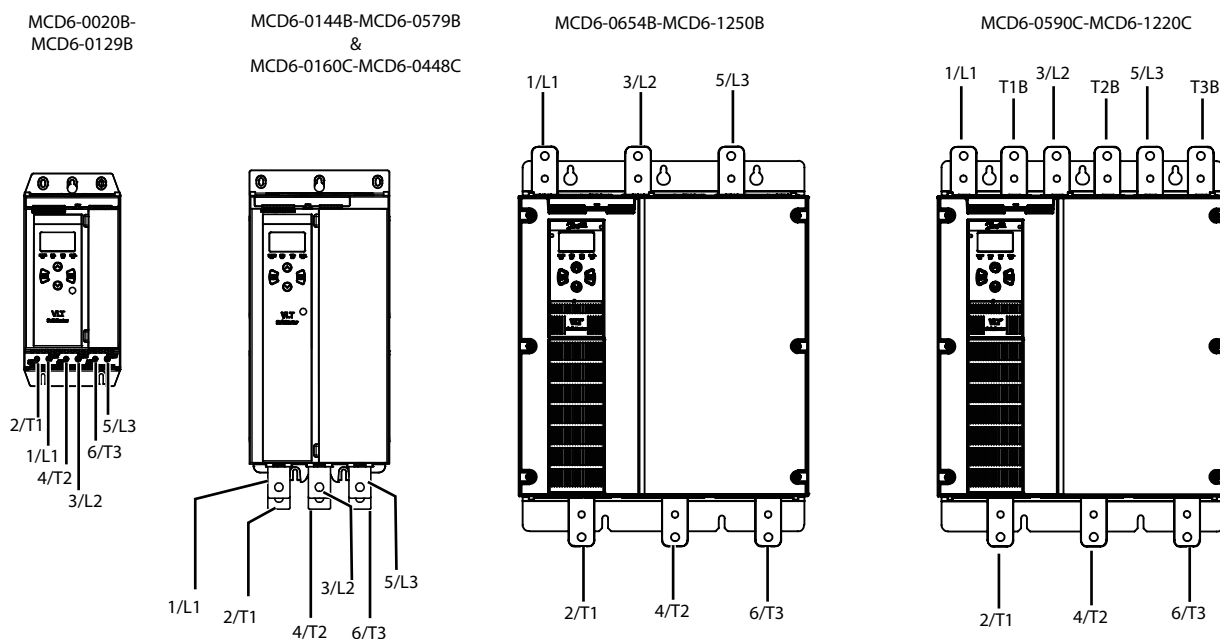
Illustration 13: Bornes d'entrée et de sortie pour les terminaisons électriques
