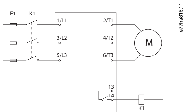
Illustration 10: Démarreur progressif installé avec contacteur principal
