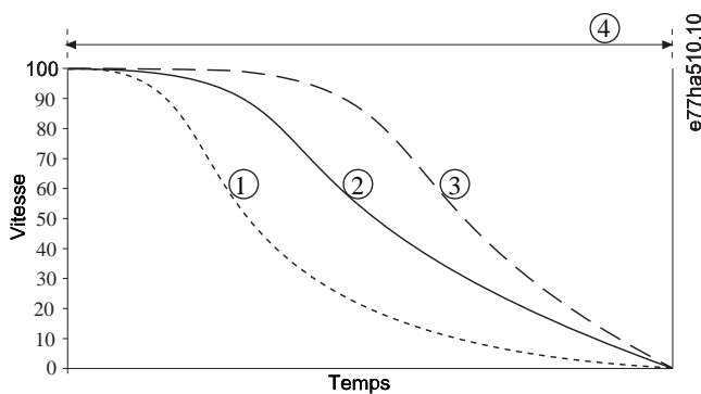
Illustration 35: Exemple d'arrêt par contrôle progressif (paramètre 2-11 Profil arrêt prog)
