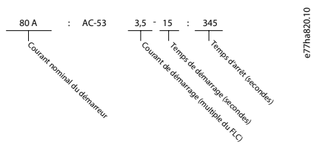
Illustration 2: Format AC53b (courant nominal avec bipasse)
