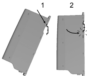
3 pav.: Tvirtinimas DIN bėgeliu, MI1–MI3
