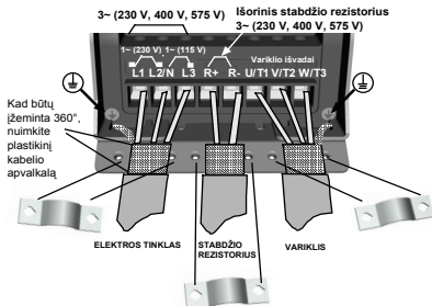
8 pav.: Vacon 20 maitinimo jungtis, MI2–MI3
