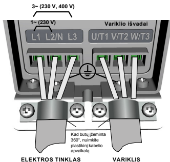
7 pav.: Vacon 20 maitinimo jungtis, MI1
