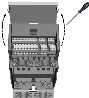
11 pav.: MI1–MI3 dangtelio atidarymas
