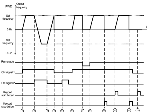
Рис. 9.6: Логика пуска/останова, выбор 3
