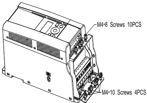
Рис. 3.14: Винты M4
