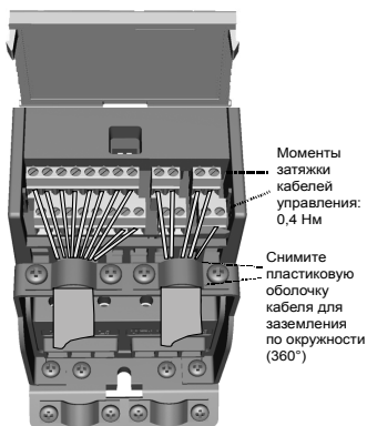
Рис. 3.11: Установите кабели управления. MI1 - MI3. См. раздел 6.2
