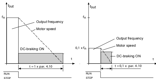
Рис. 9.8: Время торможения постоянным током в режиме останова выбегом
