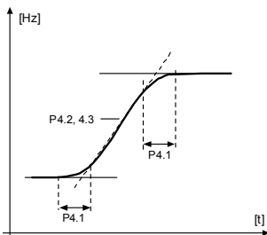
Рис. 9.7: S-образное ускорение/замедление
