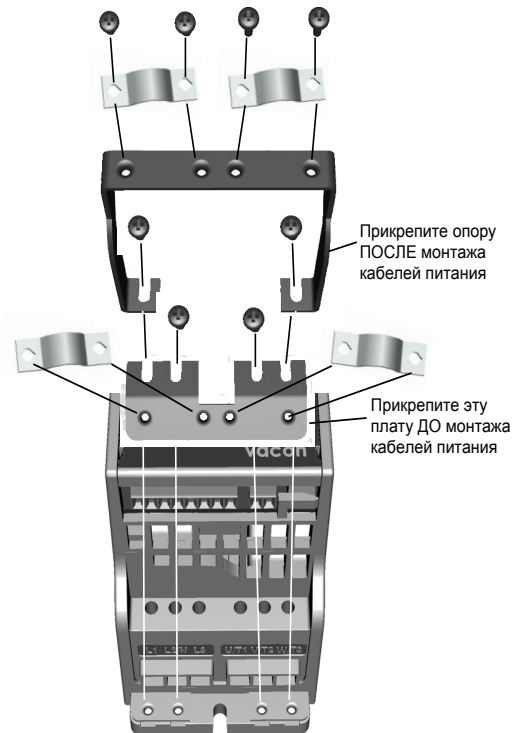
Рис. 3.9: Монтаж платы защитного заземления (PE) и крепления кабелей пользовательского интерфейса (API), M11 - M13
