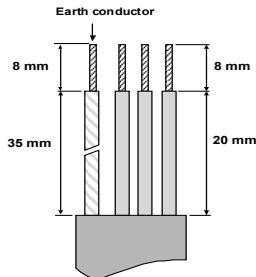
Рис. 3.15: Зачистка кабелей
