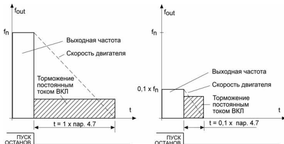
Рисунок 9.5: Время торможения постоянным током в режиме останова с выбегом
