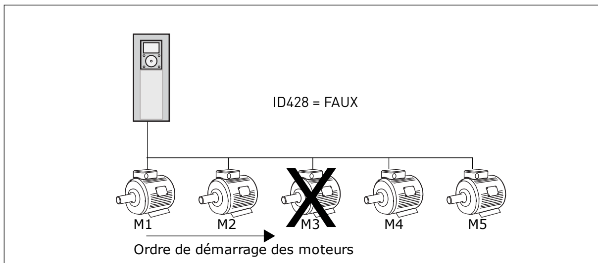
Fig. 81: Logique d'interverrouillage 2
