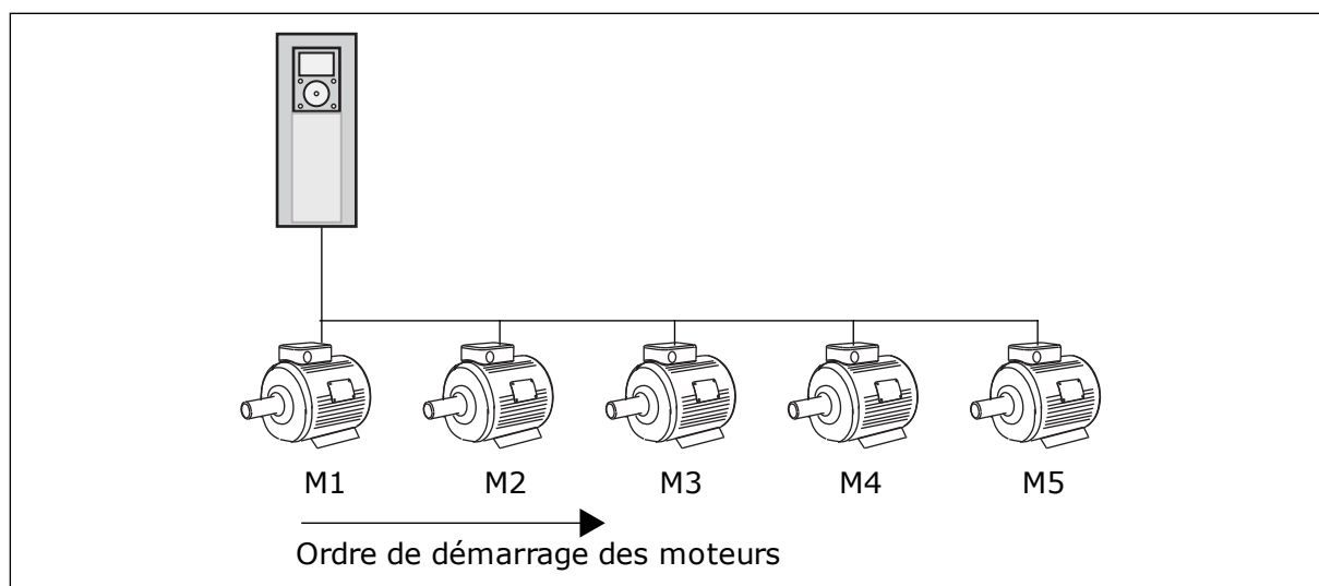
Fig. 80: Logique d'interverrouillage 1
