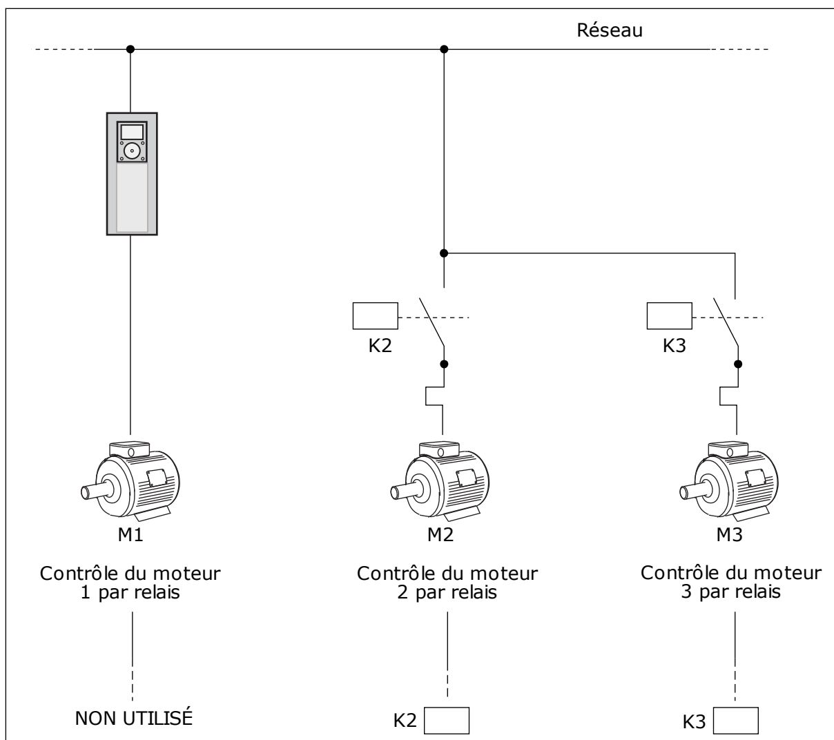
Fig. 83: Sélection 0
