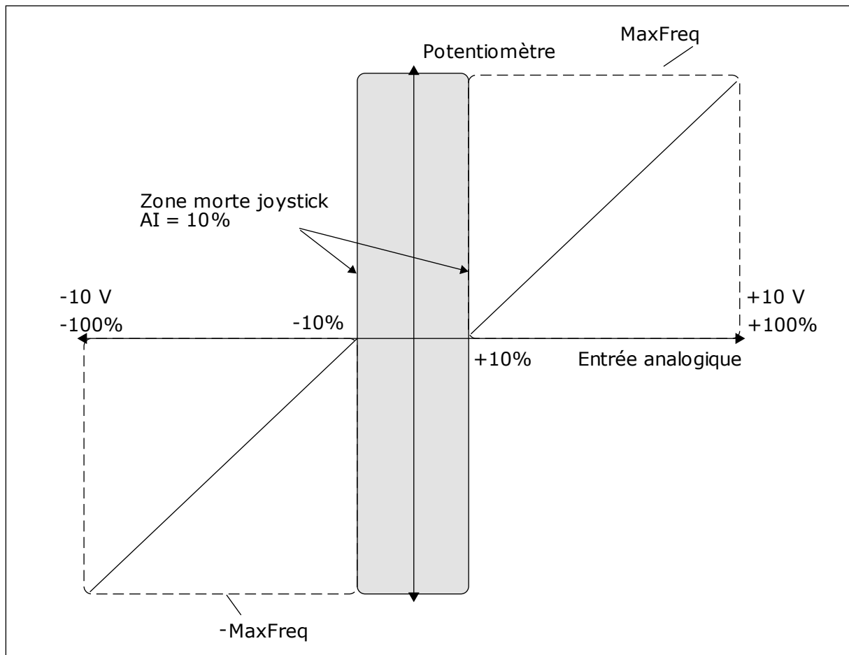
Fig. 38: Fonction Joystick
