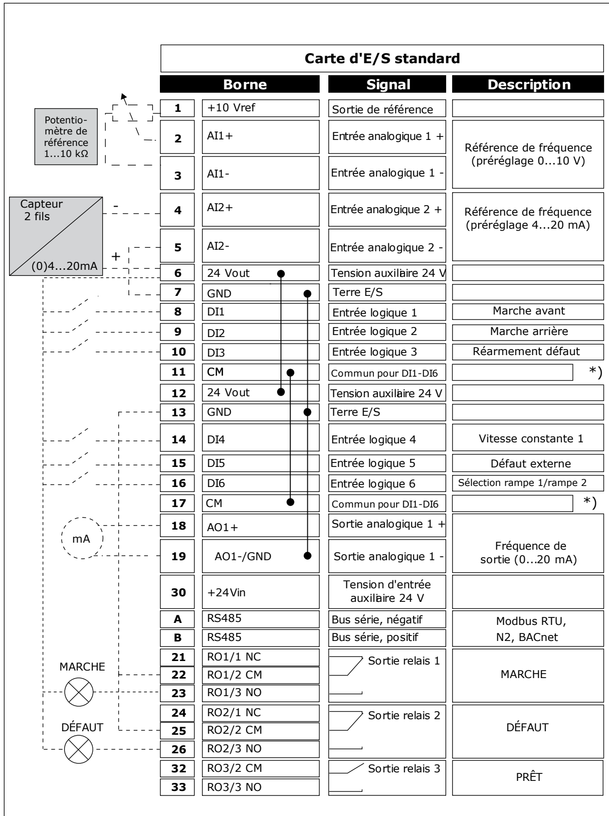
Fig. 12: Raccordements de commande préréglés de l'applicatif Multi-configuration
