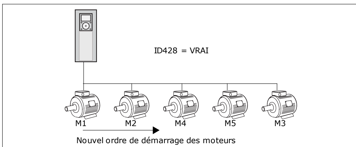
Fig. 82: Logique d'interverrouillage 3
