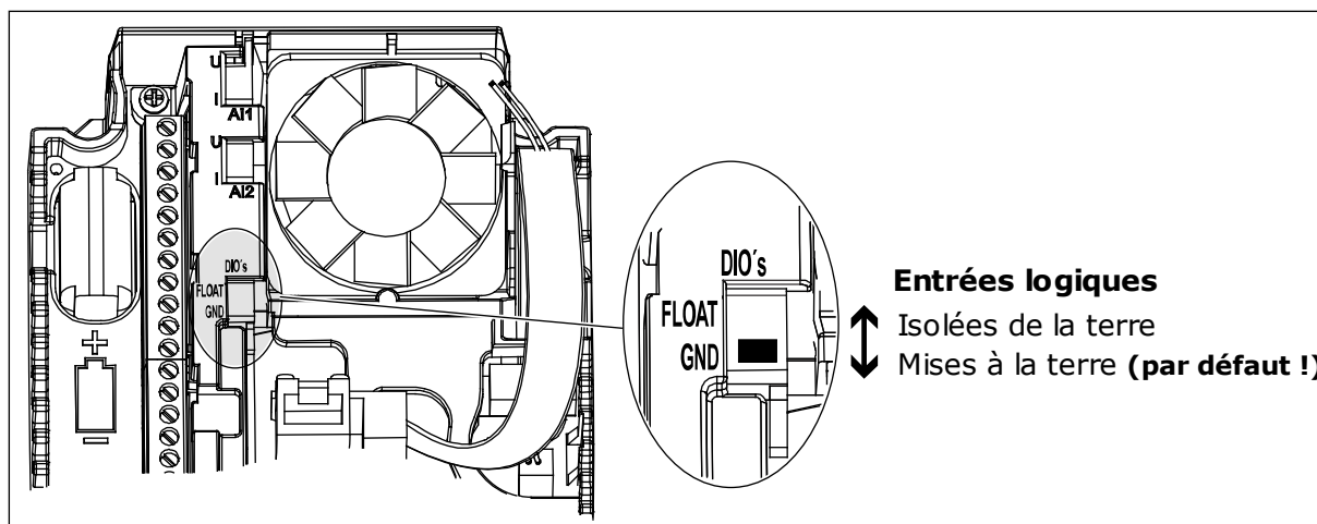
Fig. 9: Interrupteur DIP
