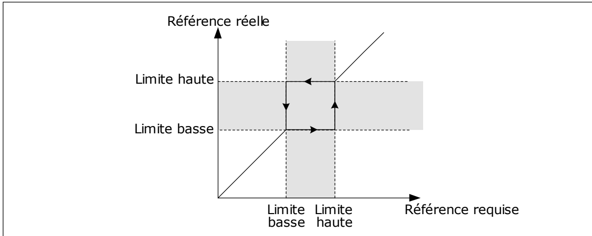
Fig. 53: Fréquences interdites
