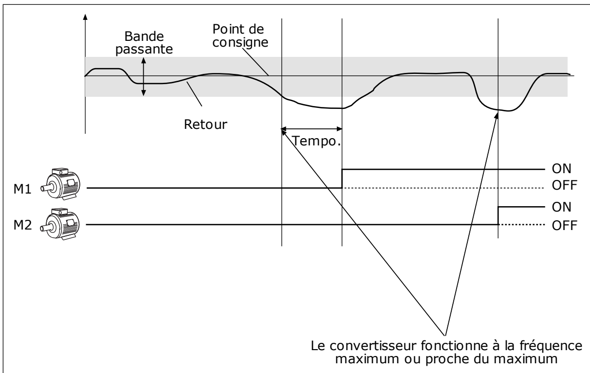
Fig. 79: Fonction Multi-pompe
