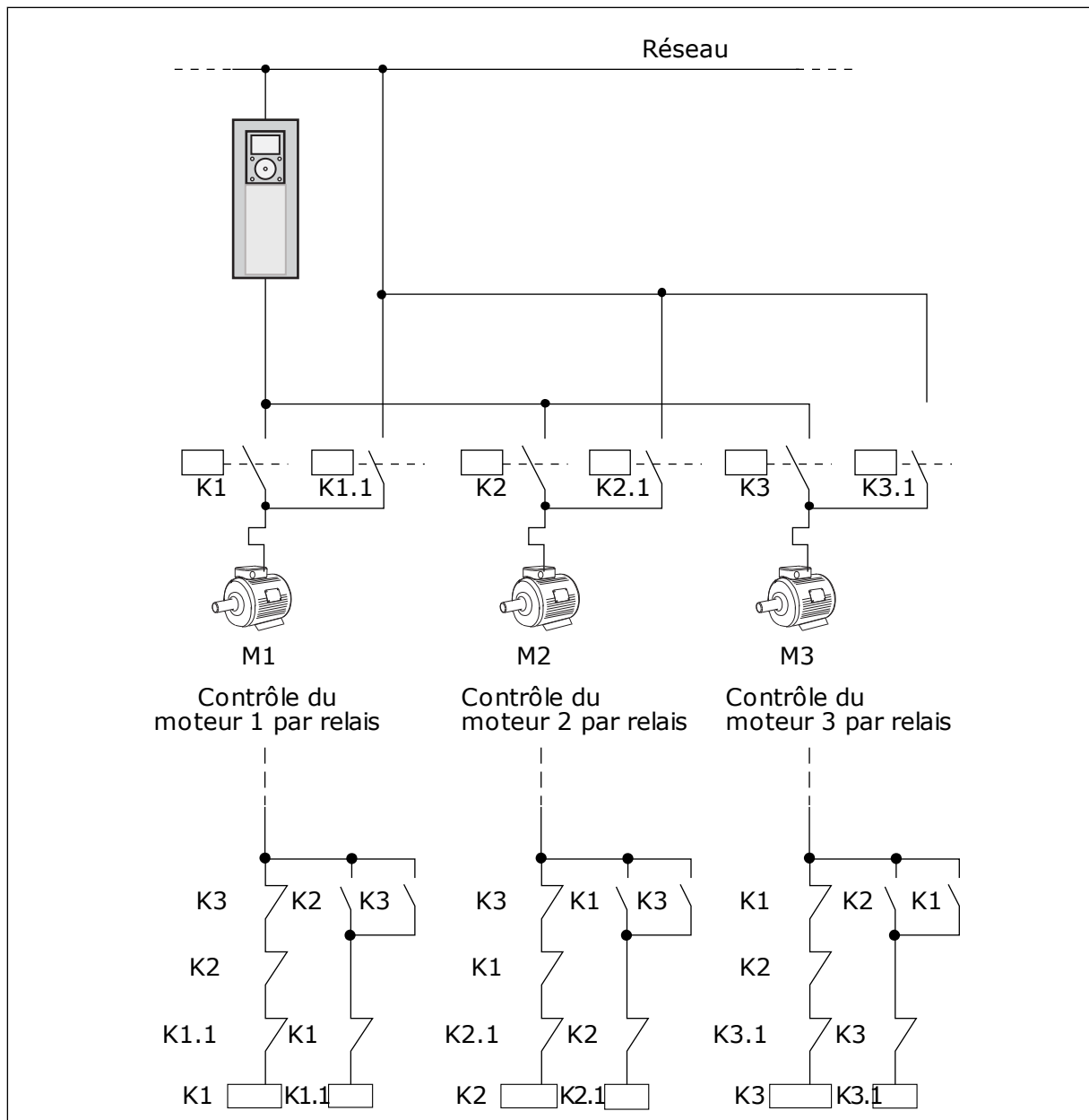
Fig. 84: Sélection 1
