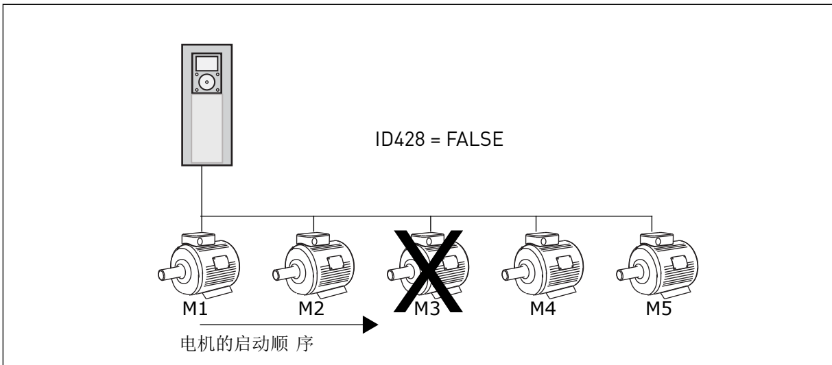
图 81: 互锁逻辑 2
