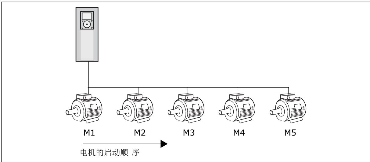
图 80: 互锁逻辑 1
