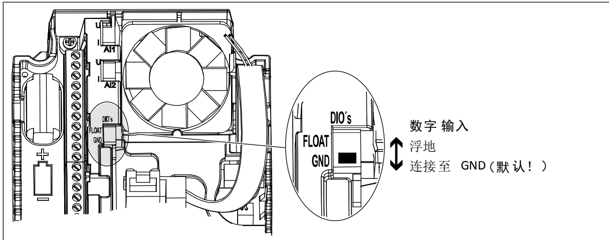
图 5: DIP 开关
