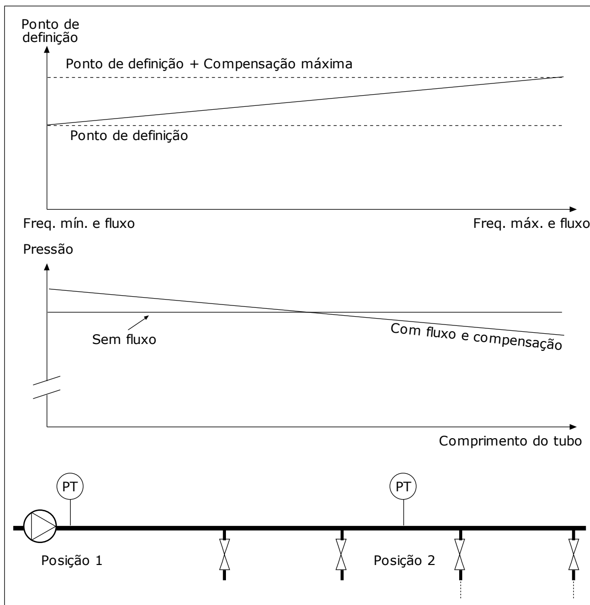
Fig. 75: Ativar ponto de definição 1 para compensação de perda de pressão
