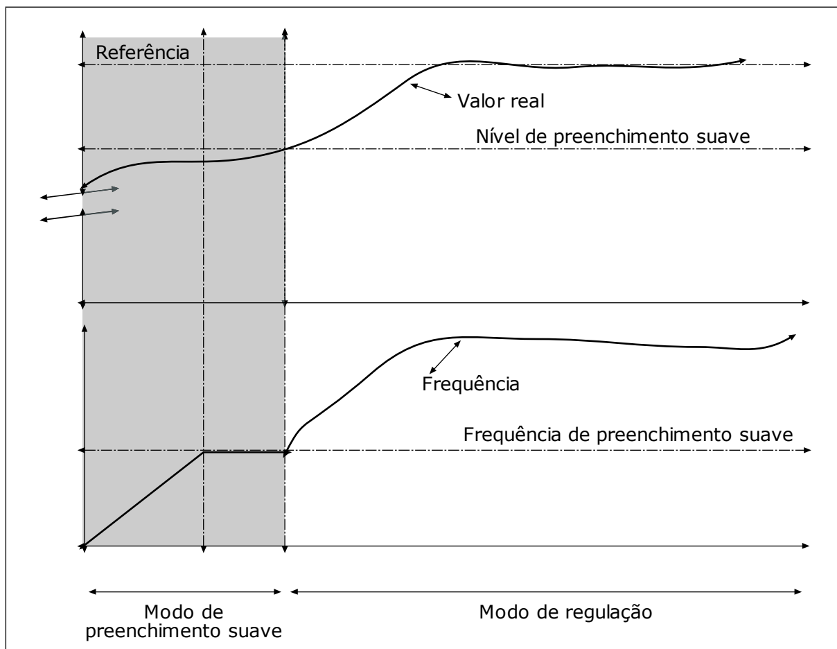
Fig. 76: A Função Preenchimento suave
