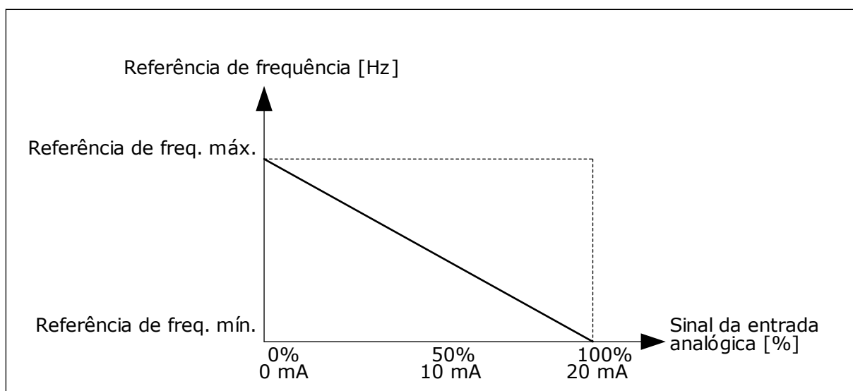
Fig. 51: Inversão do sinal de AI1, seleção 1
