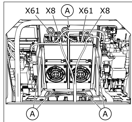
A. Viisi ruuvia
