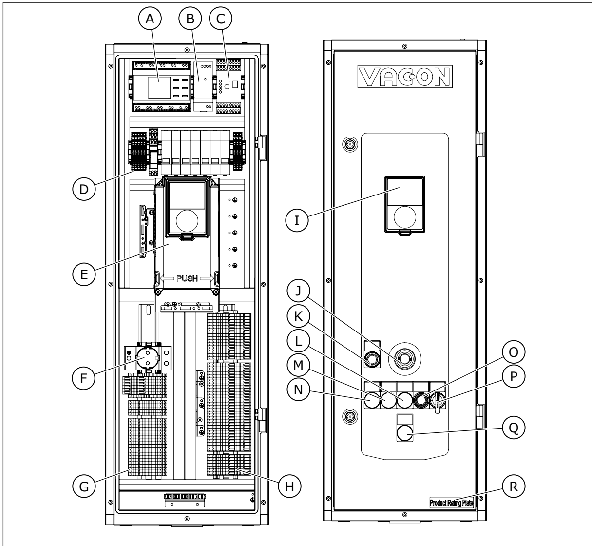
Kuva 42: Kaapin ohjausosaston komponentit
