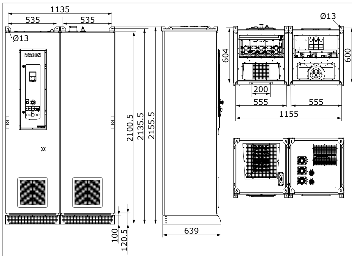
Kuva 9: Valinnaisella sinisuodattimella varustetun kaapin mitat, MR10, [mm], IEC
