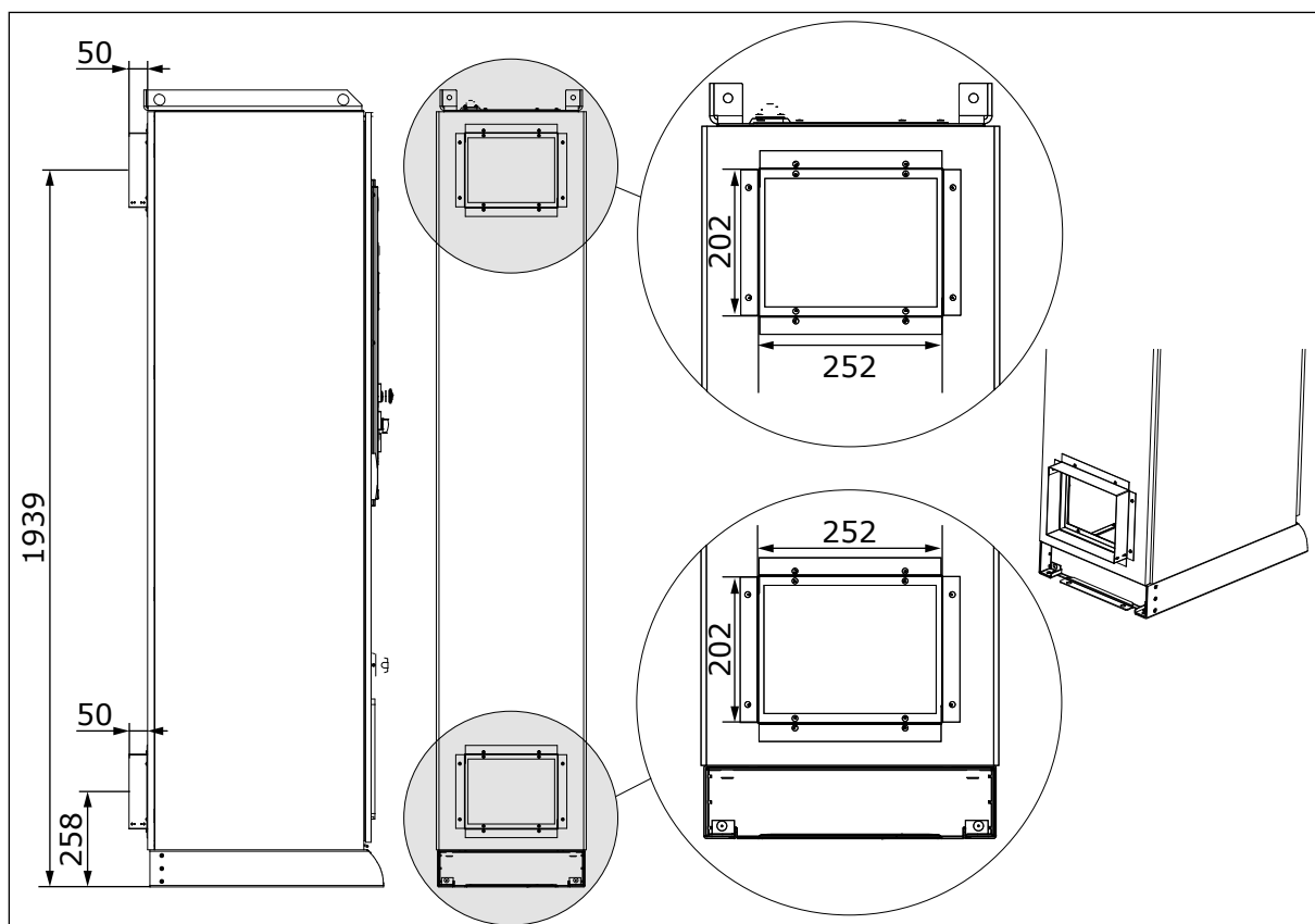
Kuva 26: Takakanavan jäähdytyksen mitat, MR8
