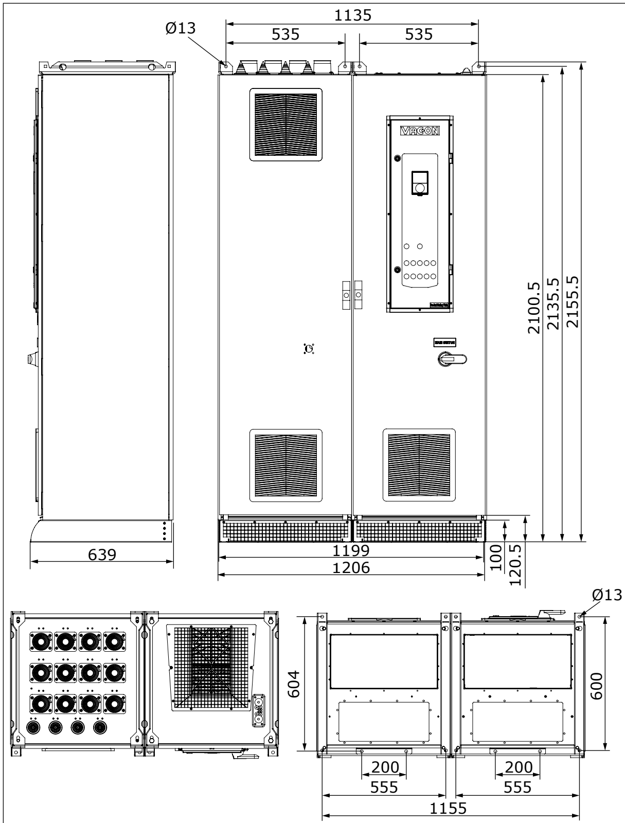
Kuva 7: Valinnaisella yläkaapeloinnilla ja tulokontaktorilla varustetun kaapin mitat, MR10 min. 416 A, [mm], IEC. Katso Taulukko 5.
