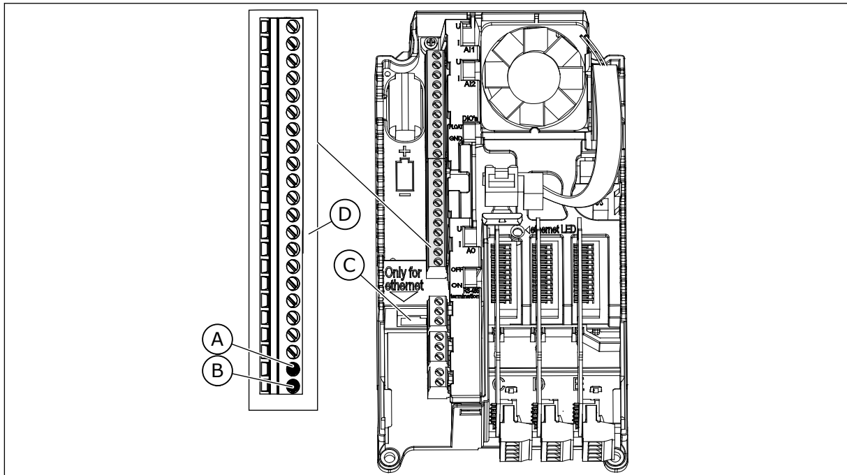
Kuva 43: Ethernet- ja RS485-liitännät
