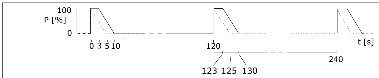
Kuva 45: LD- ja HD-pulssien käyttöjaksot
