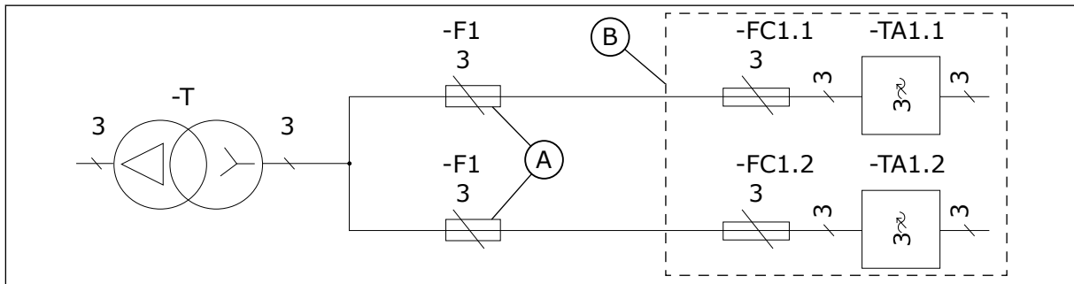
Kuva 34: Sulakkeiden sijainti, MR12
