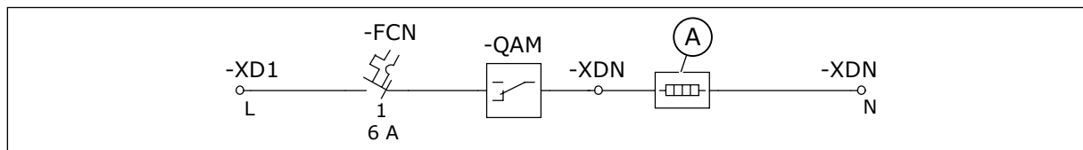
Kuva 17: Moottorin lämmittimen ohjaus
