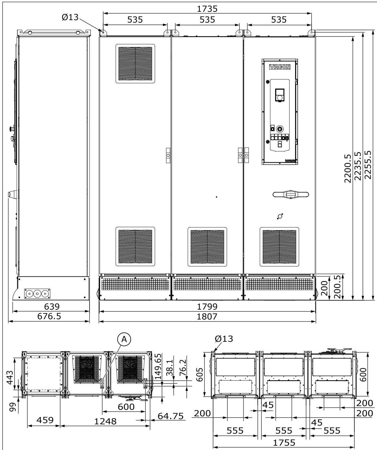
Kuva 15: Valinnaisella yläkaapeloinnilla tai tulokontaktorilla varustetun kaapin mitat, MR12, [mm], NAM. Kuvassa esitetään valinnaisella yläkaapeloinnilla varustettu taajuusmuuttaja.
