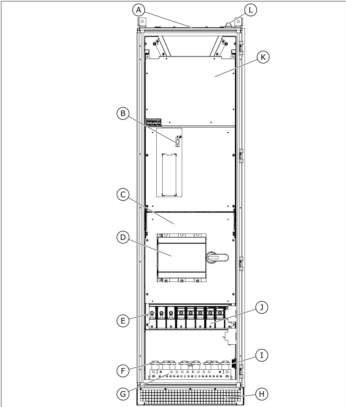
Kuva 37: MR10-malli sisältä ilman suojakansia
