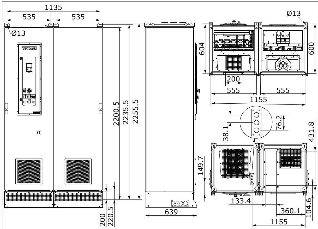
Kuva 16: Valinnaisella sinisuodattimella varustetun kaapin mitat, MR10, [mm], NAM
