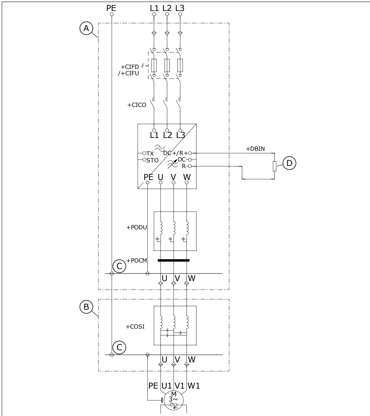
Kuva 28: Kaapin pääpiirikaavio, MR8-MR10
