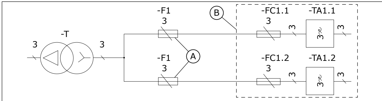
Fig. 30: Emplacement des fusibles, MR12
