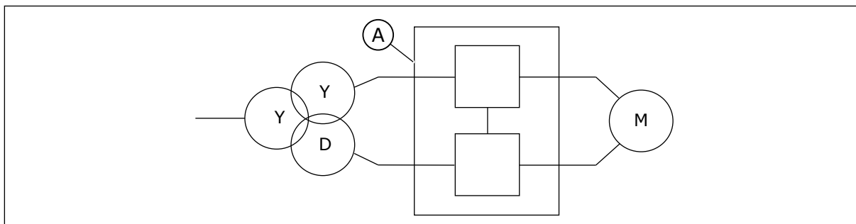
Fig. 28: Le fonctionnement à 12 mesures de MR12
