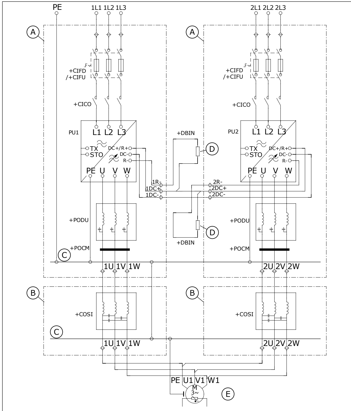
Fig. 27: Principal schéma de circuit de l'armoire, MR12
