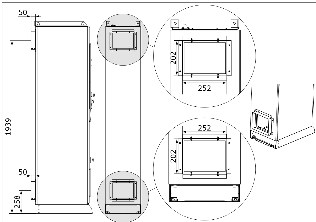
Fig. 24: Dimensions du refroidissement par canal arrière, MR8
