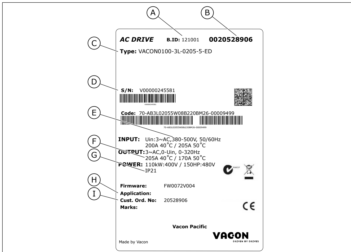
Fig. 2: Étiquette d'emballage des convertisseurs de fréquence Vacon
