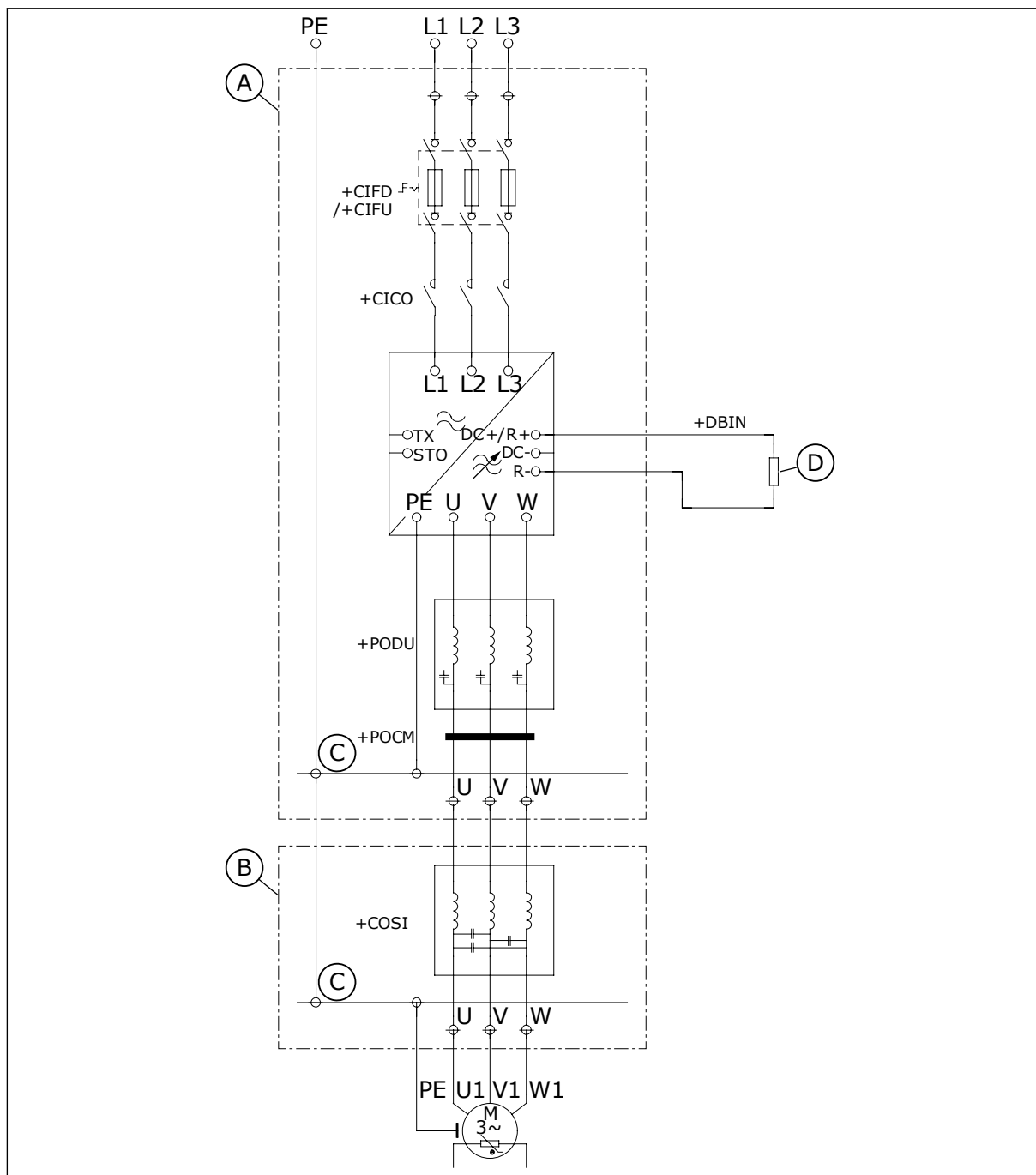
Fig. 26: Principal schéma de circuit de l'armoire, MR8-MR10
