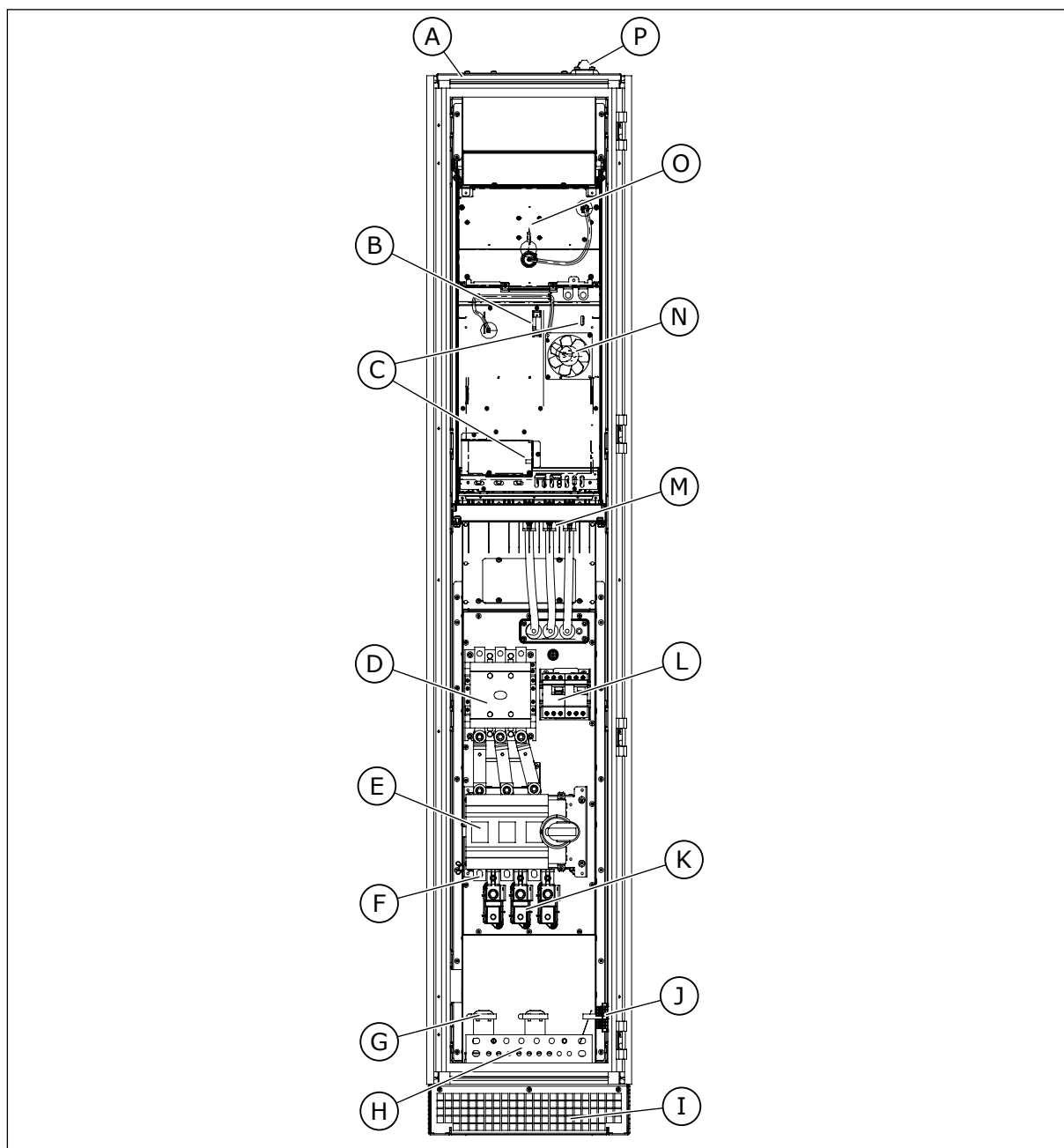
Fig. 33: Disposition intérieure de MR8, sans capots de protection
