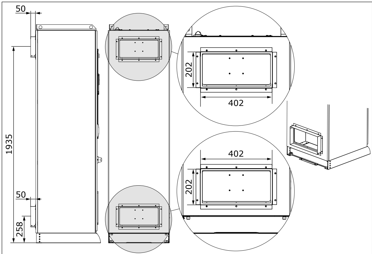
Fig. 25: Dimensions du refroidissement par canal arrière, MR9 et MR10
