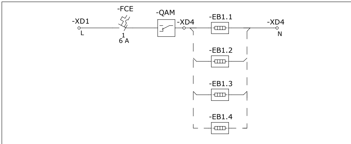
Fig. 16: Résistance de réchauffage de l'armoire
