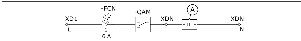
Fig. 15: Commande de la résistance de réchauffage du moteur
