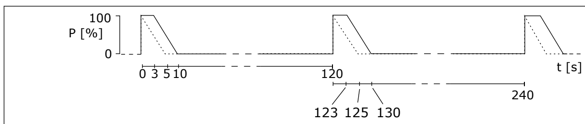
Fig. 43: Les cycles des impulsions de régime normal et de régime intensif
