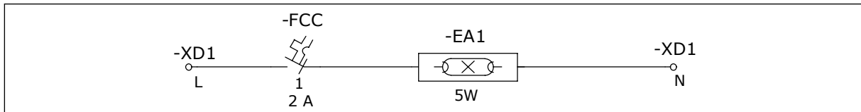
Fig. 17: Éclairage d'armoire
