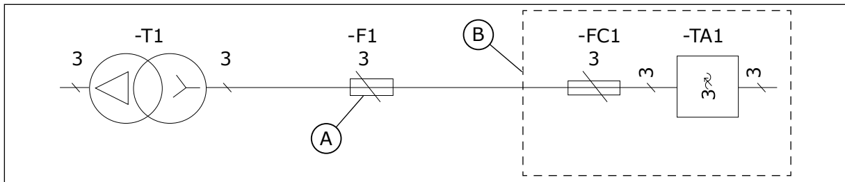
Fig. 29: Emplacement des fusibles, MR8-MR10
