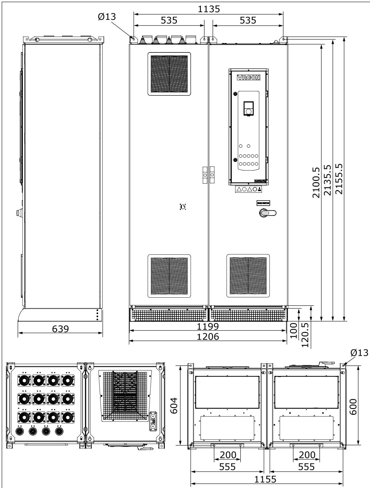
Fig. 7: Dimensions de l'armoire avec le câblage en option par le haut et/ou le contacteur d'entrée, MR10 avec un minimum de 416 A, [mm], CEI. Voir le tableau Table 5.
