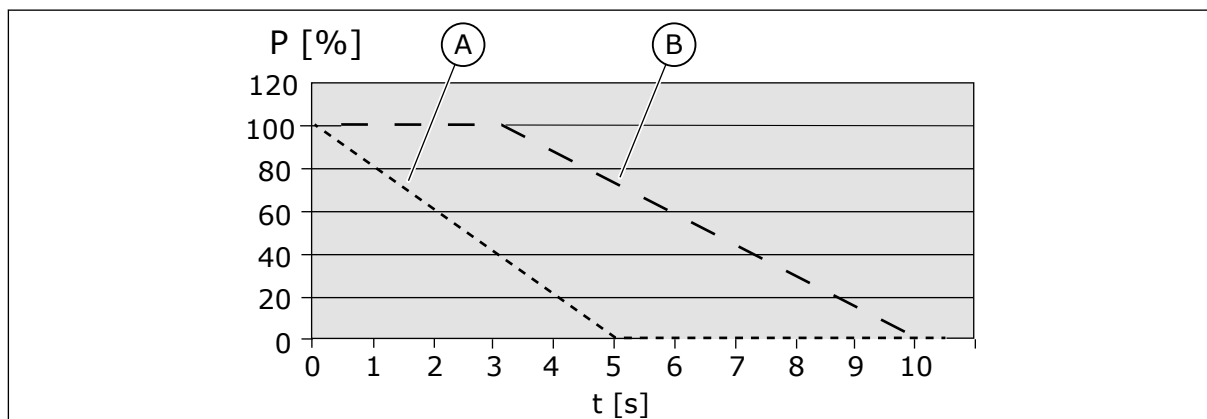
Fig. 42: Les impulsions de régime normal et de régime intensif
