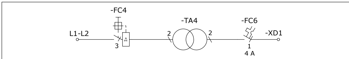
Fig. 18: Transformateur de tension auxiliaire
