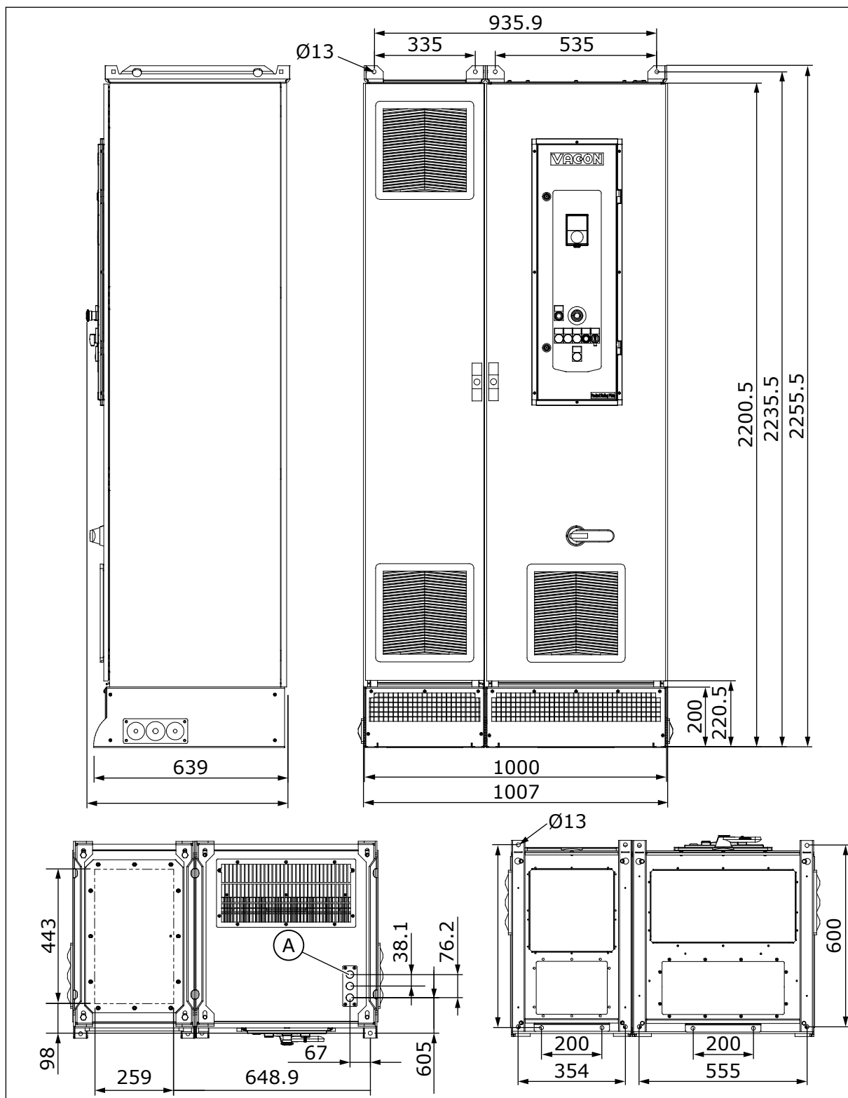
Fig. 13: Dimensions de l'armoire avec le câblage en option par le haut et/ou le contacteur d'entrée, MR10 avec un minimum de 416 A, [mm], NAM
