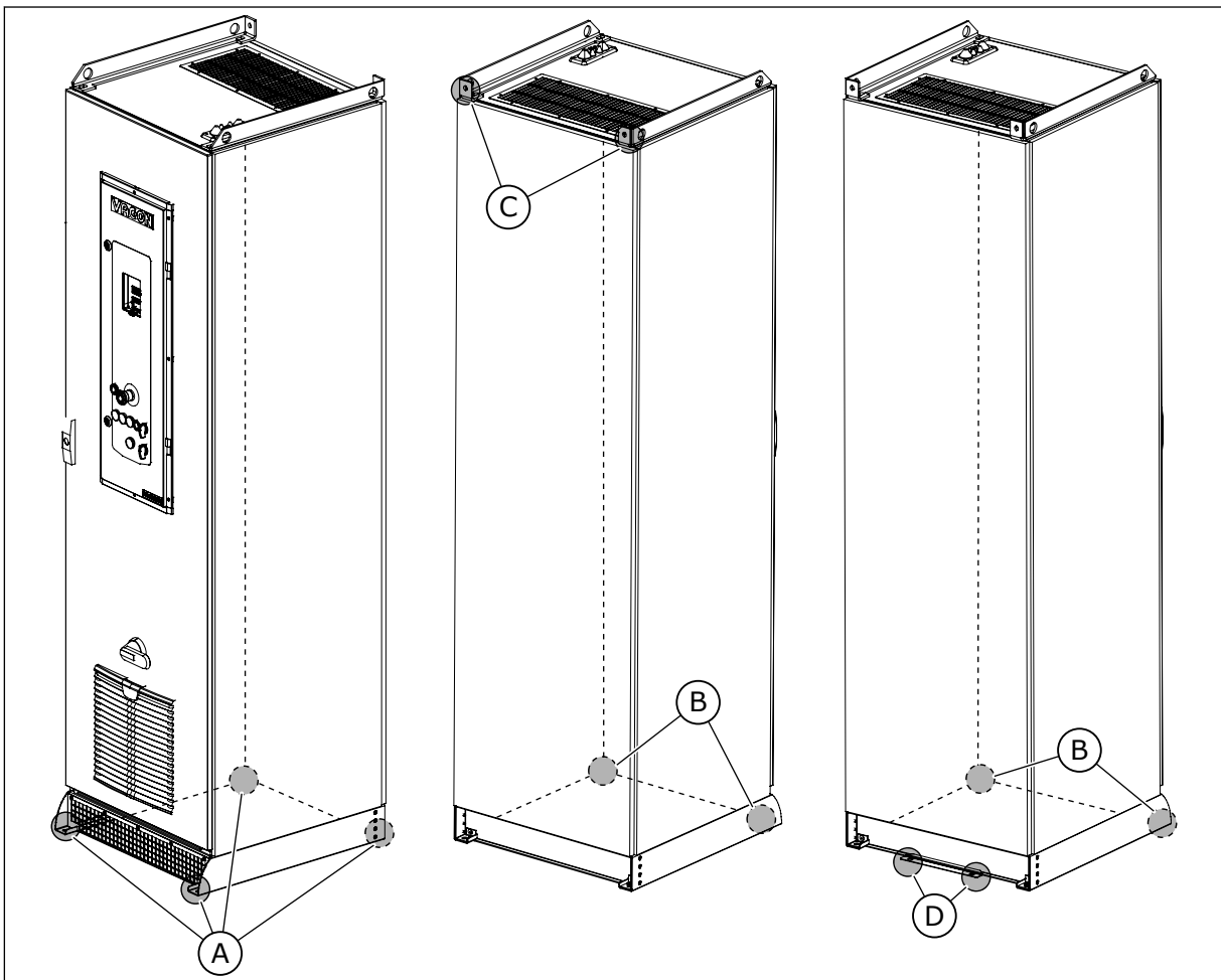
Fig. 22: Points de fixation de l'armoire.
