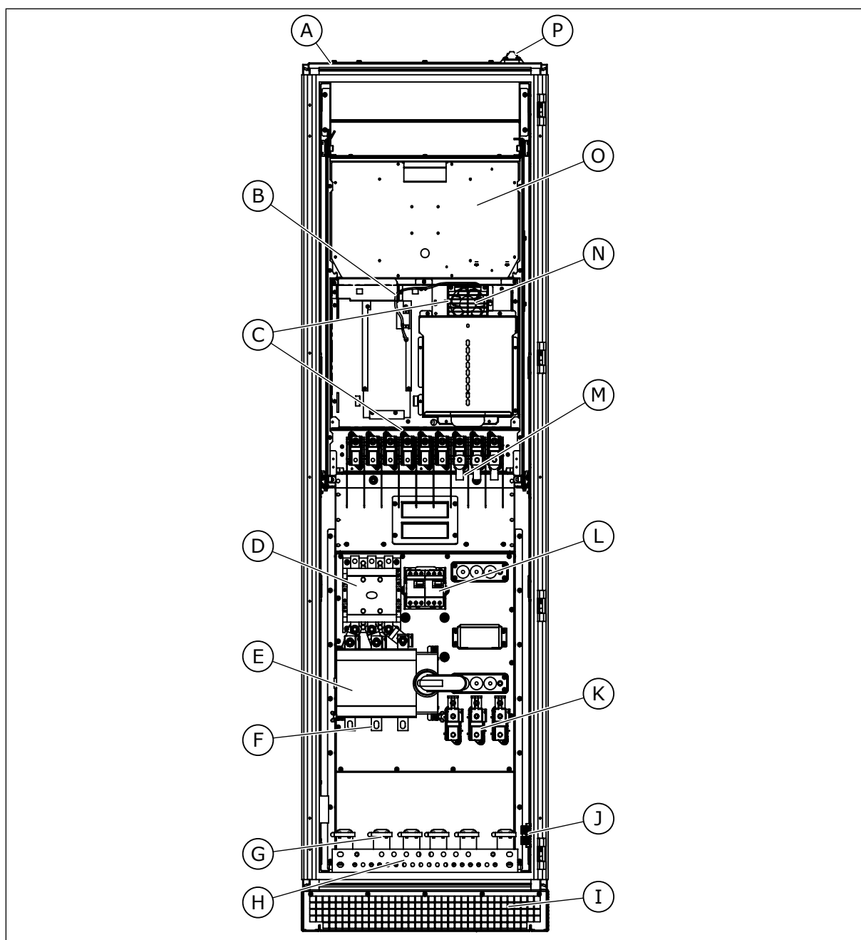
Fig. 34: Disposition intérieure de MR9, sans capots de protection
