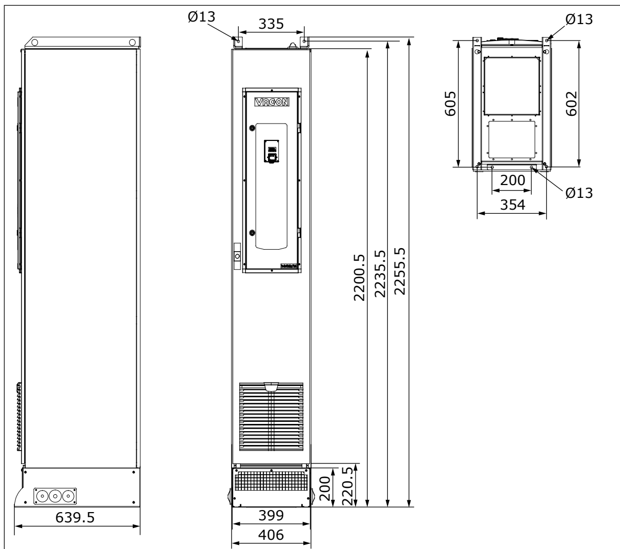
Fig. 9: Dimensions de l'armoire par défaut, MR8, [mm], NAM
