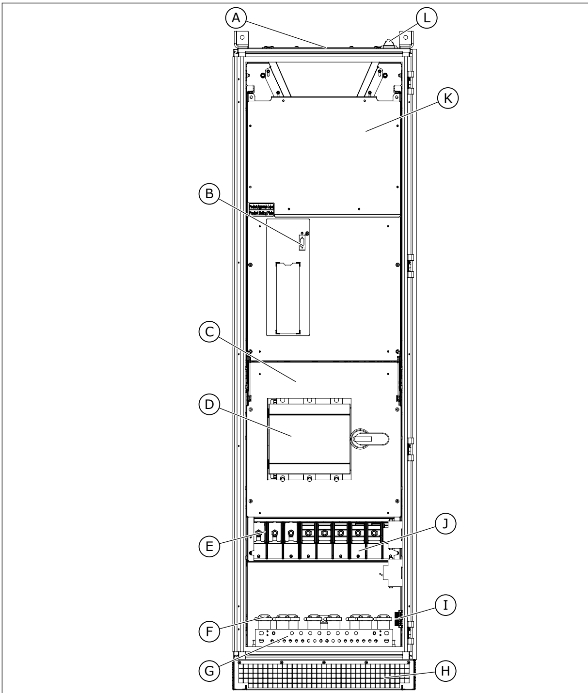
Fig. 35: Disposition intérieure de MR10, sans capots de protection
