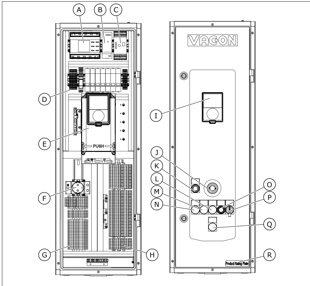
Fig. 40: Composants du compartiment de commande de l'armoire
