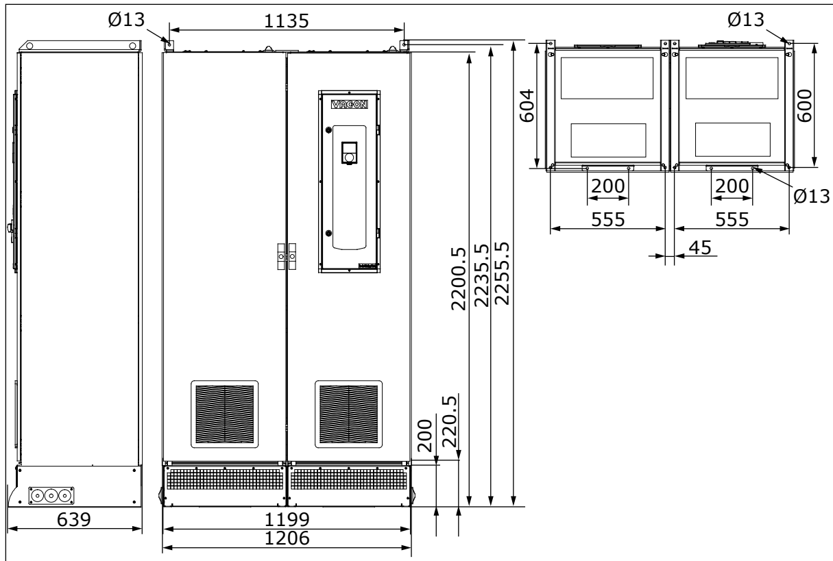
Afb. 11: De afmetingen van de standaardkast, MR12, [mm], NAM
