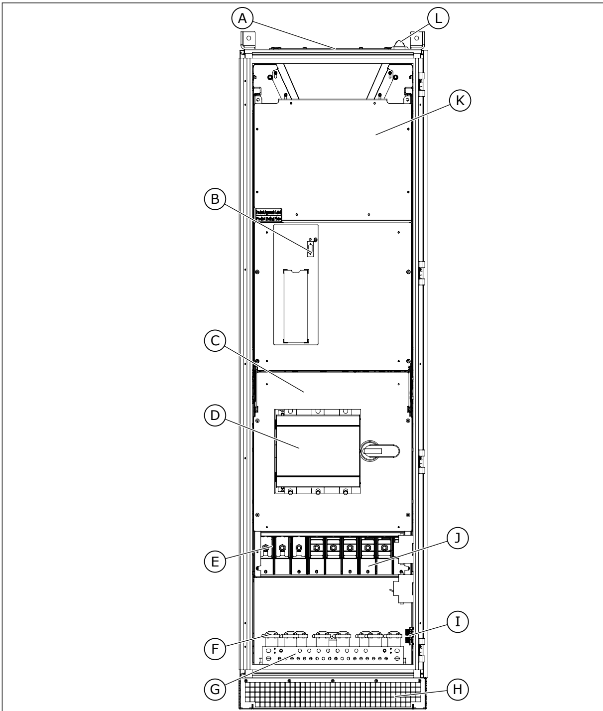
Afb. 35: De indeling binnen in de MR10, zonder beschermingskappen
