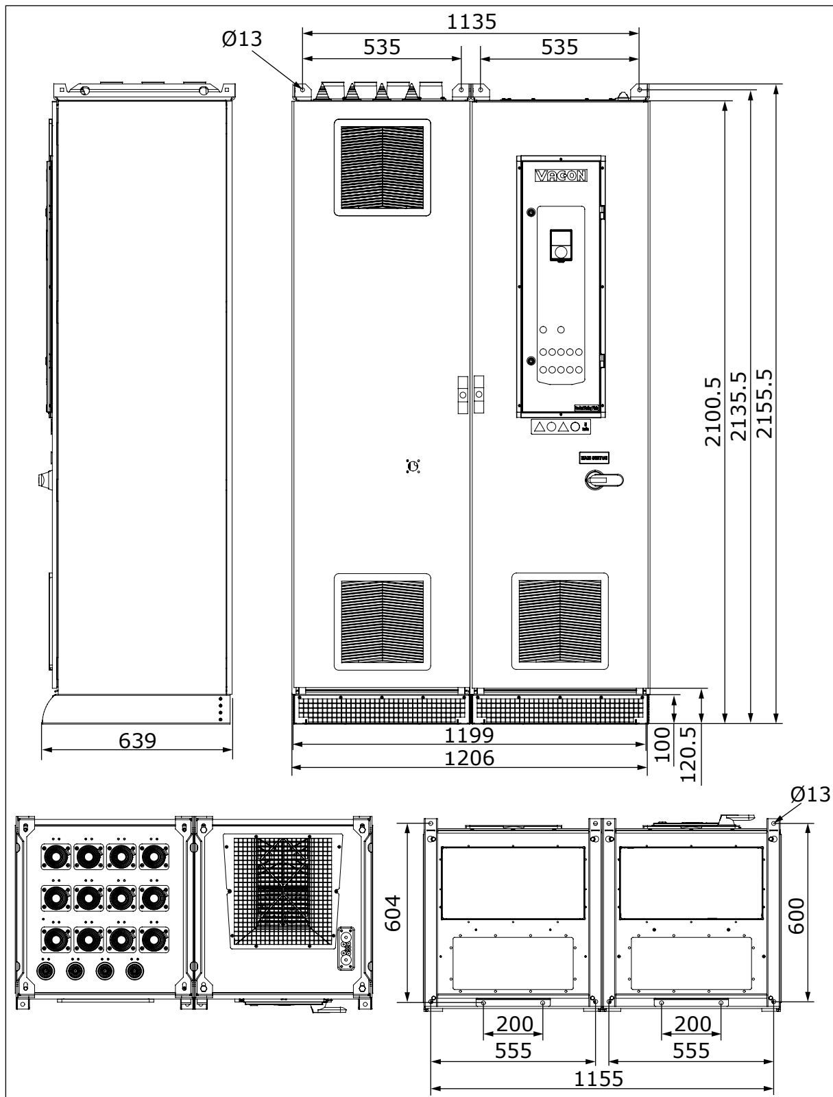
Afb. 7: De afmetingen van de kast met de optionele bekabeling via de bovenzijde en/of de netmagneetschakelaar, MR10 met min. 416 A, [mm], IEC. Zie tabel Tabel 5.
