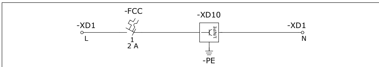
Afb. 21: de AC-contactdoos klant
