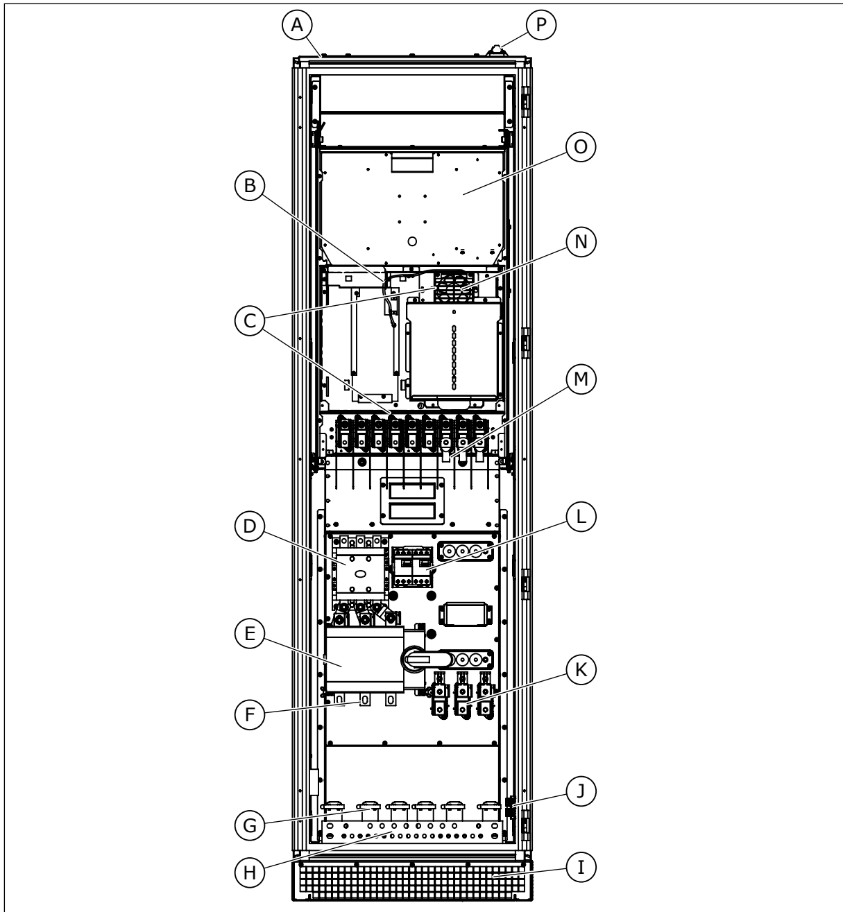
Afb. 34: De indeling binnen in de MR9, zonder beschermingskappen
