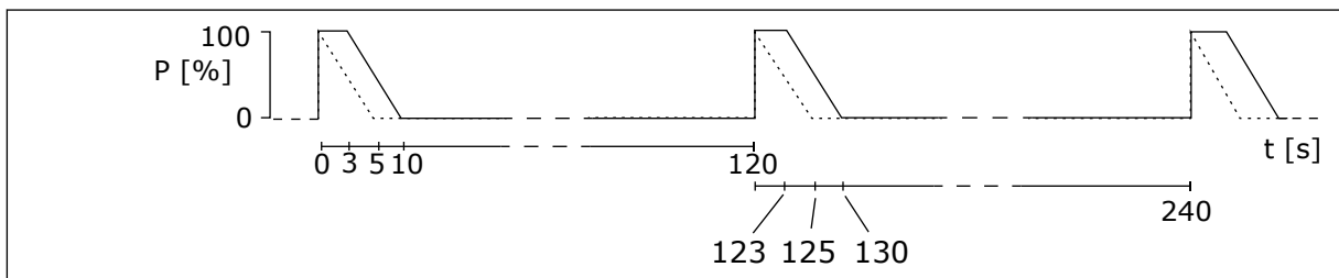
Afb. 43: Gebruikscycli van pulsen licht en zwaar gebruik
