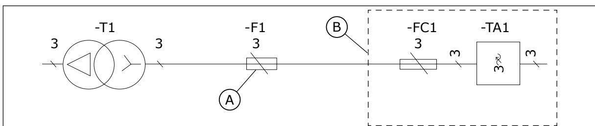
Afb. 29: Locatie van de zekeringen, MR8-MR10
