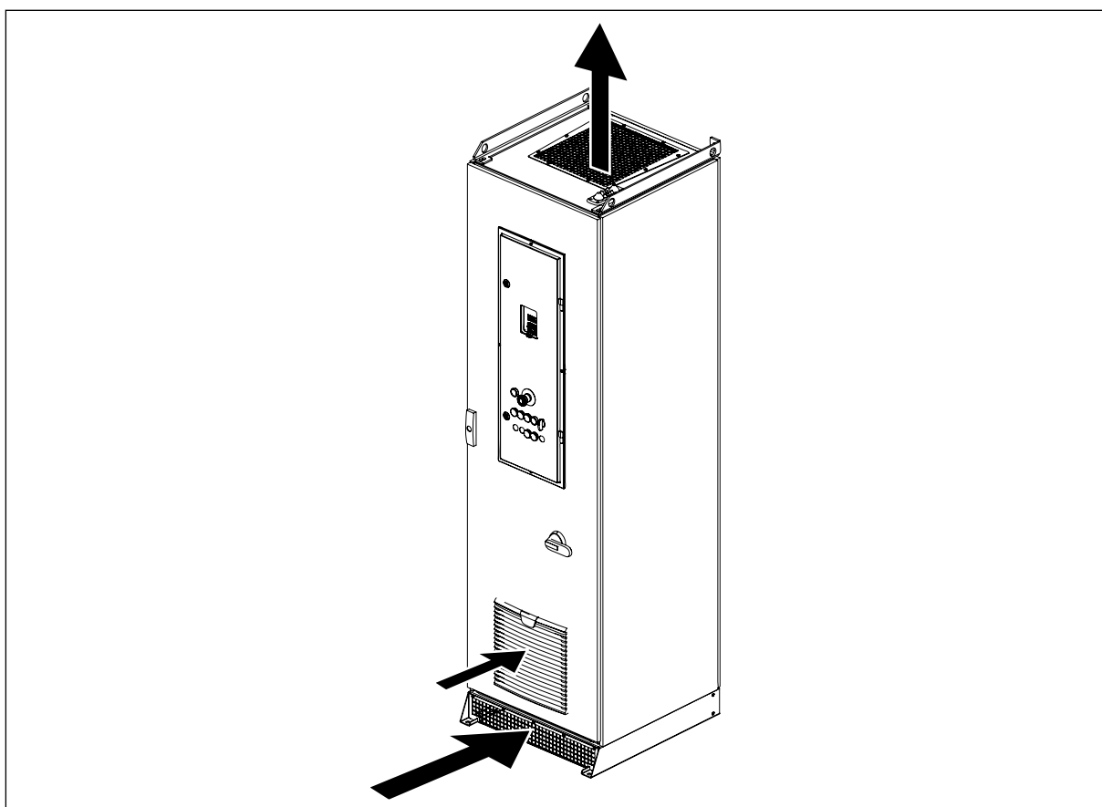
Afb. 23: De circulatie van koellucht
