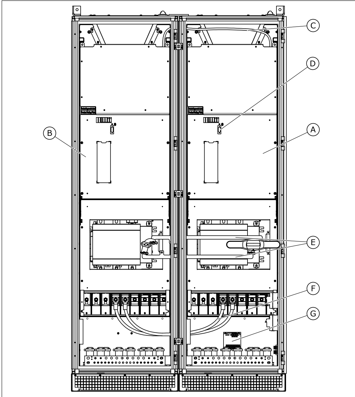
Afb. 36: De indeling binnen in de MR12, zonder beschermingskappen
