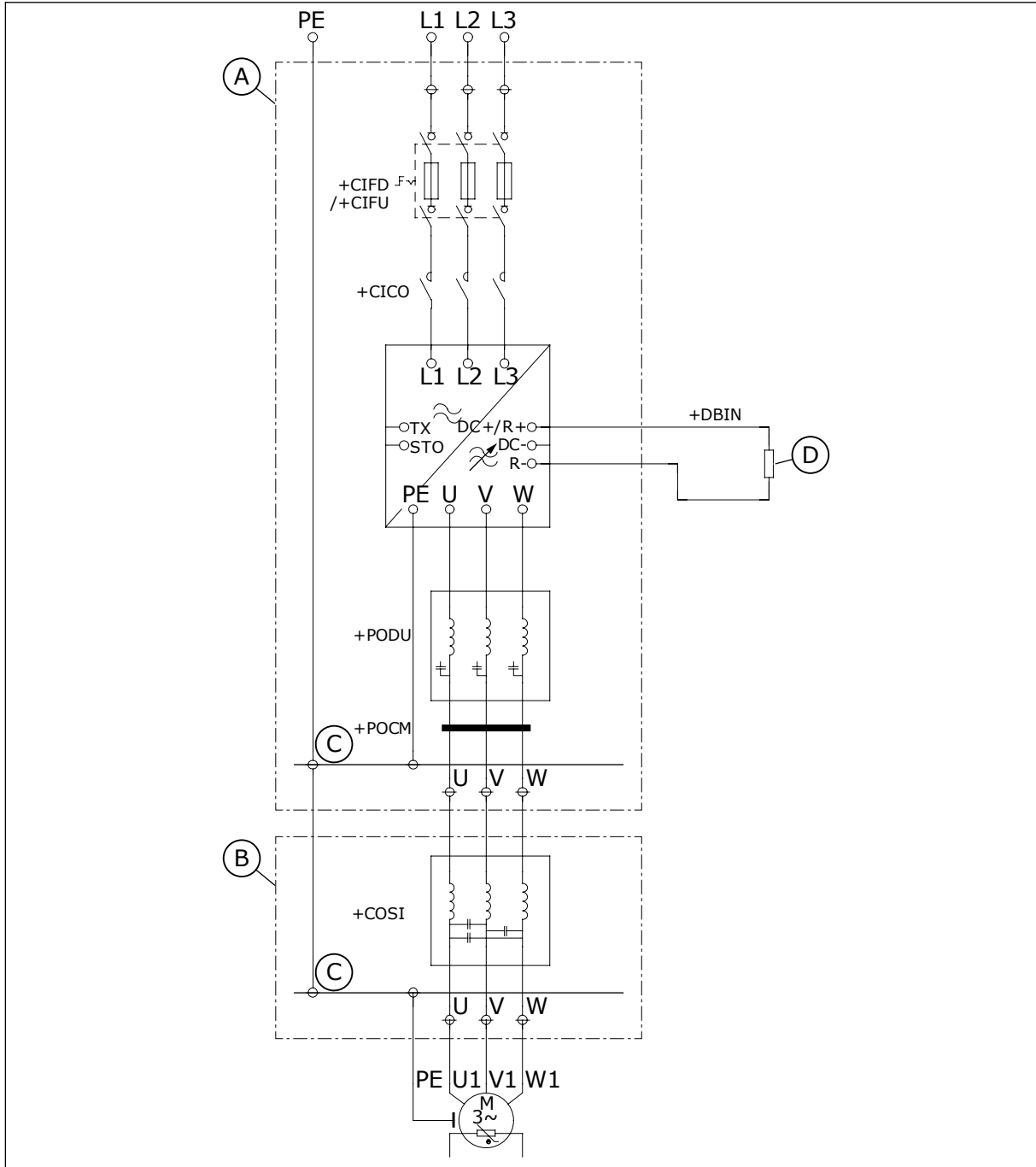
Afb. 26: Hoofdcircuitschema van de kast, MR8-MR10
