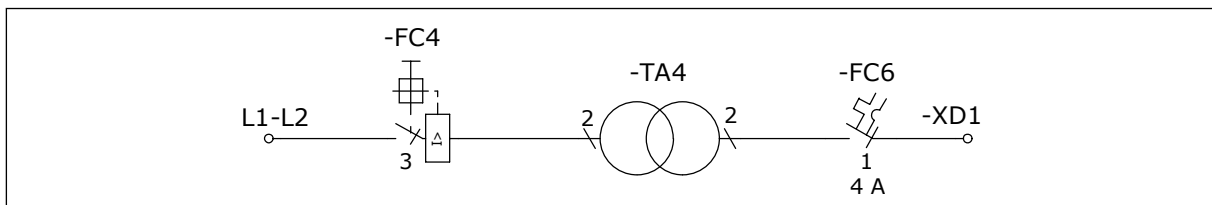
Afb. 18: De hulpspanningstransformator
