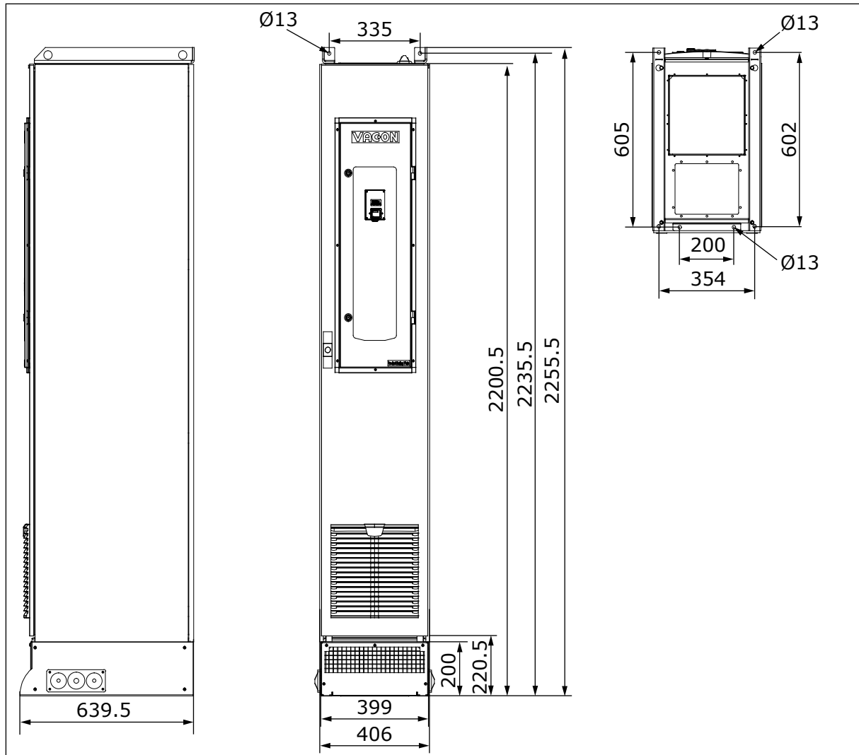
Afb. 9: De afmetingen van de standaardkast, MR8, [mm], NAM
