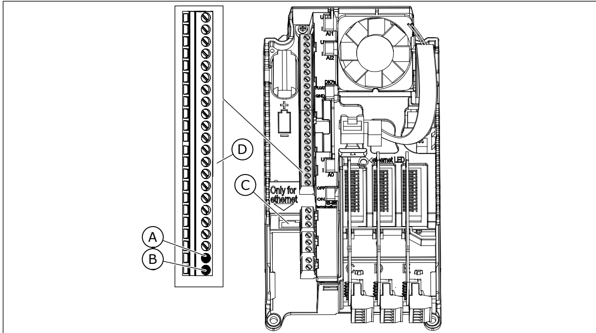
Afb. 41: Ethernet- en RS485-aansluitingen
