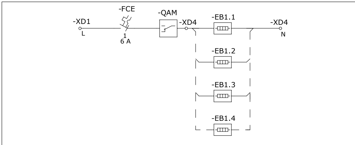
Afb. 16: De kastverwarming
