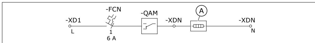
Afb. 15: De besturing van de motorverwarming
