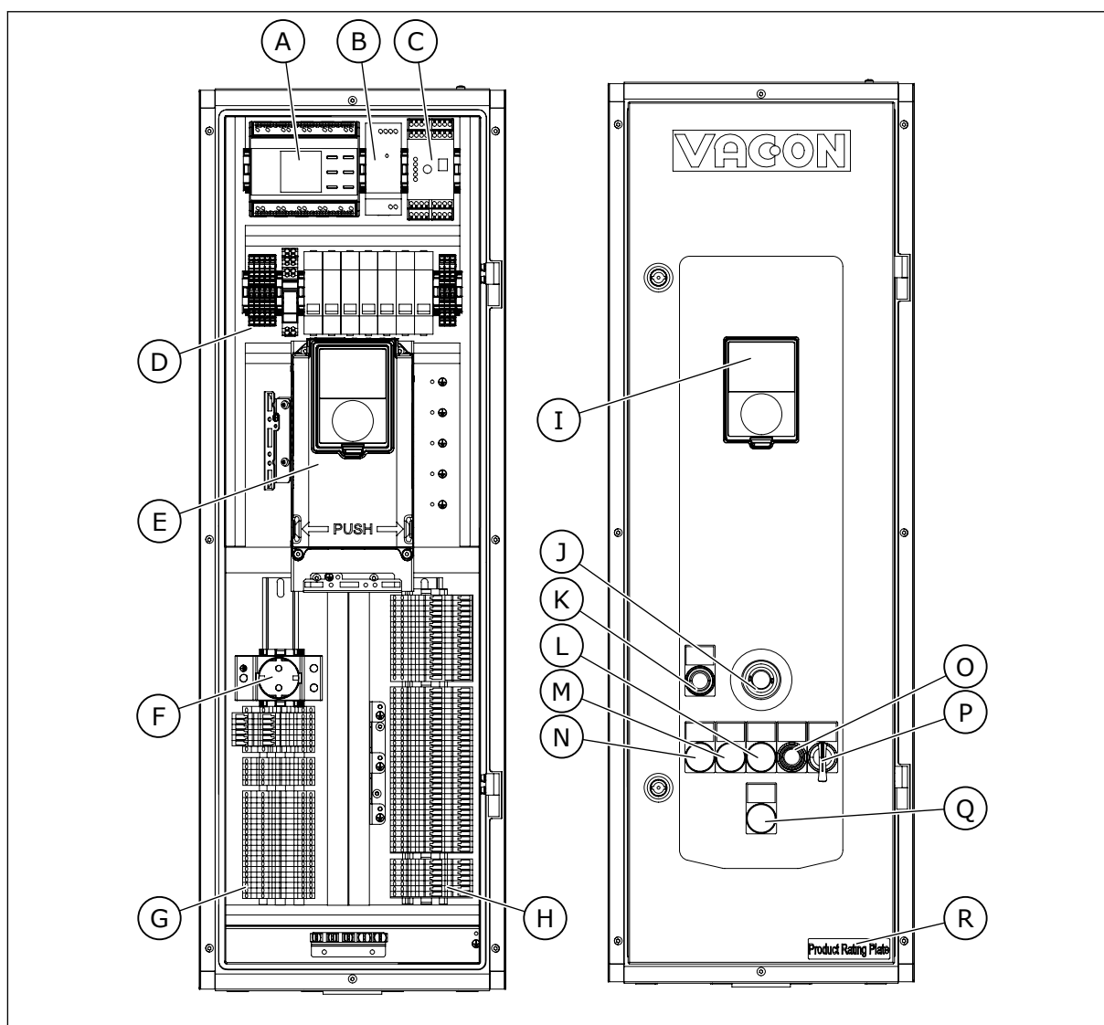
Afb. 40: De componenten van het besturingscomponent van de kast
