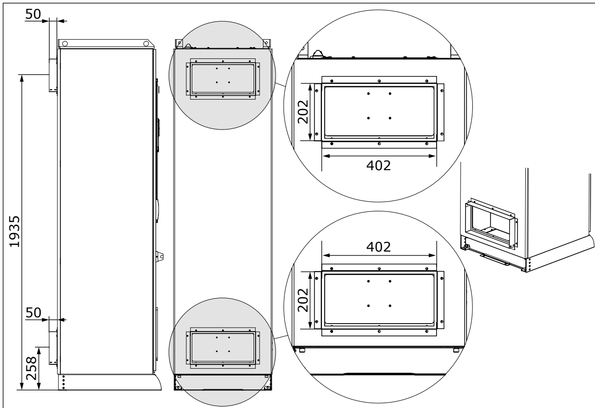
Afb. 25: Afmetingen voor de achterkanaalkoeling, MR9 en MR10
