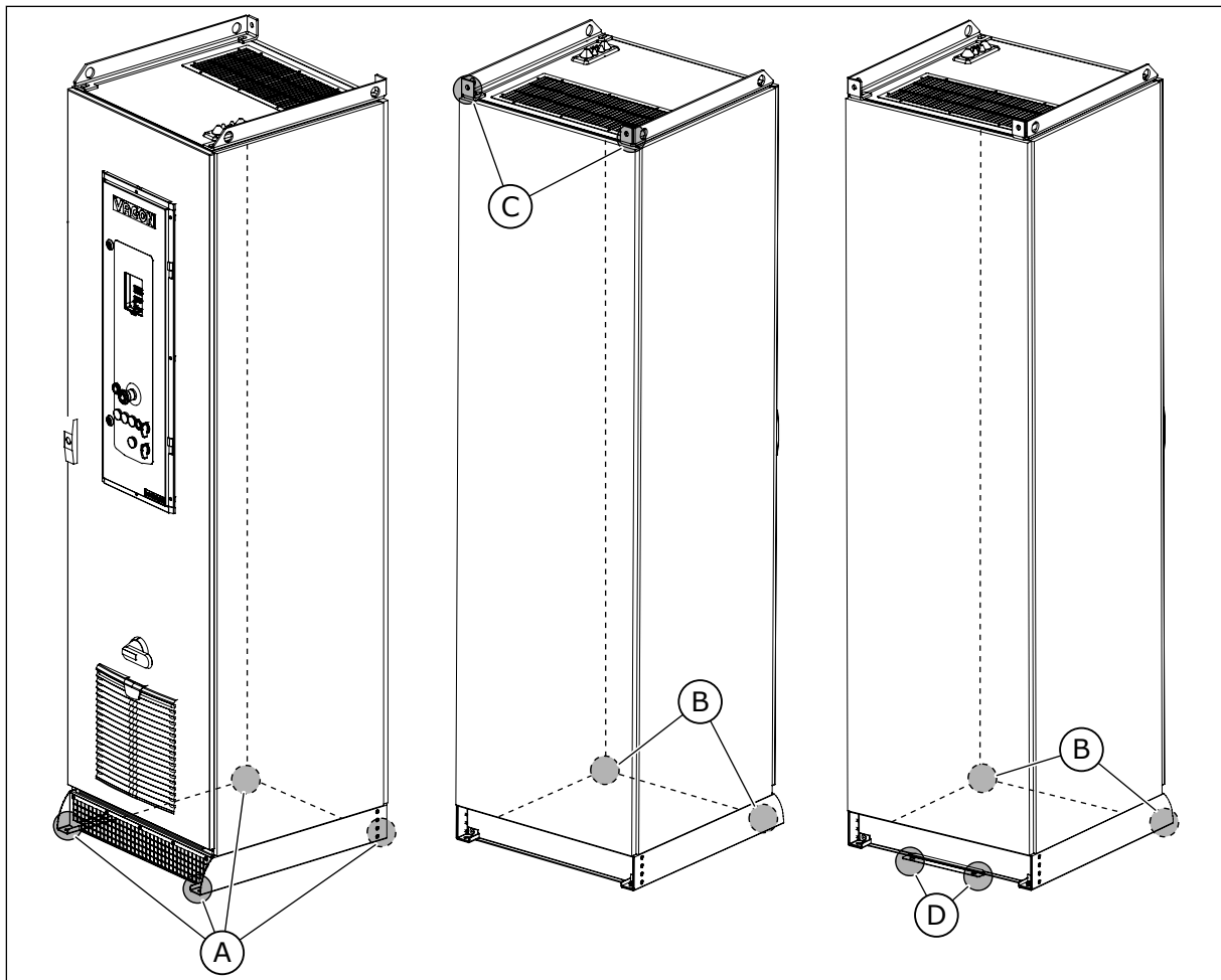
Afb. 22: De bevestigingspunten van de kast
