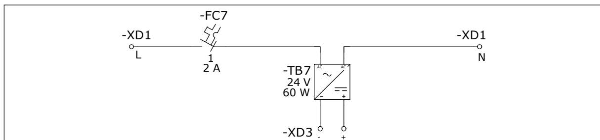
Afb. 20: De 24 VDC-voeding
