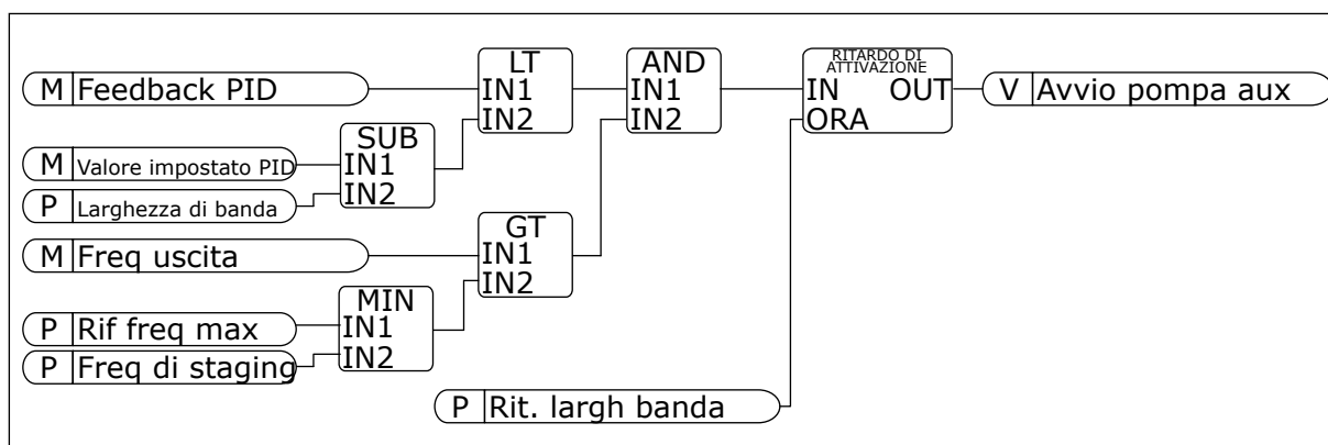
Fig. 101: Frequenza di staging
