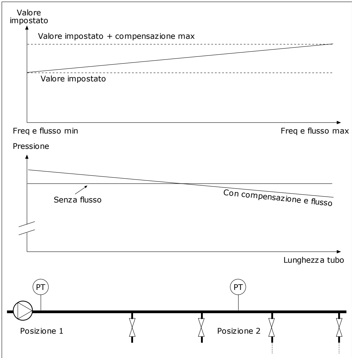
Fig. 85: Abilitazione del valore impostato 1 per compensare la perdita di pressione
