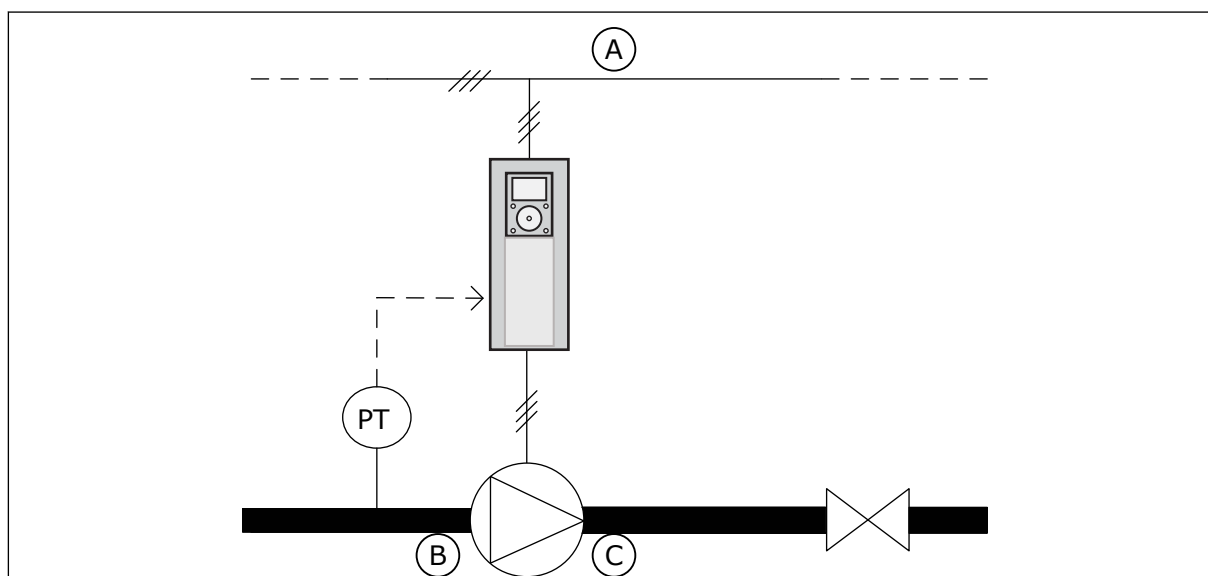
Fig. 86: la posizione del sensore di pressione
