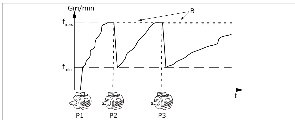
Fig. 91: Controllo nel modo inverter singolo
