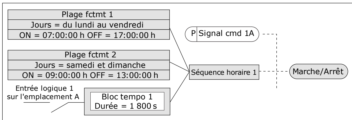
Fig. 78: La séquence horaire 1 est utilisée en tant que signal de commande pour la commande de démarrage en lieu et place d'une entrée logique
