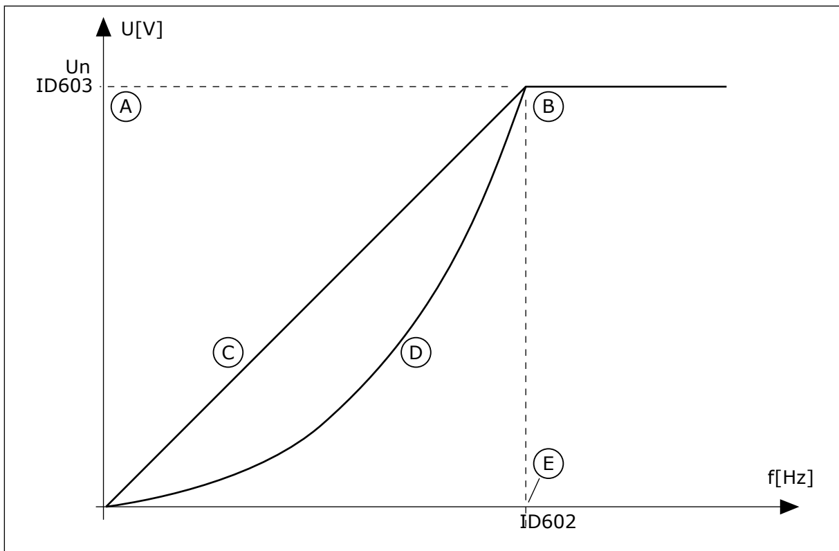
Afb. 38: Lineaire en kwadratische aanpassing van de motorspanning
