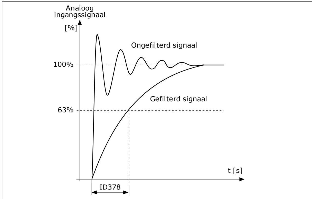
Afb. 56: Het AI1-signaalfilter
