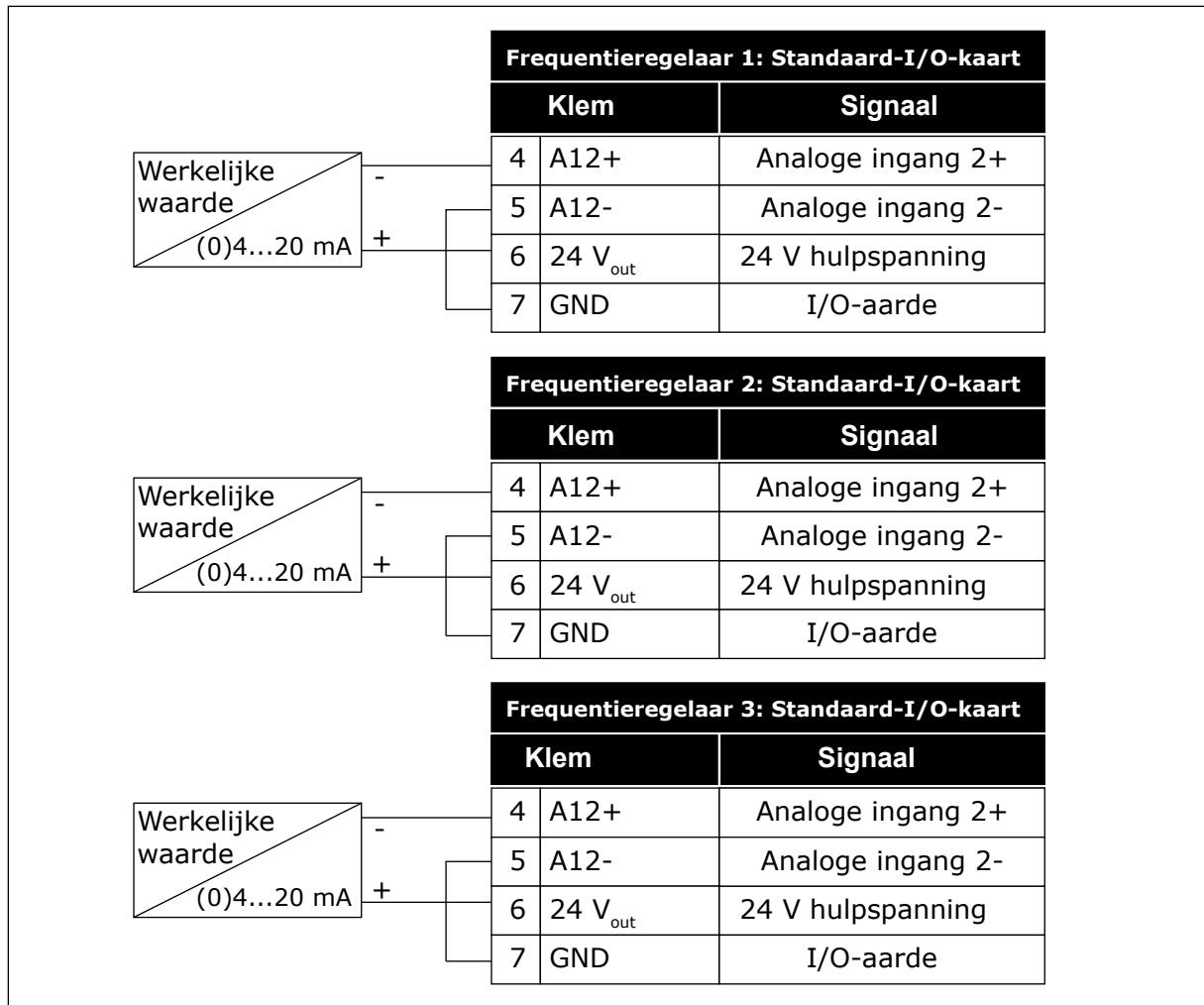
Afb. 94: Bedrading van terugkoppelingssensoren per frequentieregelaar
