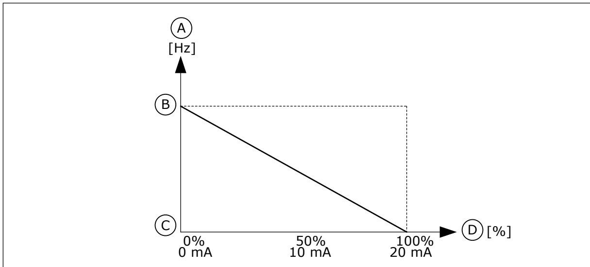
Afb. 61: AI1-signaalinversie bij parameterwaarde 1
