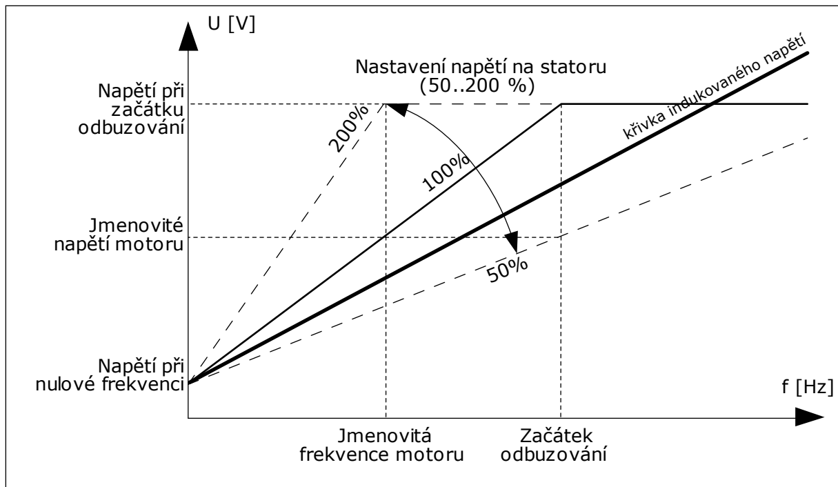
Obr. 37: Nastavení napětí na statoru
