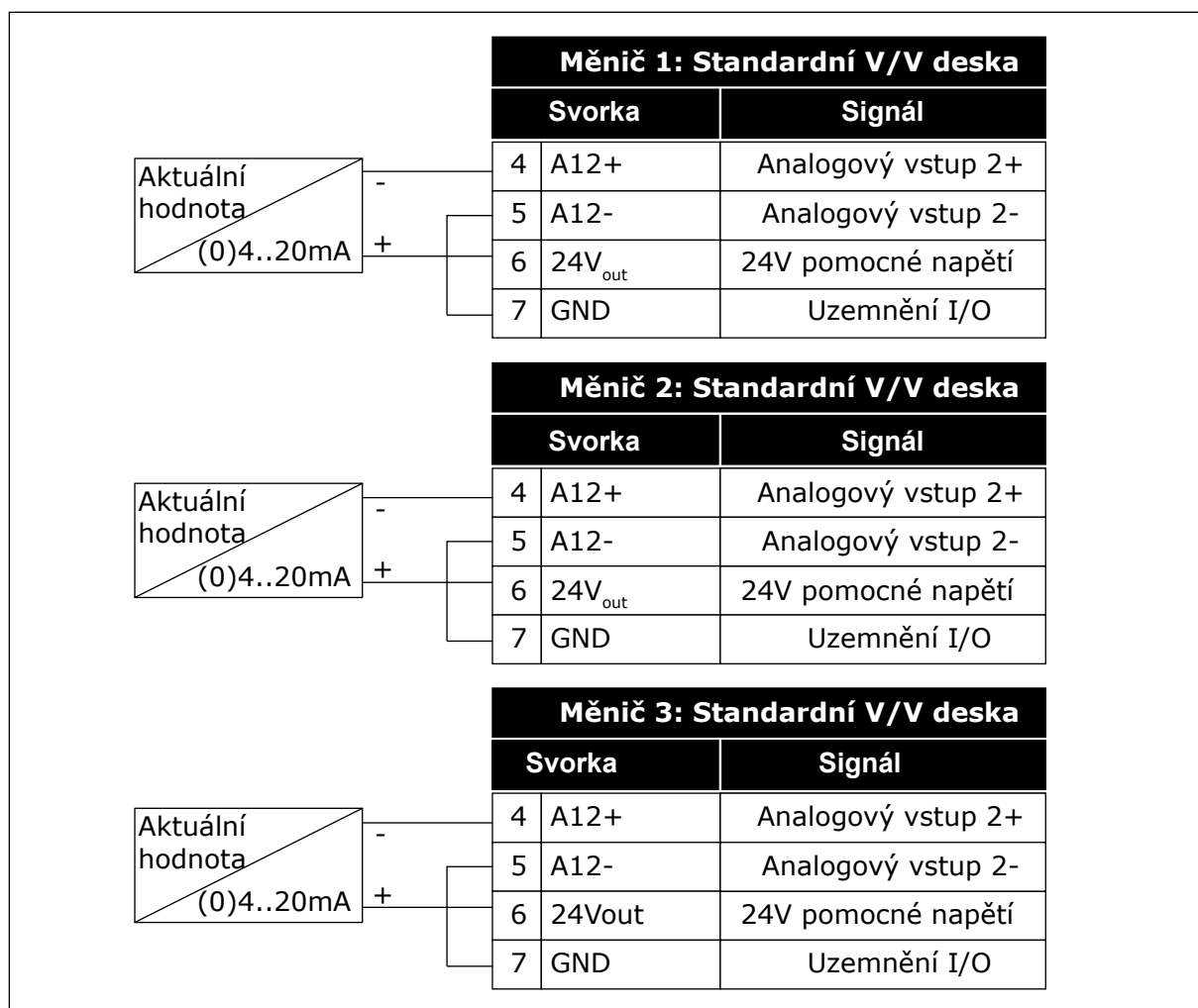
Obr. 94: Zapojení snímačů zpětné vazby pro každý měnič
