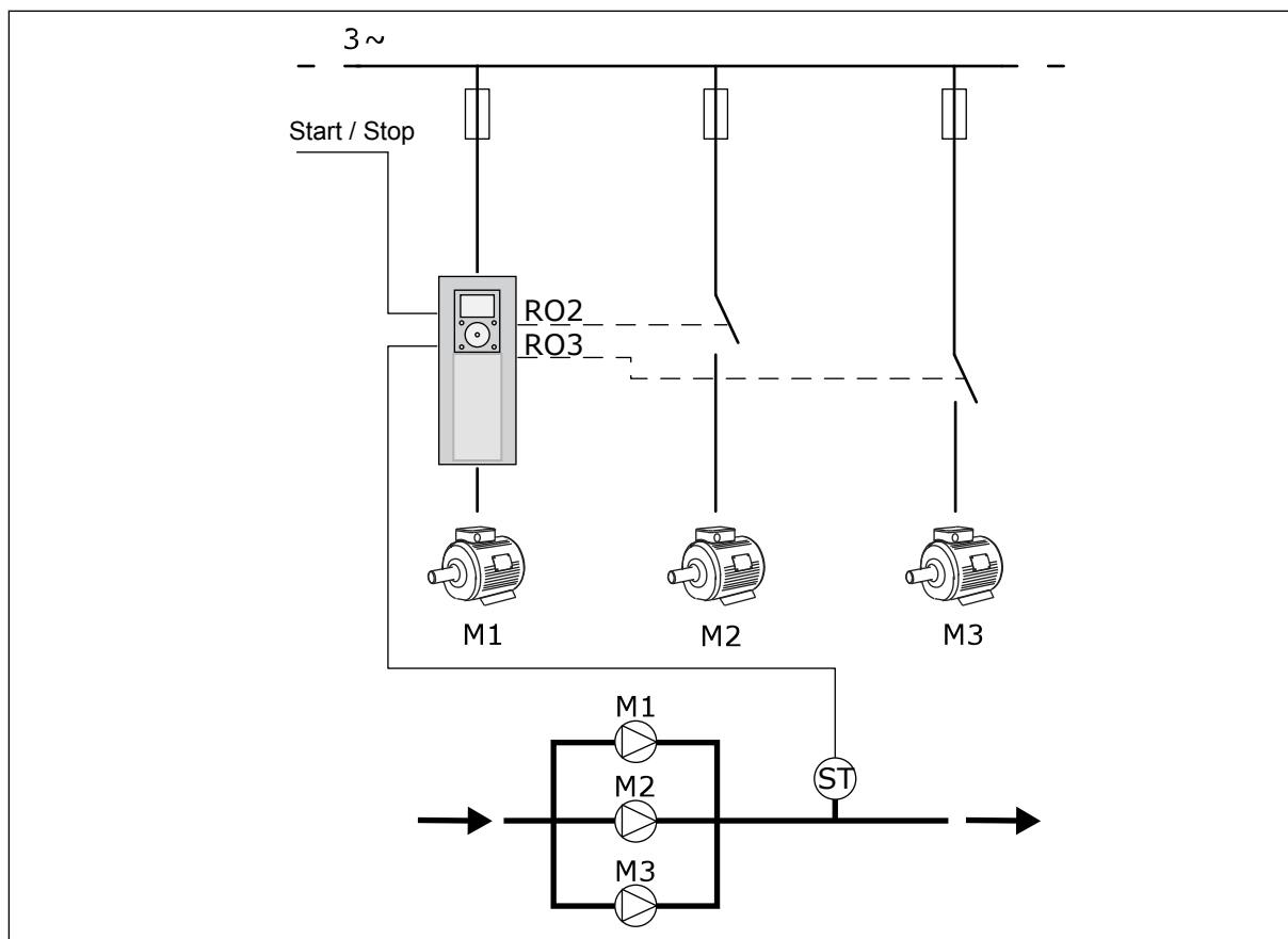
Obr. 8: Konfigurace multi-čerpádků (se samostatným měničem)
