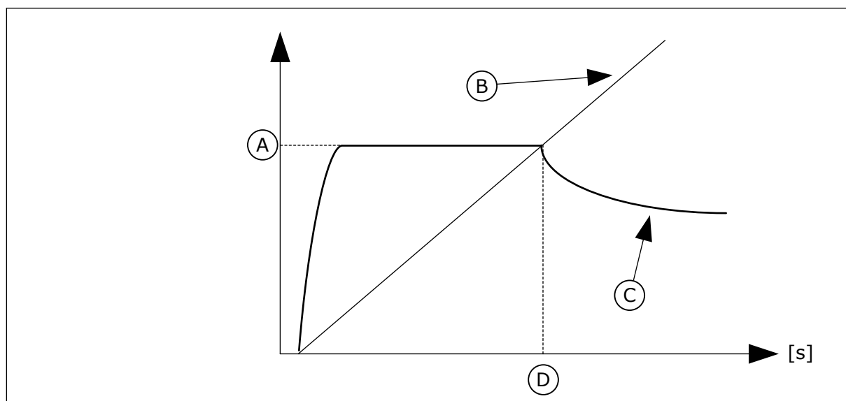
Fig. 40: I/f-startparameterne
