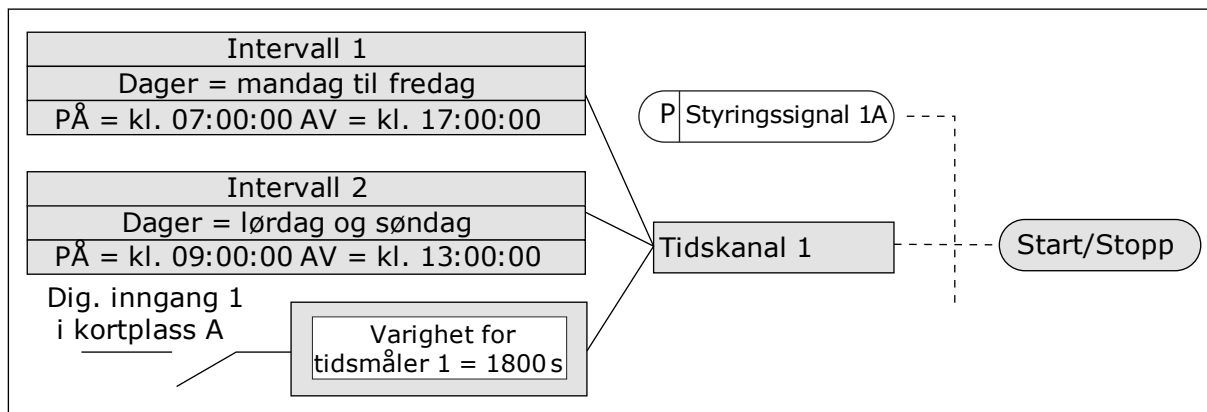
Fig. 78: Tidskanal 1 brukes som styresignal for startkommandoen i stedet for en digital inngang.
