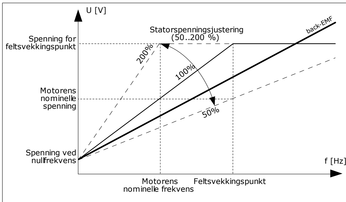
Fig. 37: Statorspeningsjusteringen
