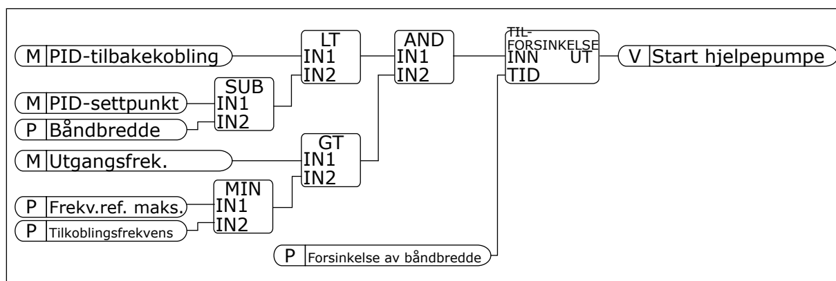
Fig. 101: Tilkoblingsfrekvens
