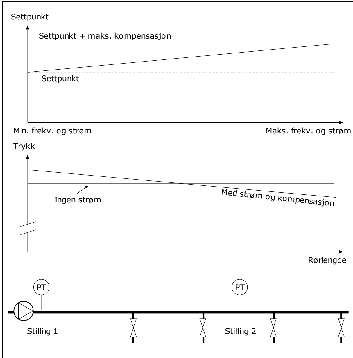
Fig. 85: Aktivere settpunkt 1 for kompensasjon for trykktap
