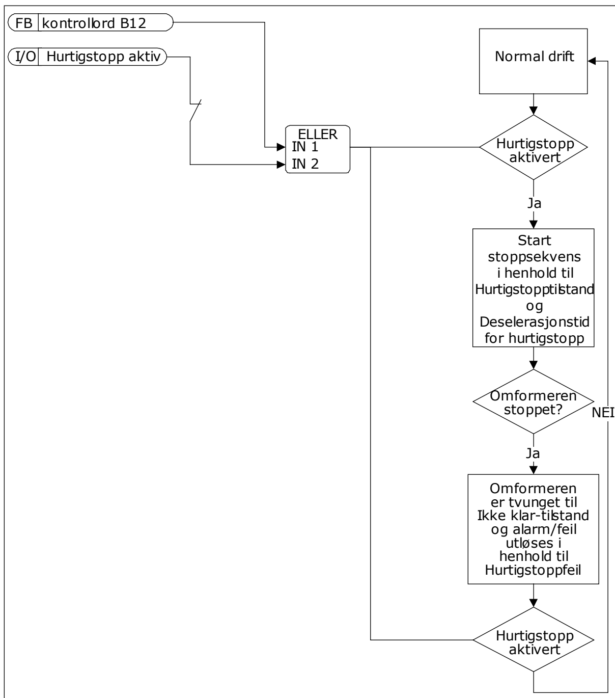
Fig. 71: Hurtigstoplogikken
