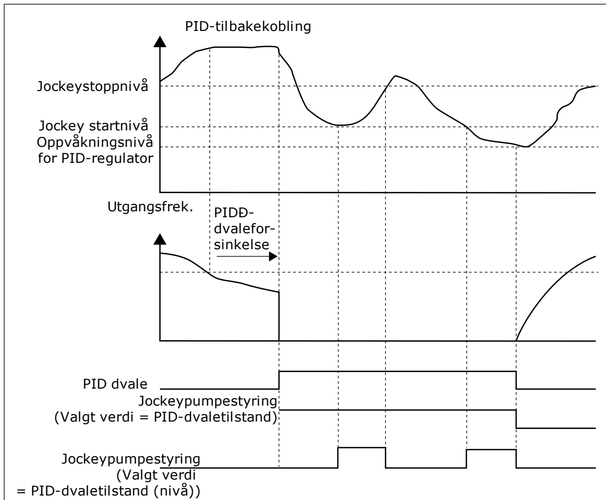
Fig. 105: Jockeypumpefunksjonen
