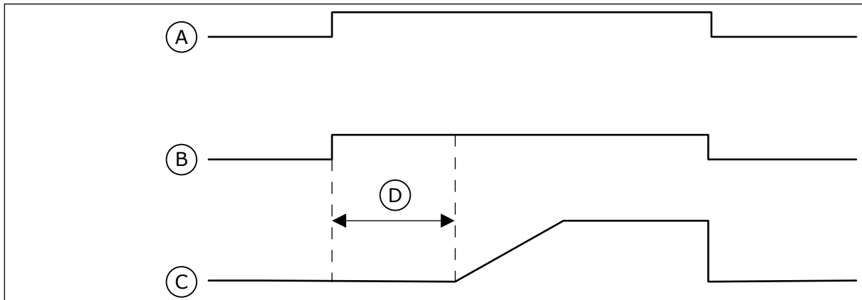
Fig. 106: Sugepumpefunksjonen
