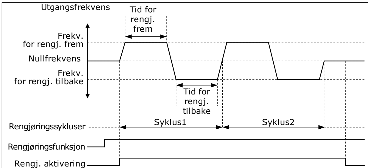
Fig. 104: Autorengjøringsfunksjonen
