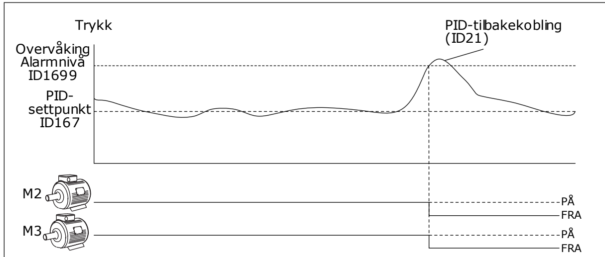
Fig. 100: Funksjonen Overtrykksovervåking
