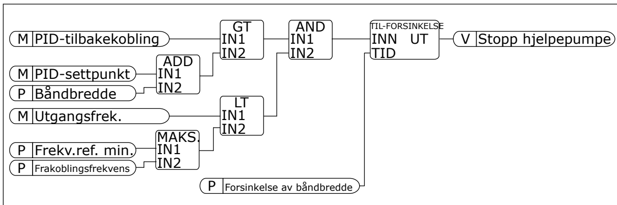
Fig. 102: Frakoblingsfrekvens
