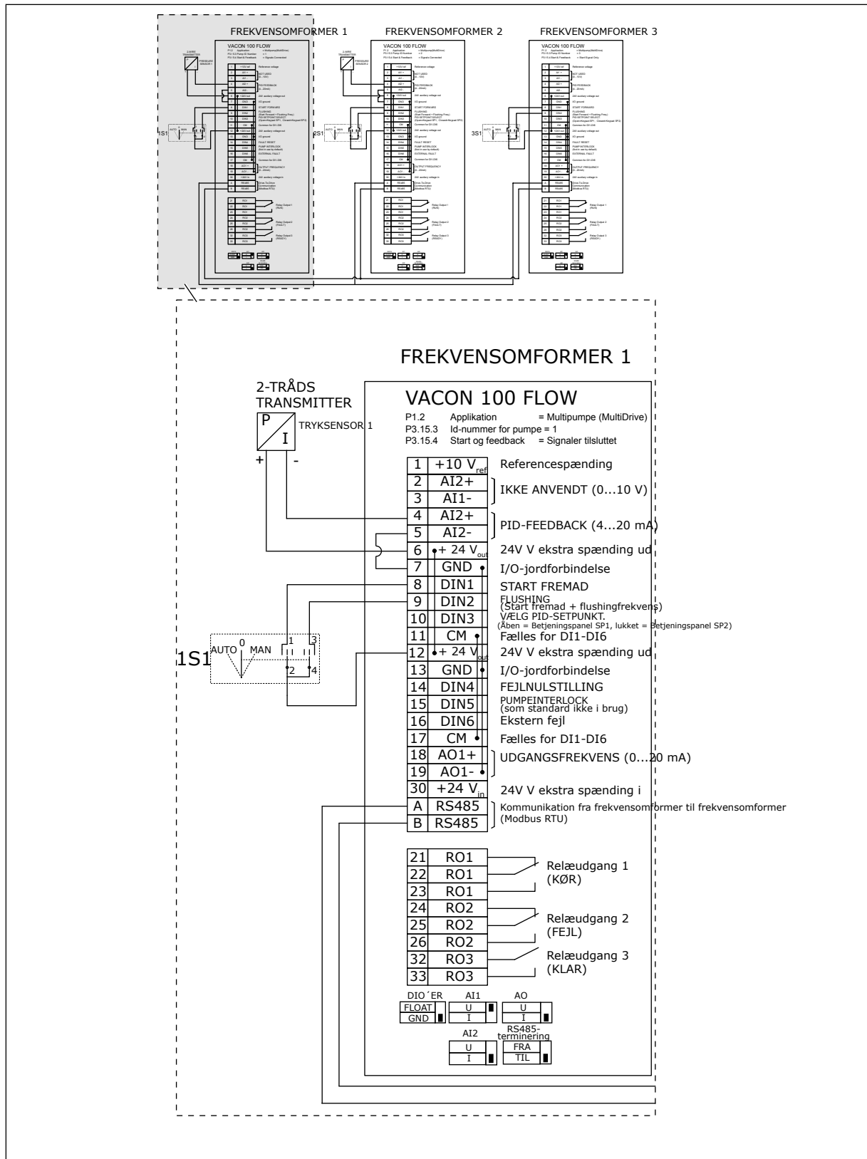
Fig. 24: Elektrisk koblings-skjema for multipumpesystem (flere omformere), eksempel 3 A
