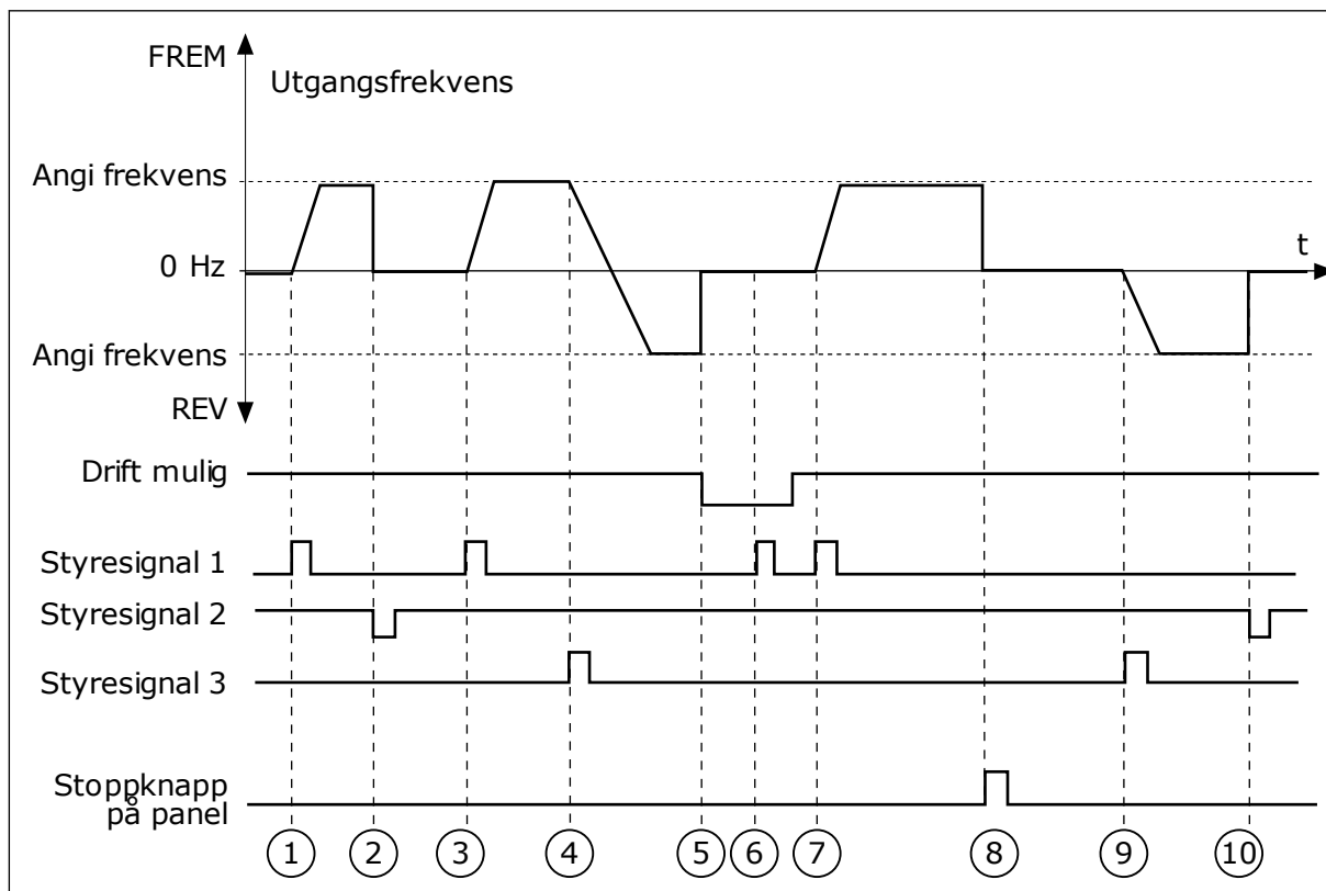
Fig. 43: Start-/Stopplogikk for I/O A = 1
