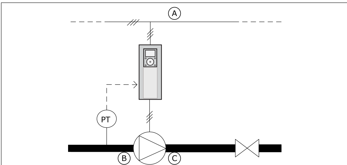
Rys. 86: Położenie czujnika ciśnienia
