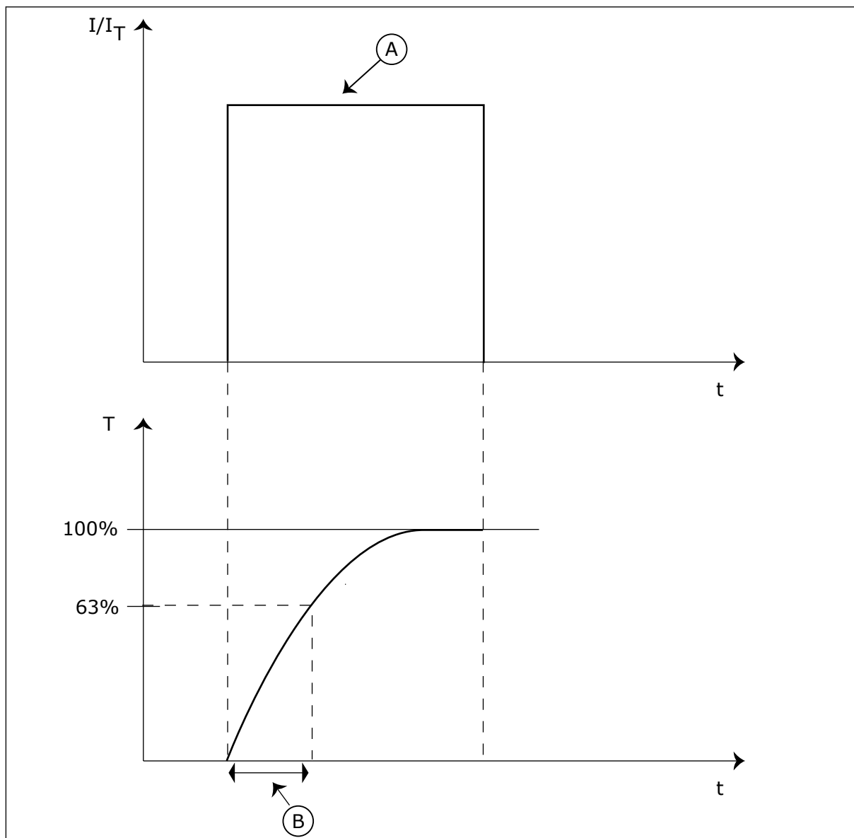
Fig. 66: Constanta temporală termică a motorului
