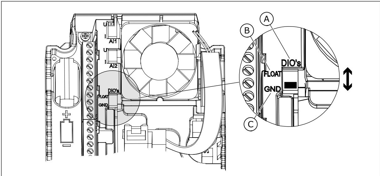
Fig. 7: Comutatorul DIP
