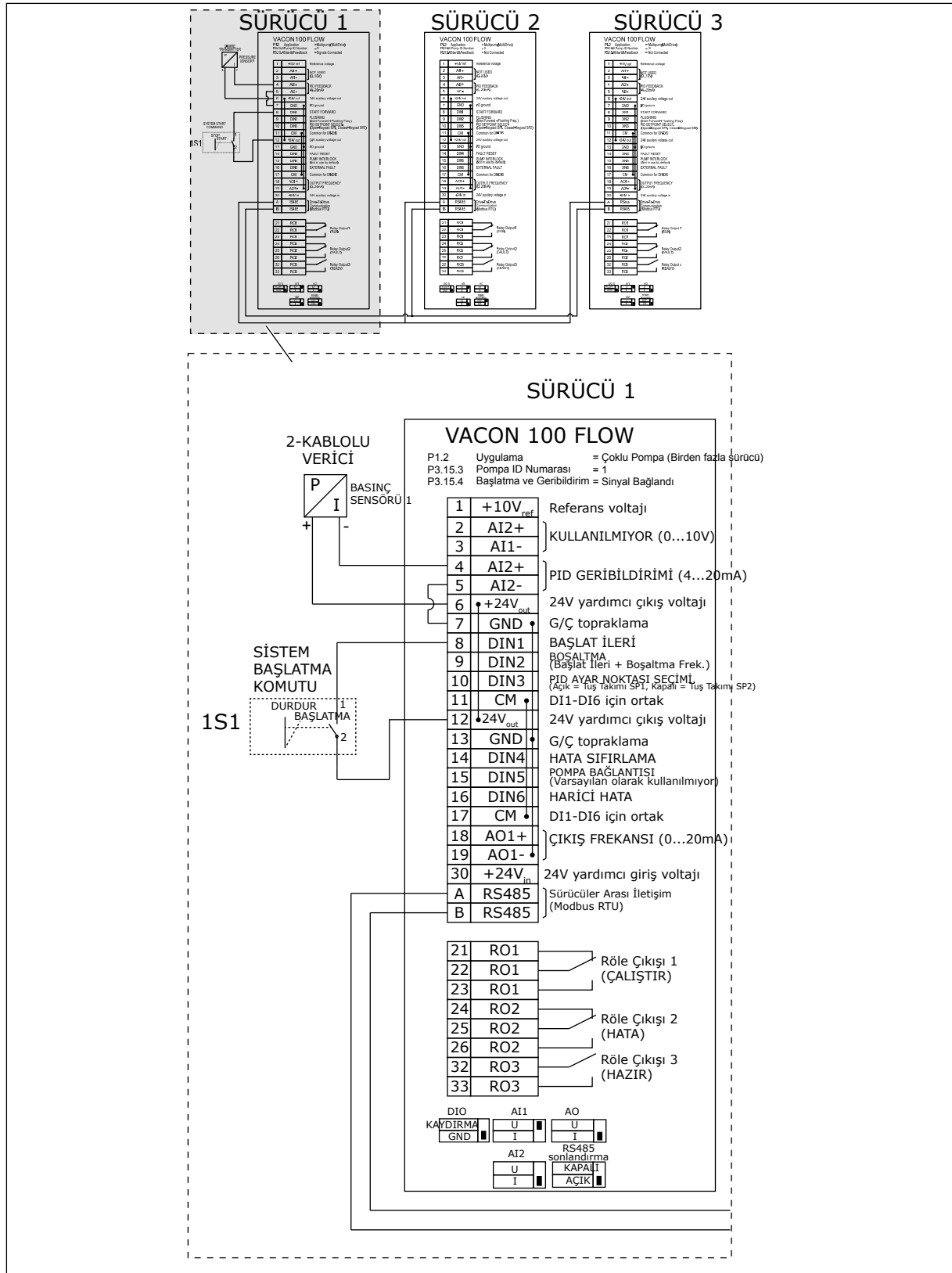
Şekil 30: Çoklu Pompa (çoklu sürücü) sisteminin elektrik kablo tesisatı şeması, örnek 5A
