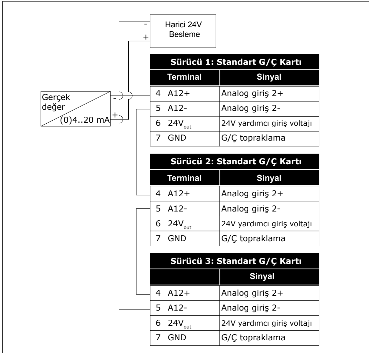
Şekil 96: Tüm sürücüler için aynı sensörün kablo tesisatı (harici 24 V kaynaktan beslenen)
