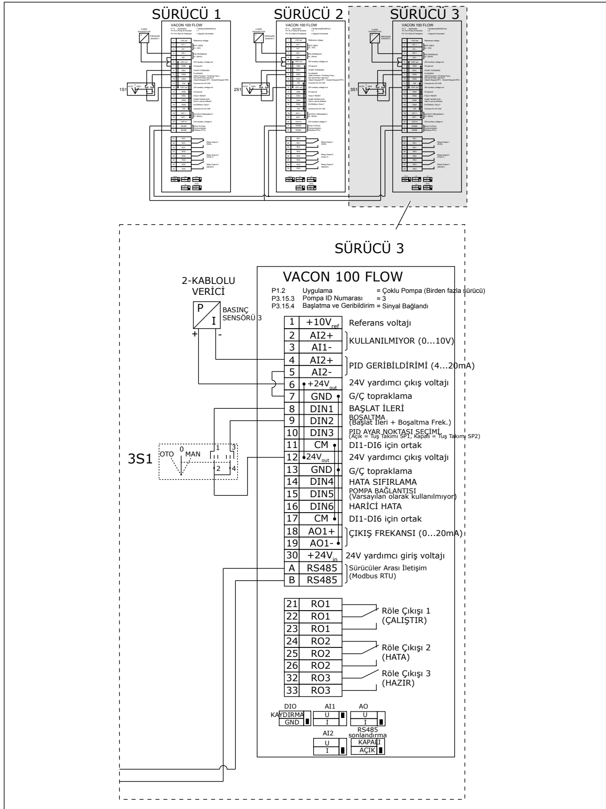
Şekil 20: Çoklu Pompa (çoklu sürücü) sisteminin elektrik kablo tesisatı şeması, örnek 1C
