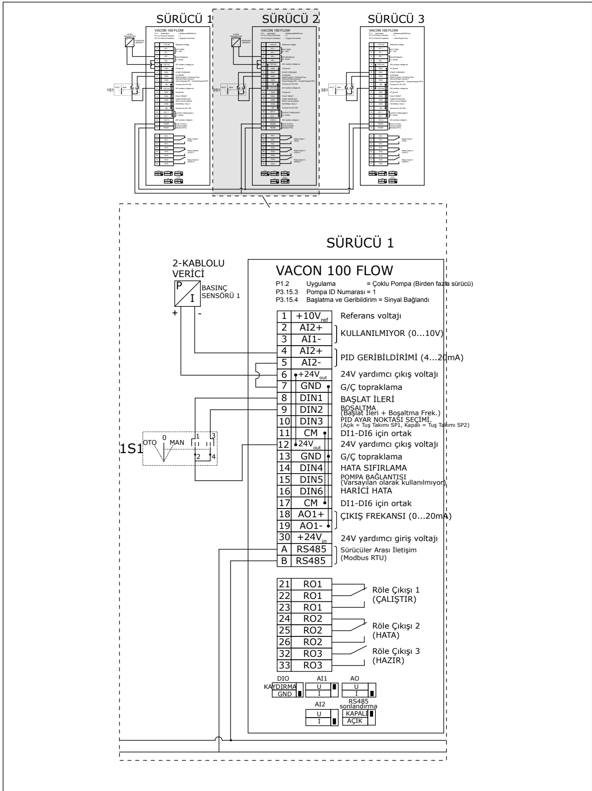
Şekil 25: Çoklu Pompa (çoklu sürücü) sisteminin elektrik kablo tesisatı şeması, örnek 3B
