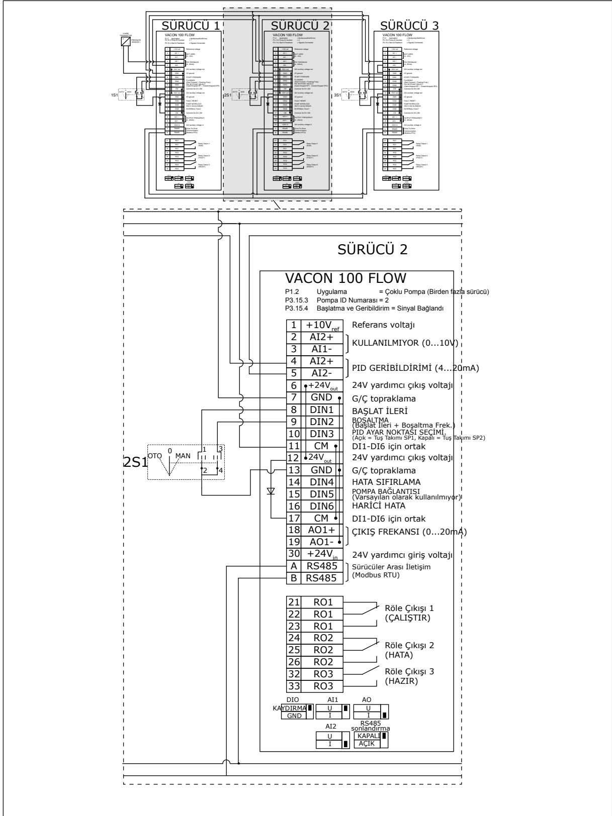
Şekil 22: Çoklu Pompa (çoklu sürücü) sisteminin elektrik kablo tesisatı şeması, örnek 2B
