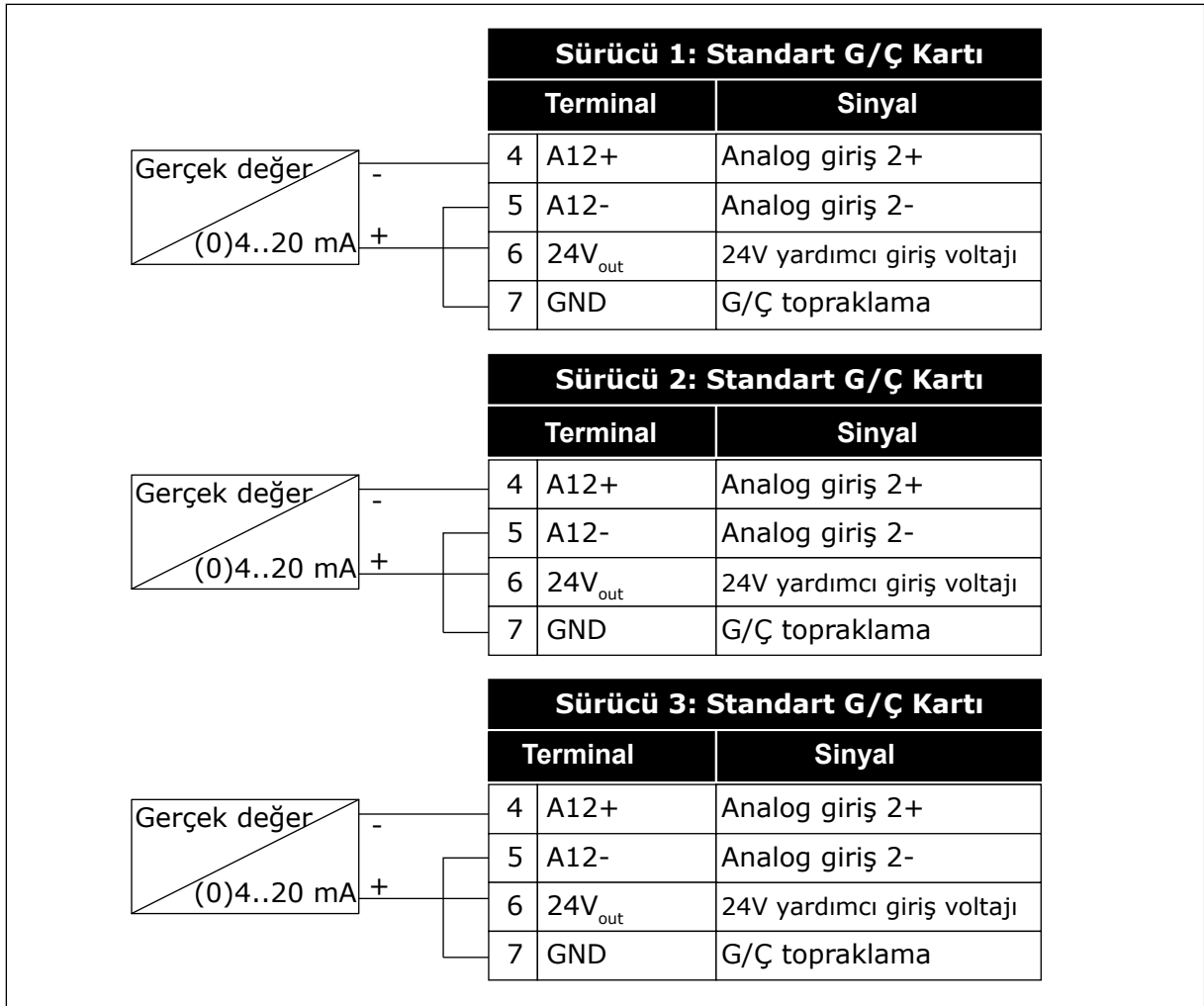
Şekil 94: Her sürücü için geribildirim sensörü kablo tesisatı
