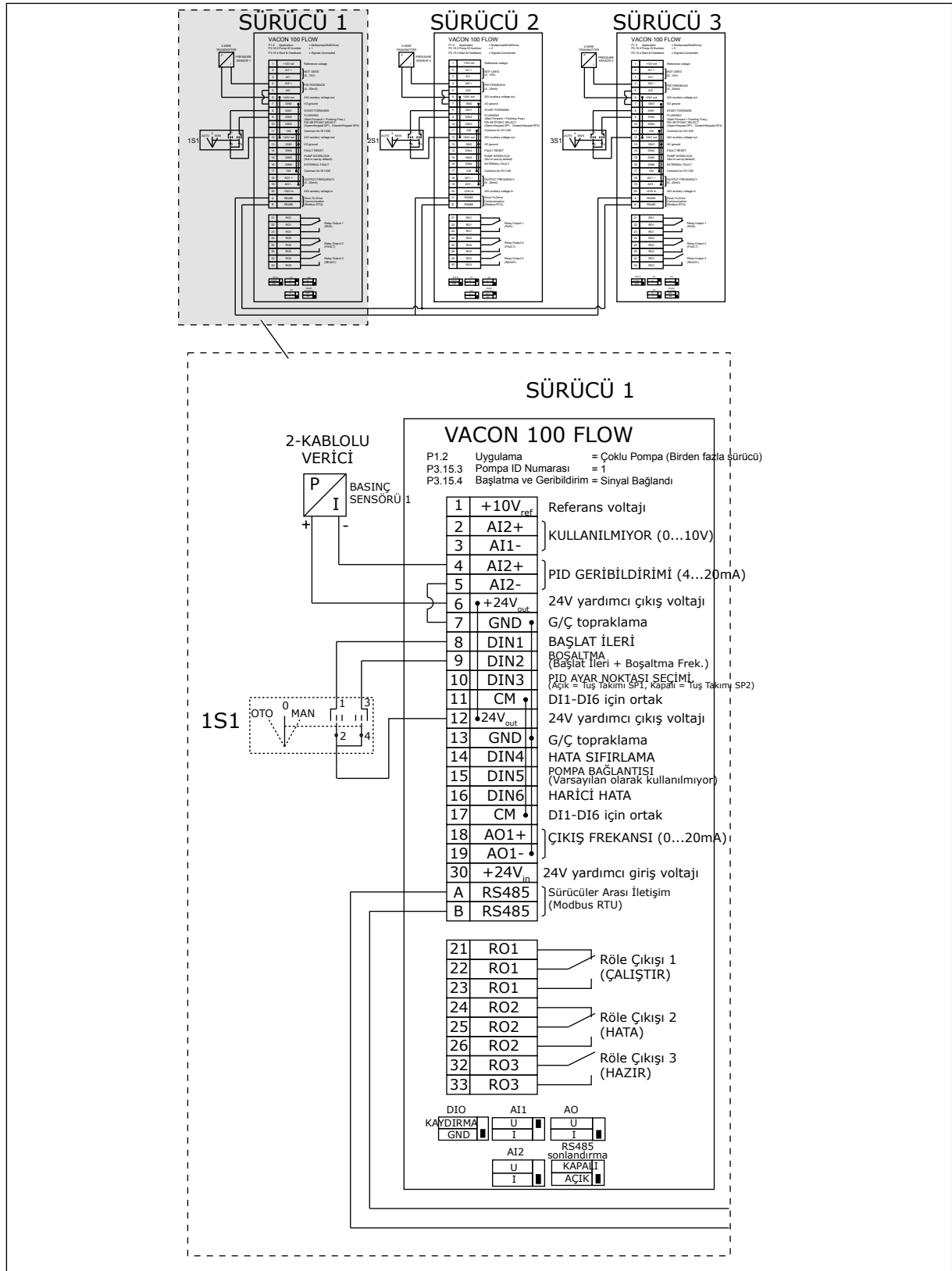
Şekil 18: Çoklu Pompa (çoklu sürücü) sisteminin elektrik kablo tesisatı şeması, örnek 1A
