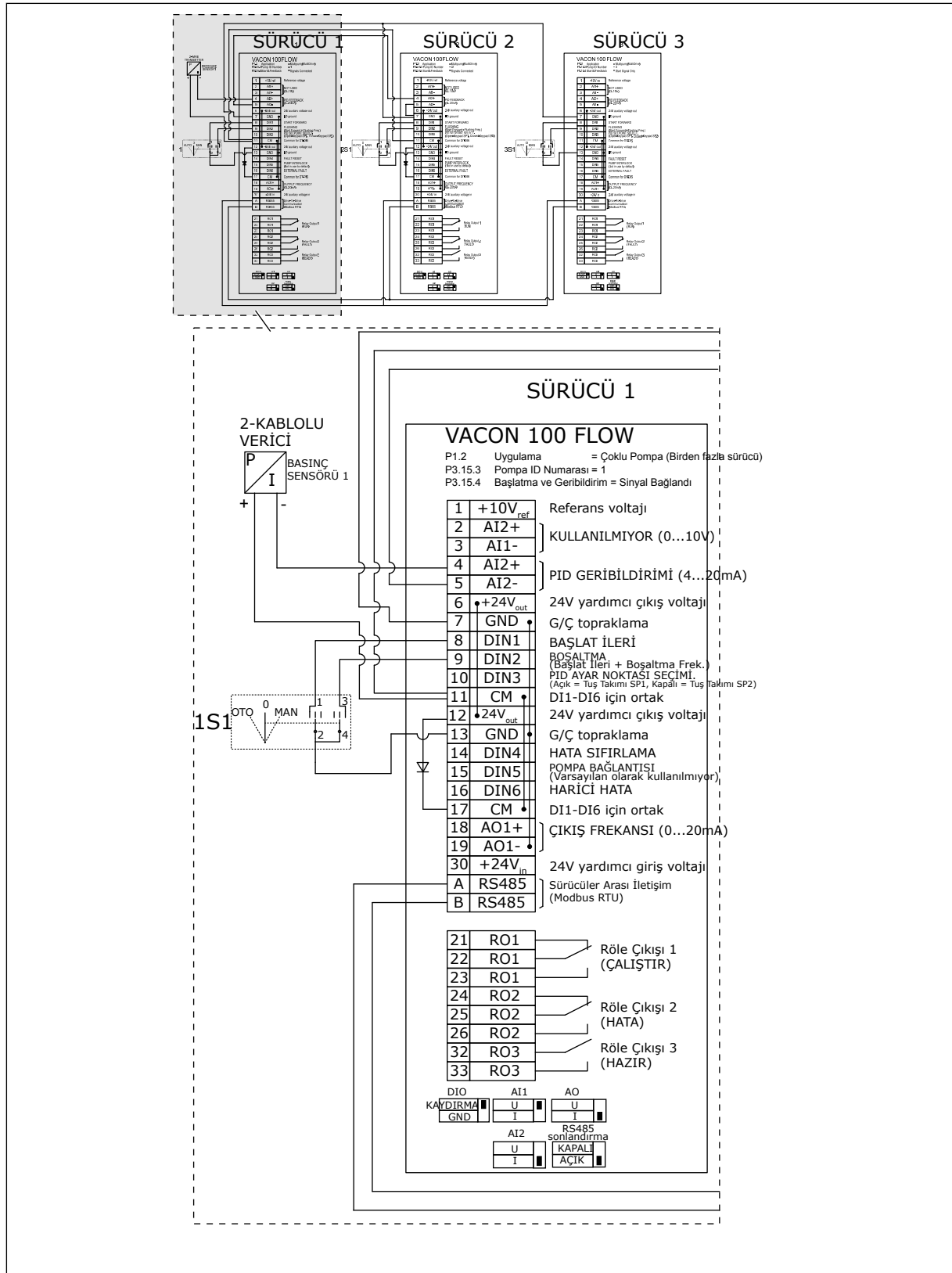
Şekil 27: Çoklu Pompa (çoklu sürücü) sisteminin elektrik kablo tesisatı şeması, örnek 4A
