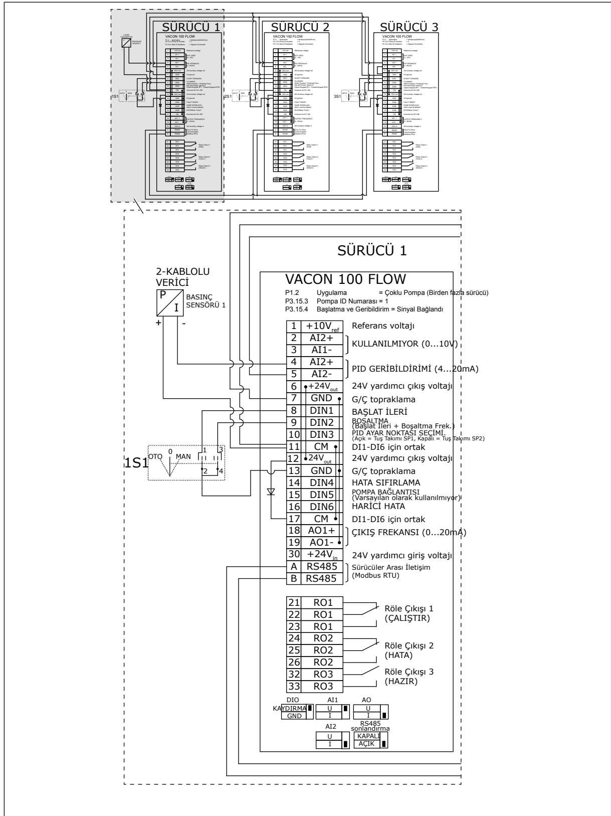
Şekil 21: Çoklu Pompa (çoklu sürücü) sisteminin elektrik kablo tesisatı şeması, örnek 2A
