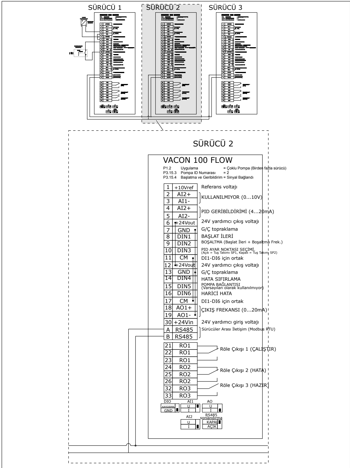
Şekil 31: Çoklu Pompa (çoklu sürücü) sisteminin elektrik kablo tesisatı şeması, örnek 5B
