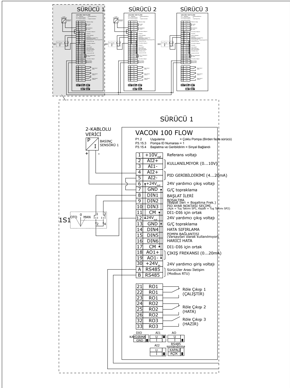
Şekil 24: Çoklu Pompa (çoklu sürücü) sisteminin elektrik kablo tesisatı şeması, örnek 3A
