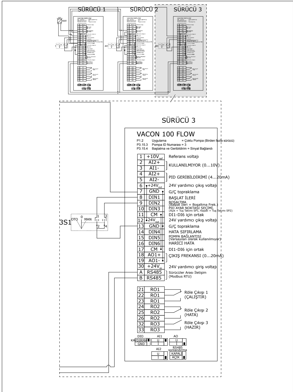
Şekil 29: Çoklu Pompa (çoklu sürücü) sisteminin elektrik kablo tesisatı şeması, örnek 4C
