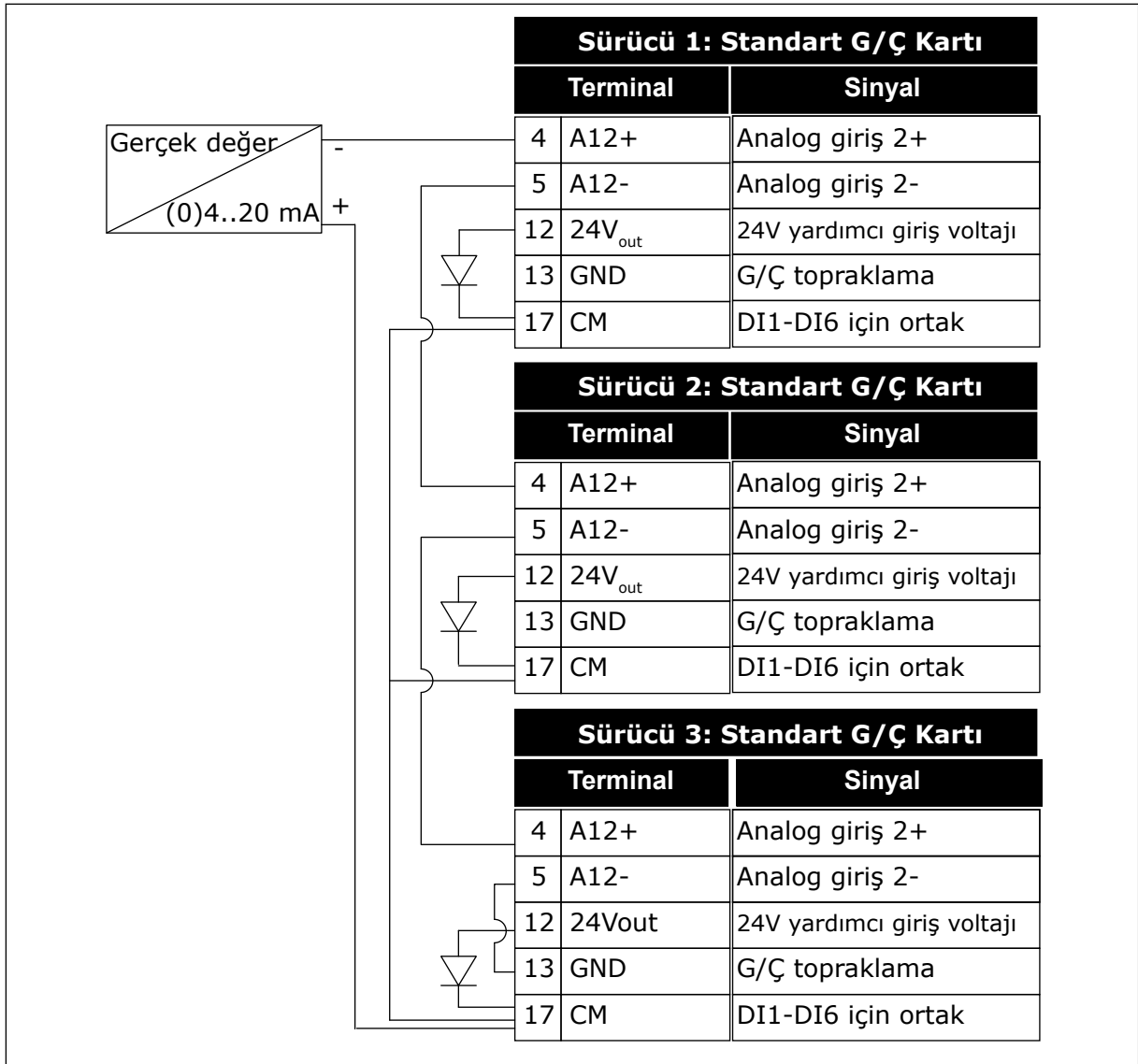
Şekil 95: Tüm sürücüler için aynı sensörün kablo tesisatı (sürücü G/Ç kartından sağlanan)
