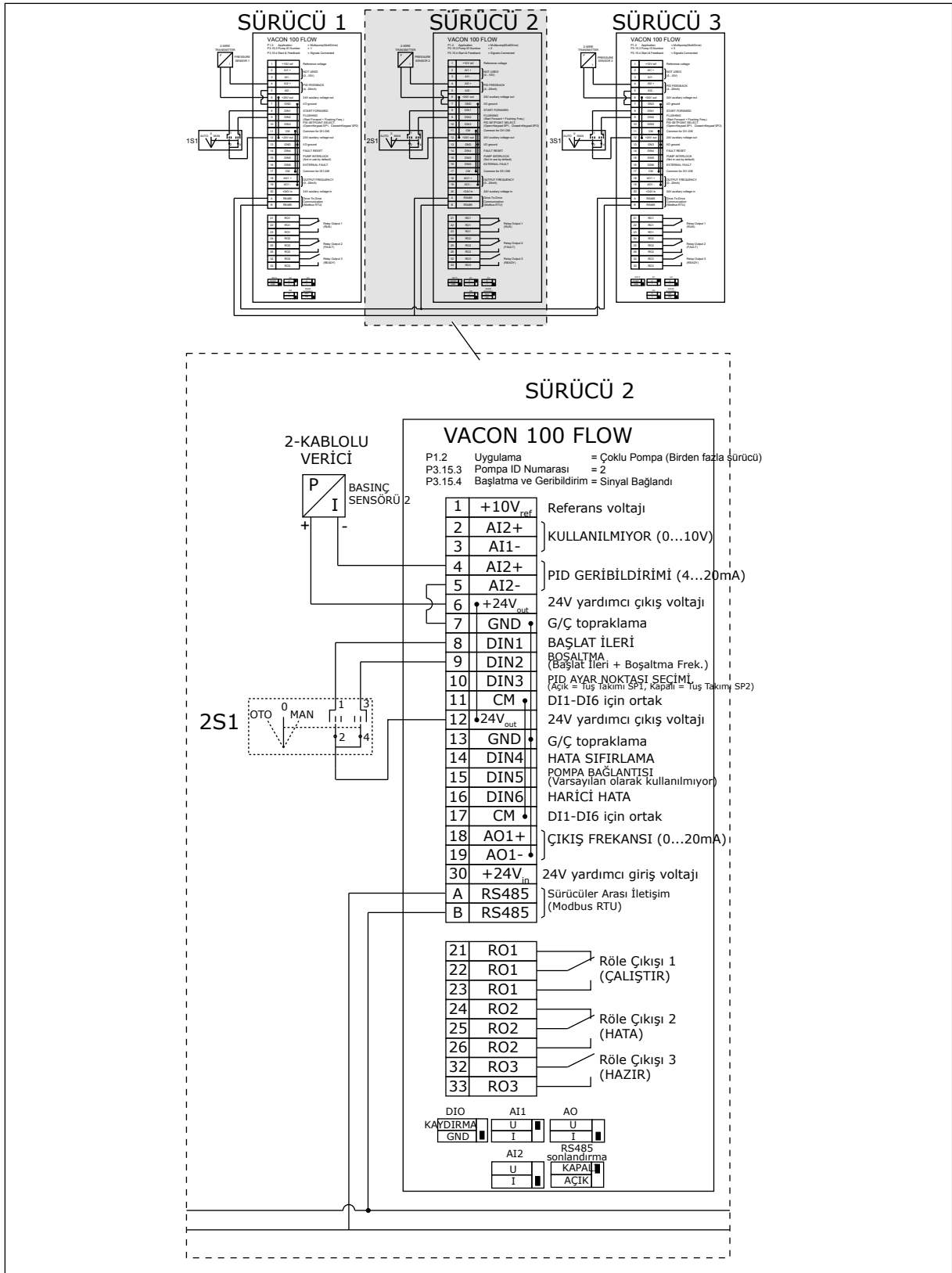
Şekil 19: Çoklu Pompa (çoklu sürücü) sisteminin elektrik kablo tesisatı şeması, örnek 1B
