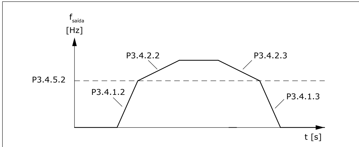
Fig. 50: Ativação da rampa 2 quando a frequência de saída exceder o nível do limiar. (P.3.4.5.2 = Limiar de frequência da rampa, P3.4.1.2 = Tempo de aceleração 1, P3.4.2.2 = Tempo de aceleração 2, P3.4.1.3 = Tempo de desaceleração 1, P3.4.2.3 = Tempo de desaceleração 2)
