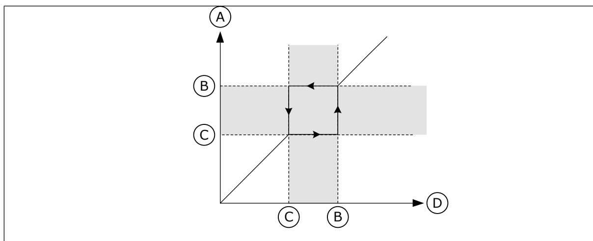
Fig. 63: As frequências proibidas
