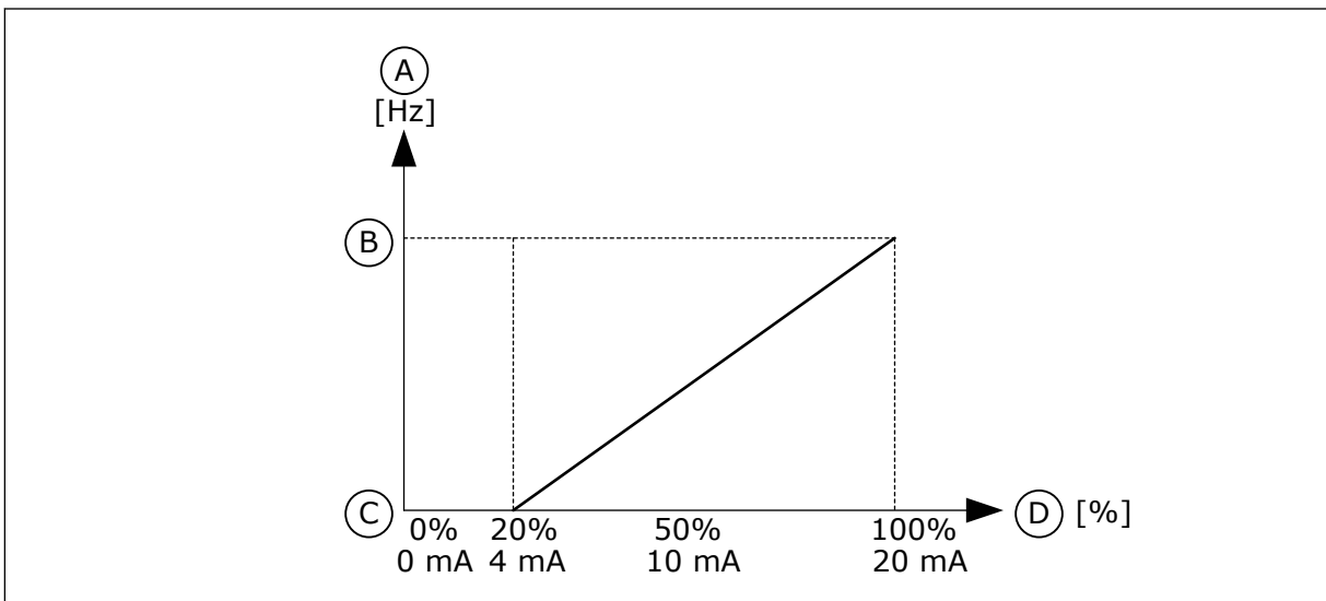
Fig. 58: A faixa de sinal da entrada analógico, seleção '1'
