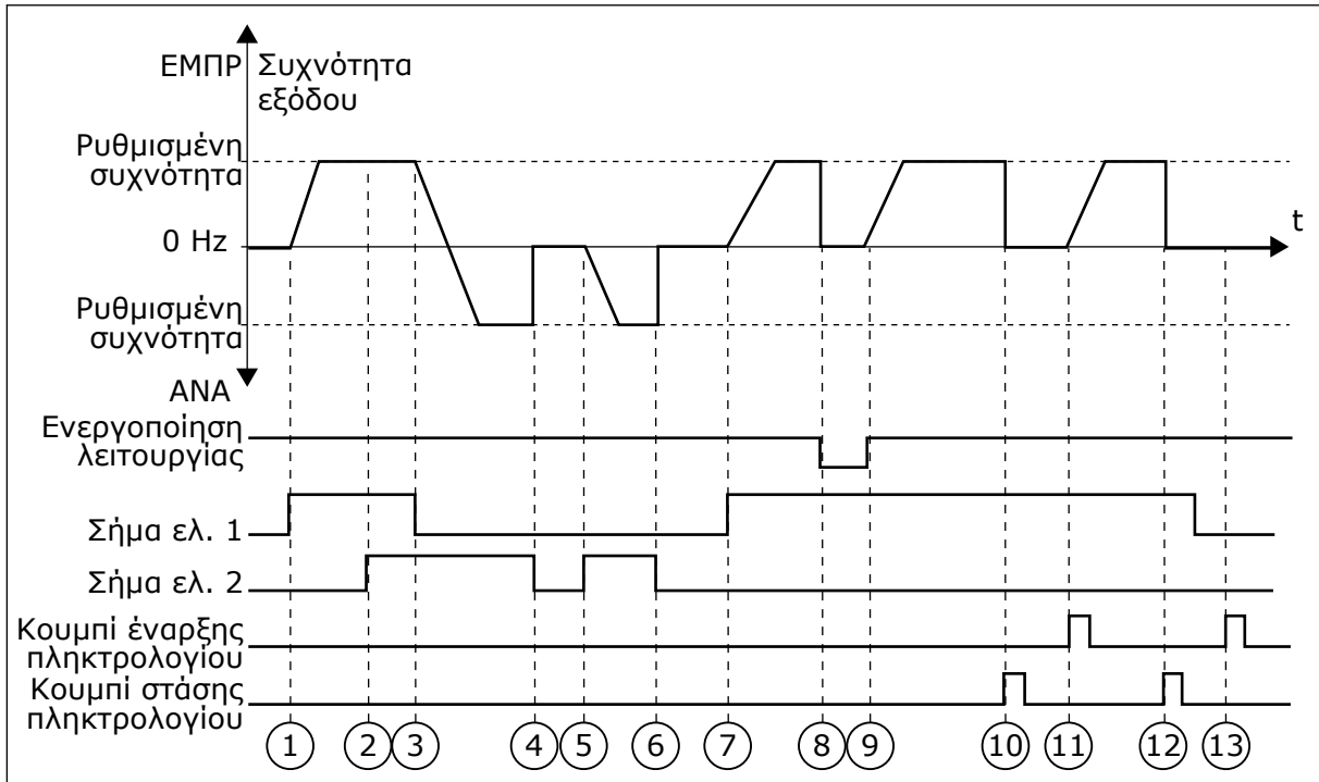
Σχ. 42: Λογική έναρξης/στάσης / O A = 0
