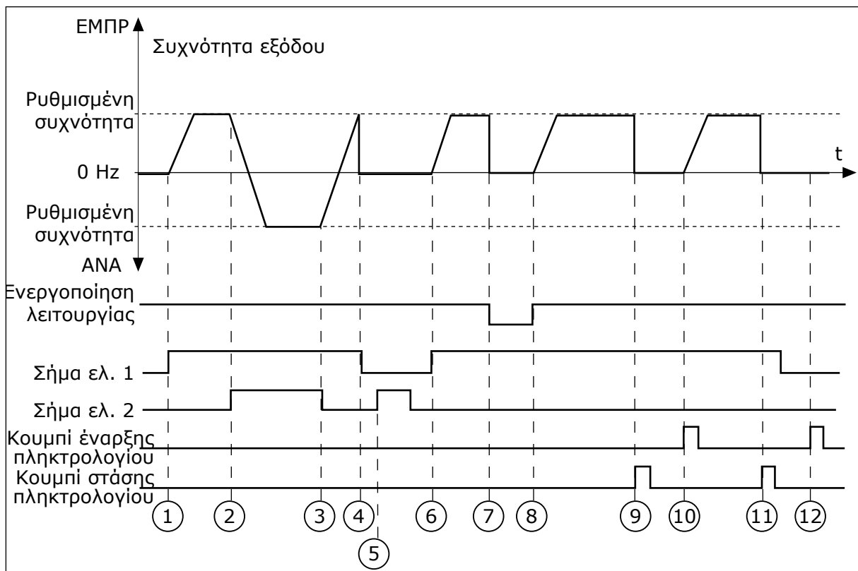
Σχ. 45: Λογική έναρξης/στάσης / O A = 3
