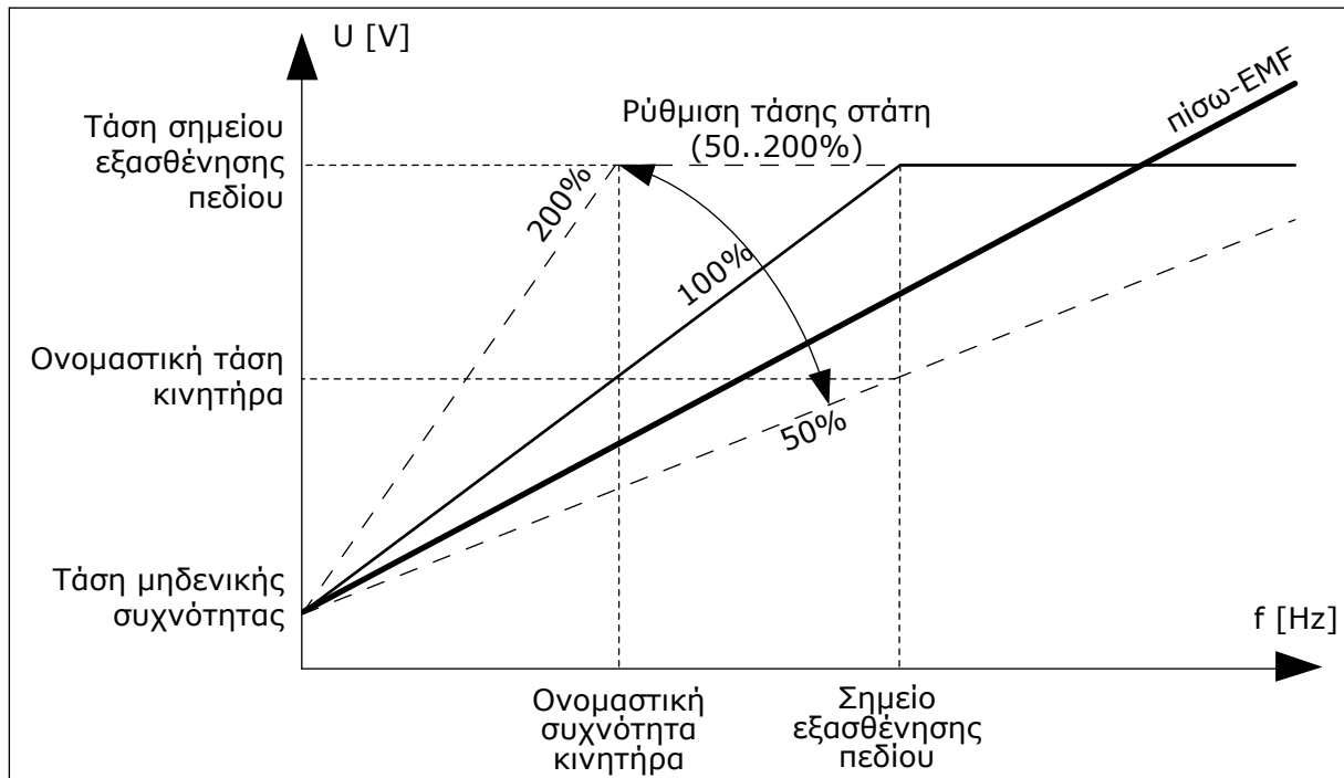
Σχ. 37: Ρύθμιση τάσης στάση
