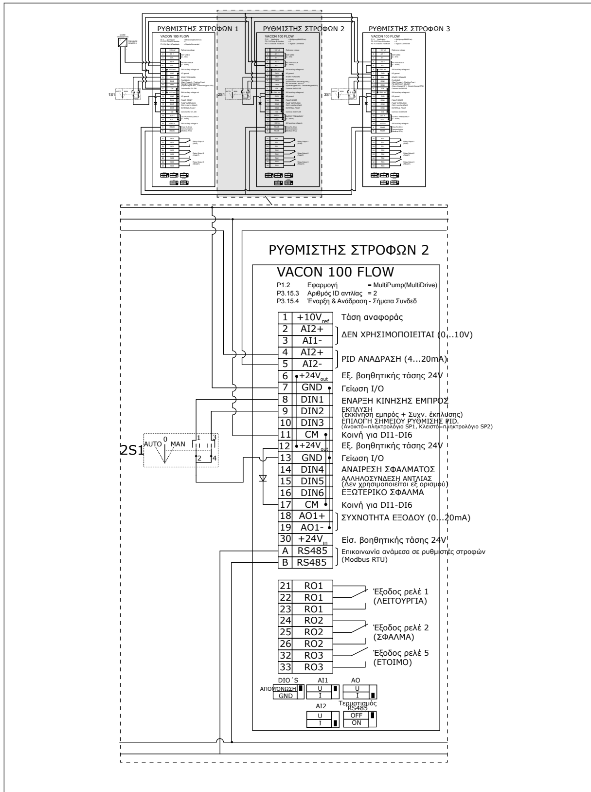
Σχ. 22: Διάγραμμα συνδεσμολογίας του συστήματος πολλαπλών αντλιών (πολλαπλοί ρυθμιζόμενες στροφών), παράδειγμα 2B
