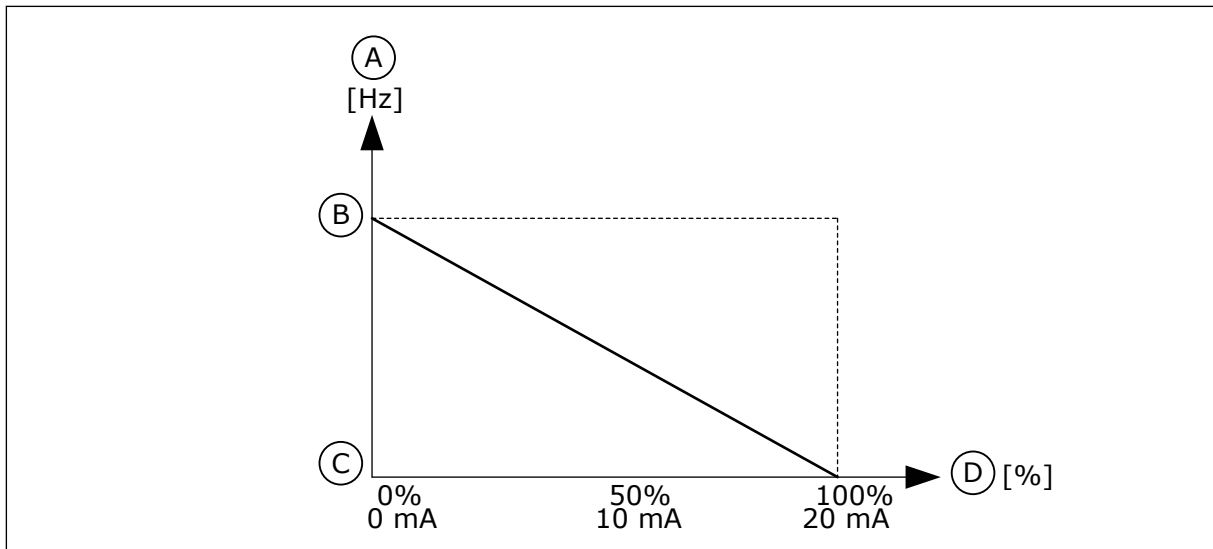
Σχ. 61: Αναστροφή σήματος AI1, επιλογή 1
