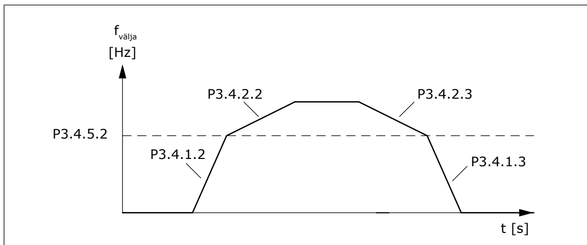
Fig. 50: Rambi 2 aktiveerimine, kui väljundsagedus tõuseb üle läve taseme. (P3.4.5.2 = rambi läve sagedus, P3.4.1.2 = kiirendusaeg 1, P3.4.2.2 = kiirendusaeg 2, P3.4.1.3 = aeglustusaeg 1, P3.4.2.3 = aeglustusaeg 2)
