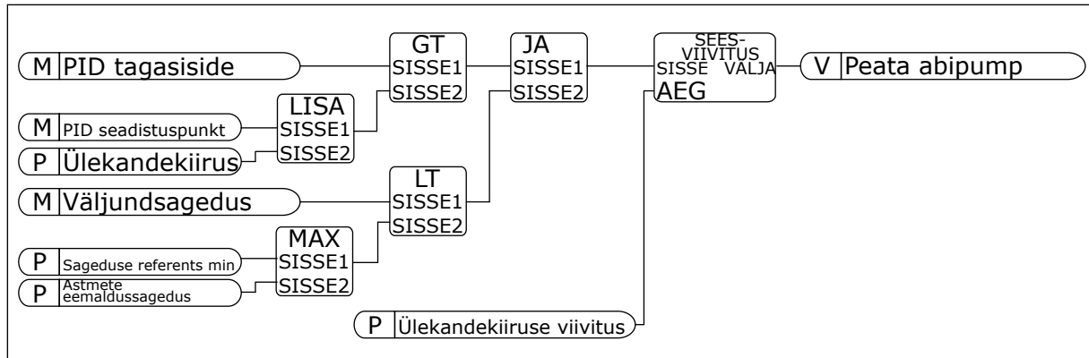
Fig. 102: Astmete eemaldussagedus
