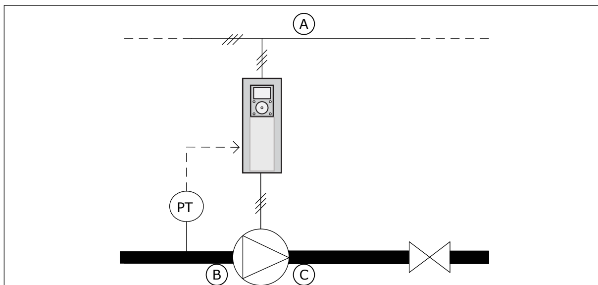
Fig. 86: Rõhuanduri asukoht
