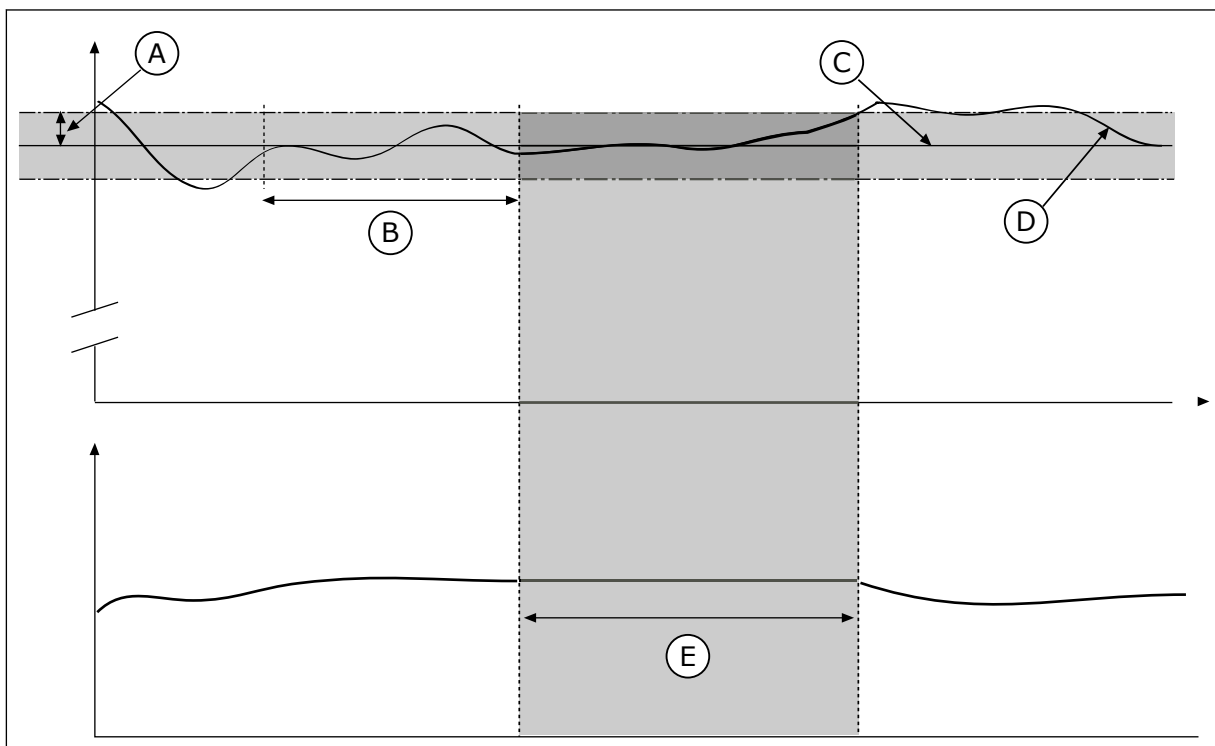
Fig. 79: Määramatuspiirkonna funktsioon
