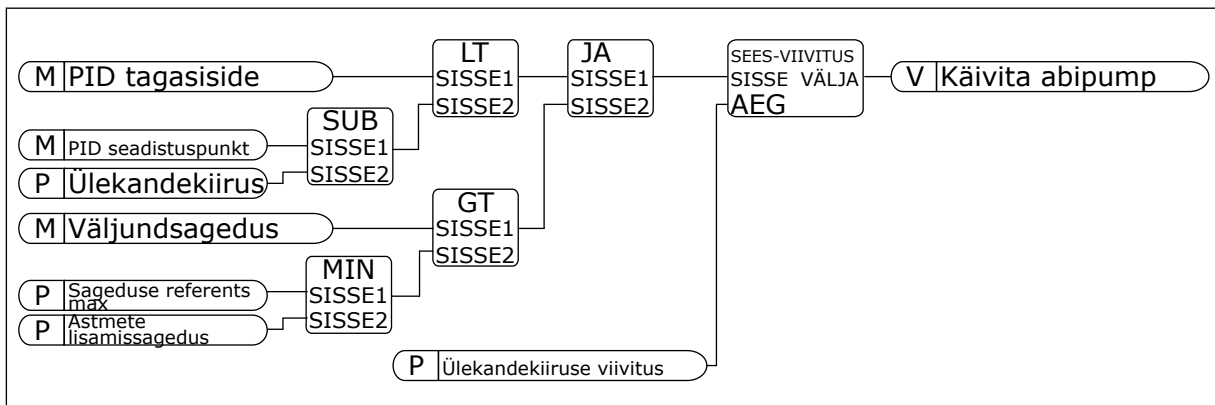
Fig. 101: Astmete lisamissagedus
