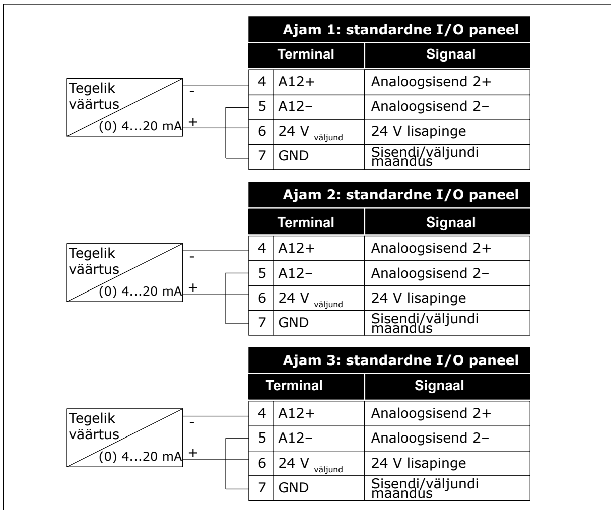
Fig. 94: Iga ajami tagasiside anduri juhtmestus
