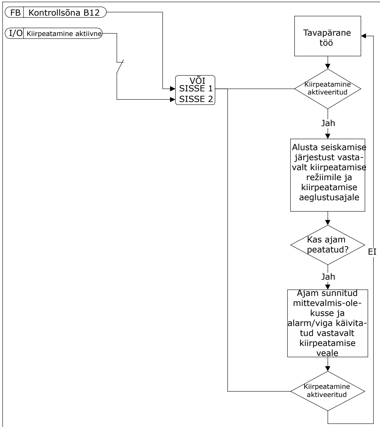
Fig. 71: Kiirpeatamise loogika
