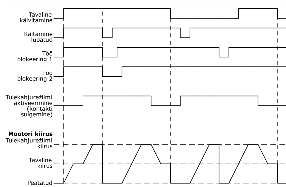
Fig. 103: Tulekahjurežiimi funktsioon
