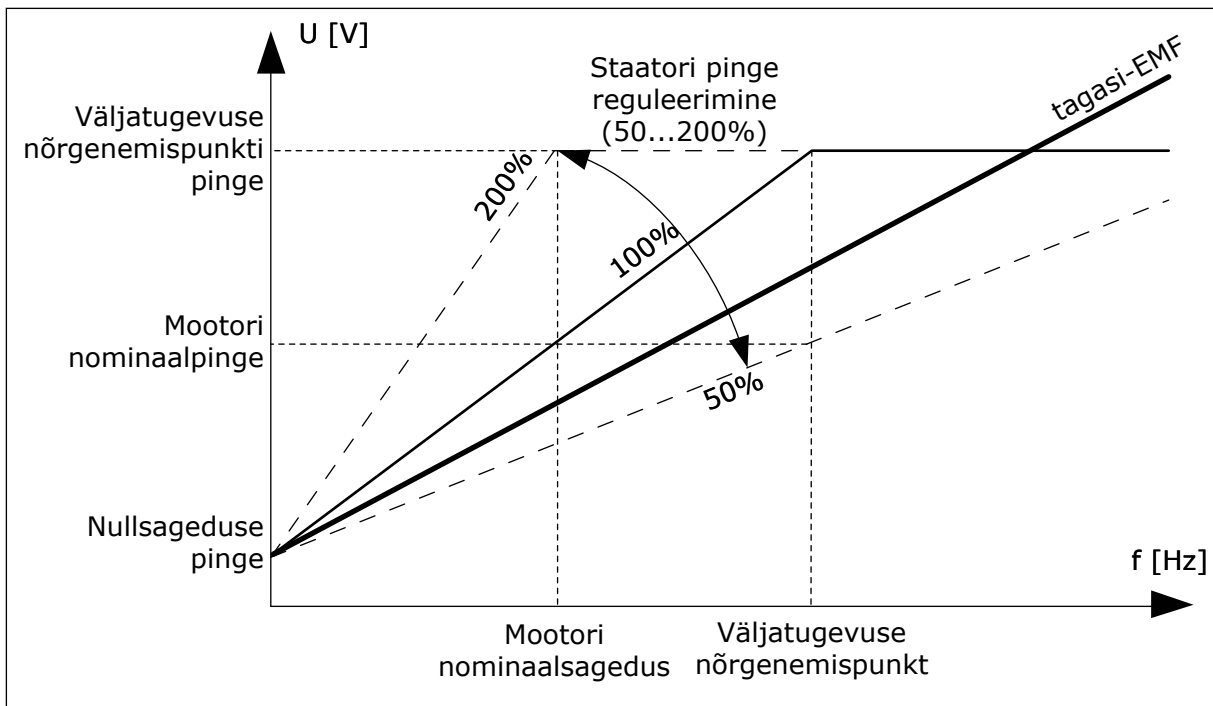
Fig. 37: Staatore pingeregulatsioon
