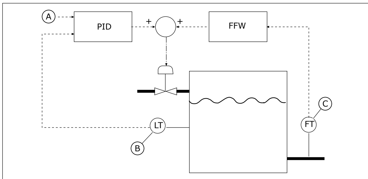
Fig. 80: Edasisöötmise juhtimine
