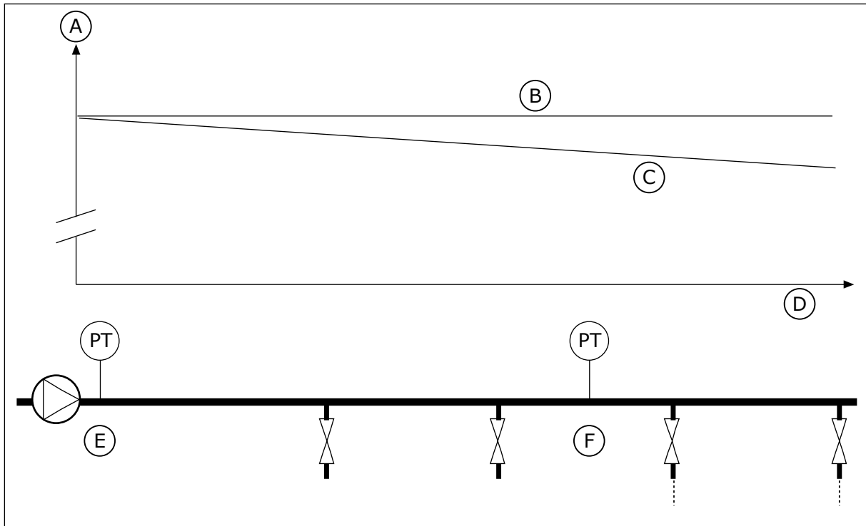
Att. 84: Spiediena sensora pozīcija
