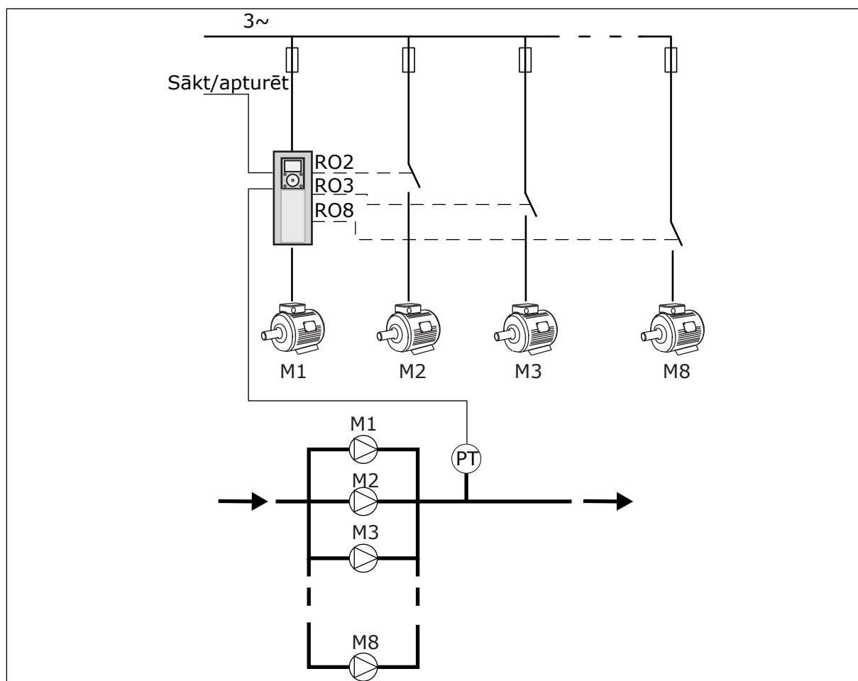
Att. 89: Viena pārveidotāja konfigurācija (PT = spiediena sensors)
