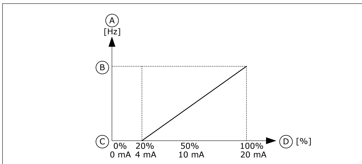
Att. 58: Analogās ievades signāla diapazons, atlase 1
