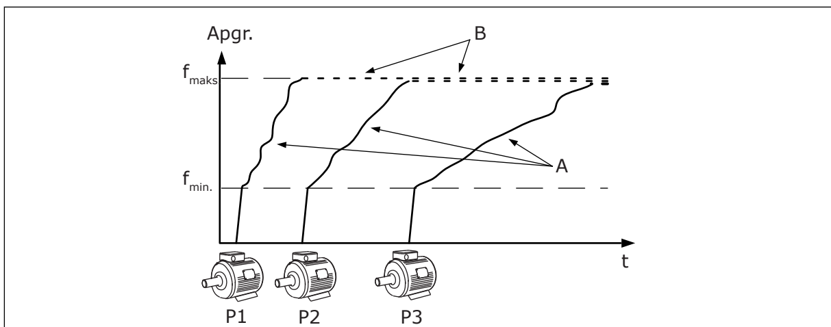
Att. 93: Vadība multivedēja režīmā
