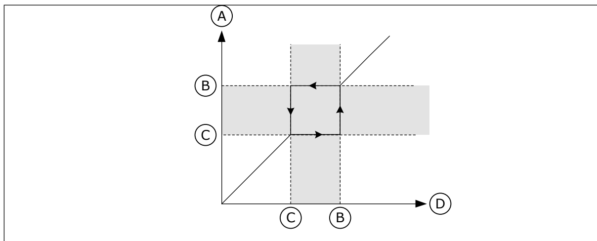
Att. 63: Aizliegtās frekvences
