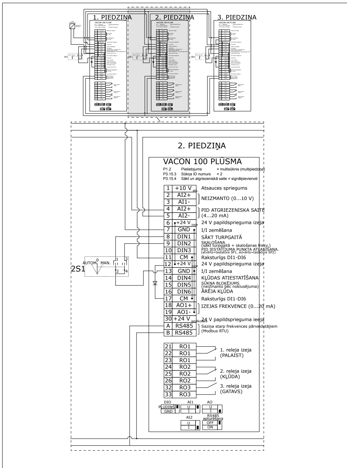
Att. 22: Multisūkņa (multipārveidotāja) sistēmas elektromontāžas shēma, piemērs 2B
