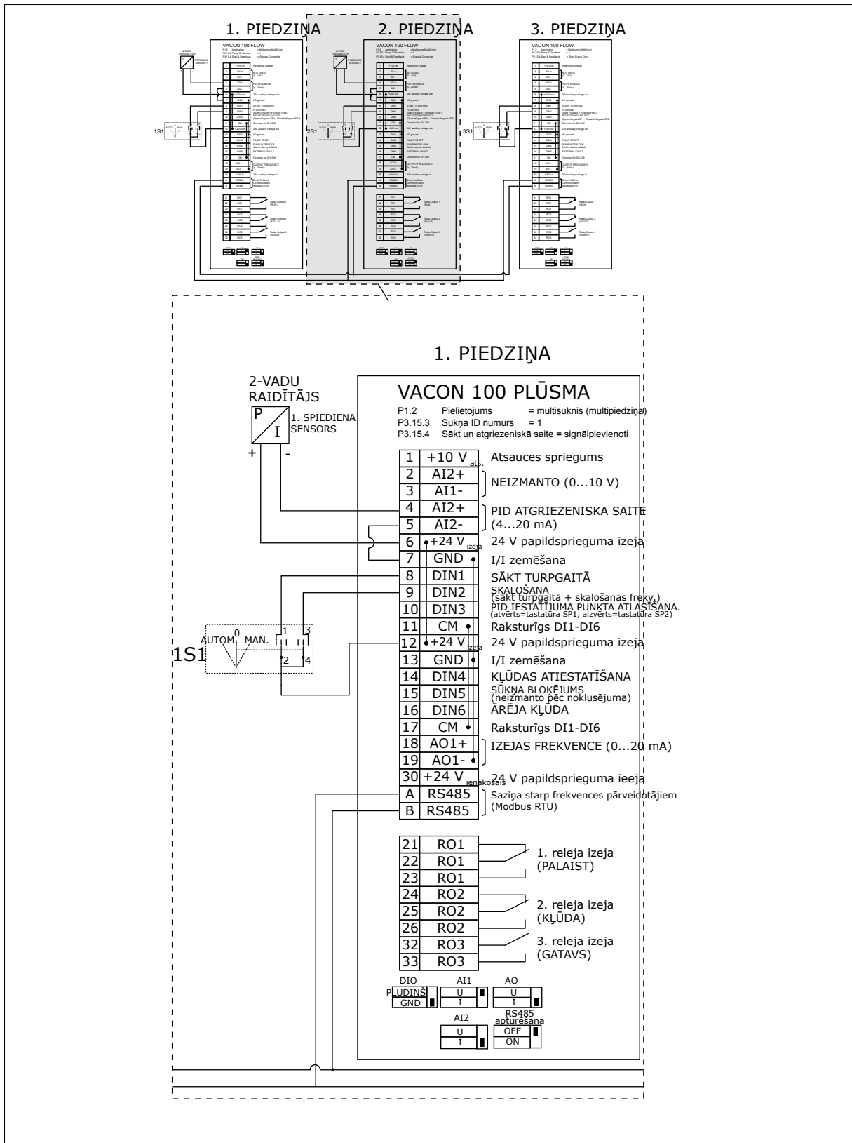
Att. 25: Multisūkņa (multipārveidotāja) sistēmas elektromontāžas shēma, piemērs 3B
