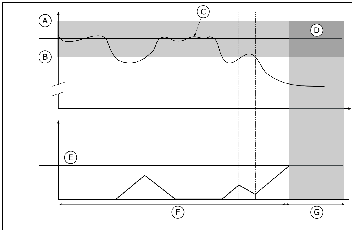
Att. 83: Atbildes pārraudzības funkcija
