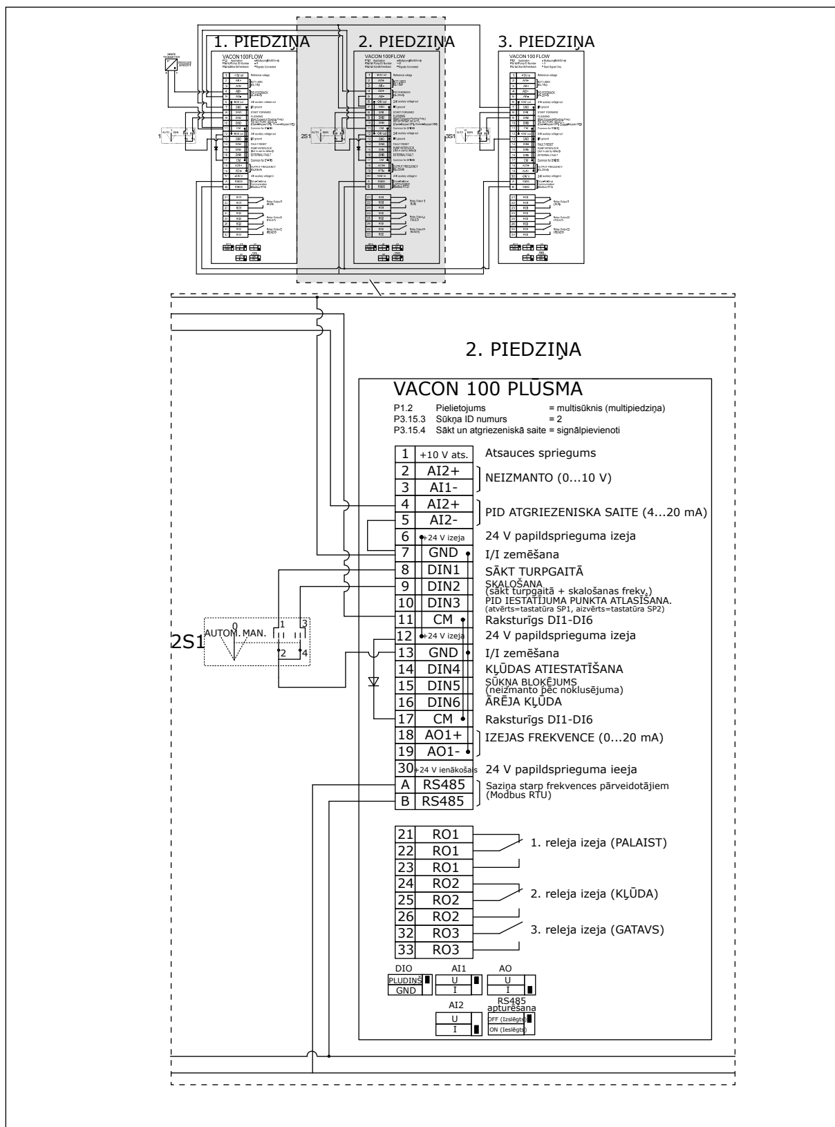
Att. 28: Multisūkņa (multipārveidotāja) sistēmas elektromontāžas shēma, piemērs 4B
