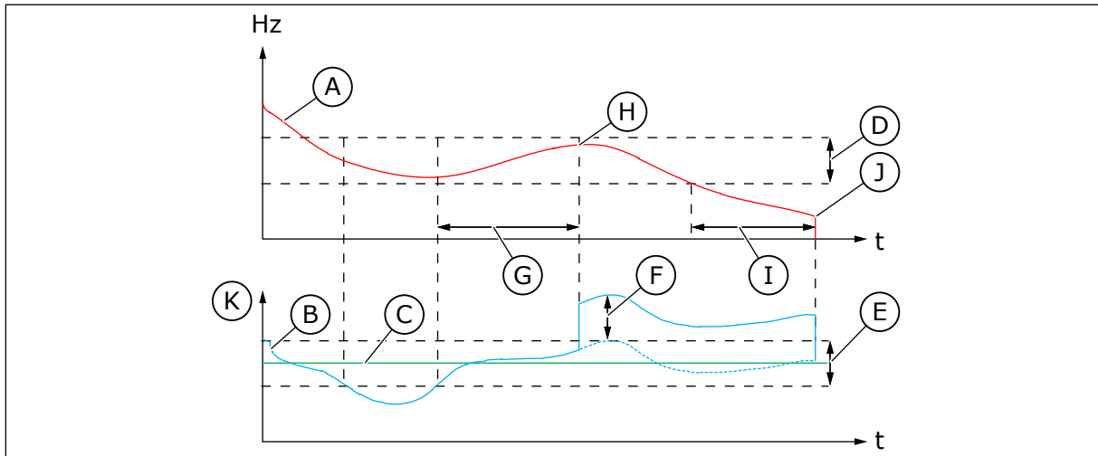
Att. 88: Miega režīms, nav konstatēts pieprasījums
