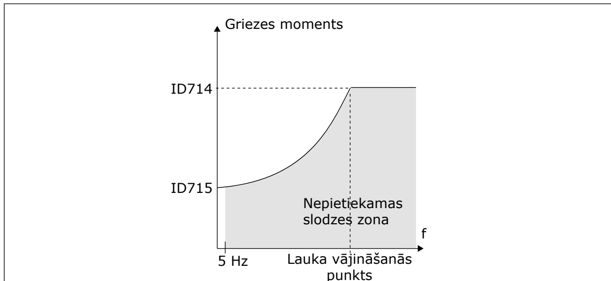
Att. 69: Minimālās slodzes iestatīšana
