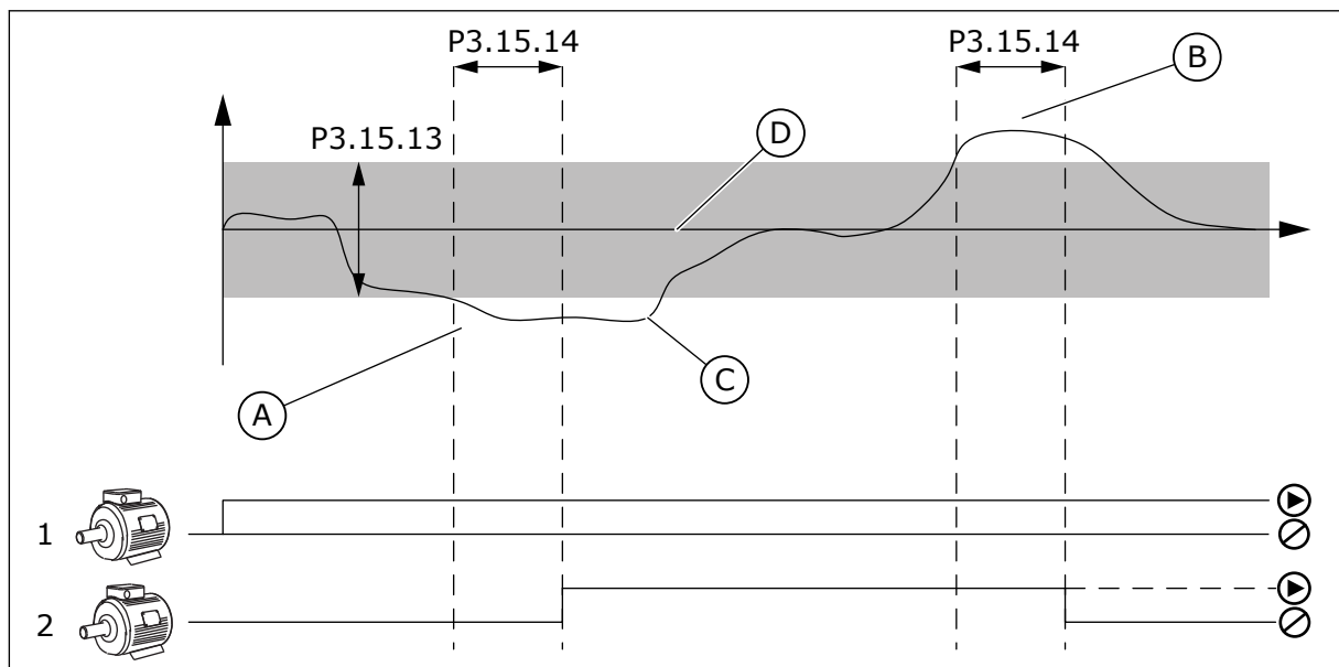
Att. 99: Papildu sūkņu sākšana vai apturēšana (P3.15.13 = joslas platums, P3.15.14 = joslas platuma aizkave)
