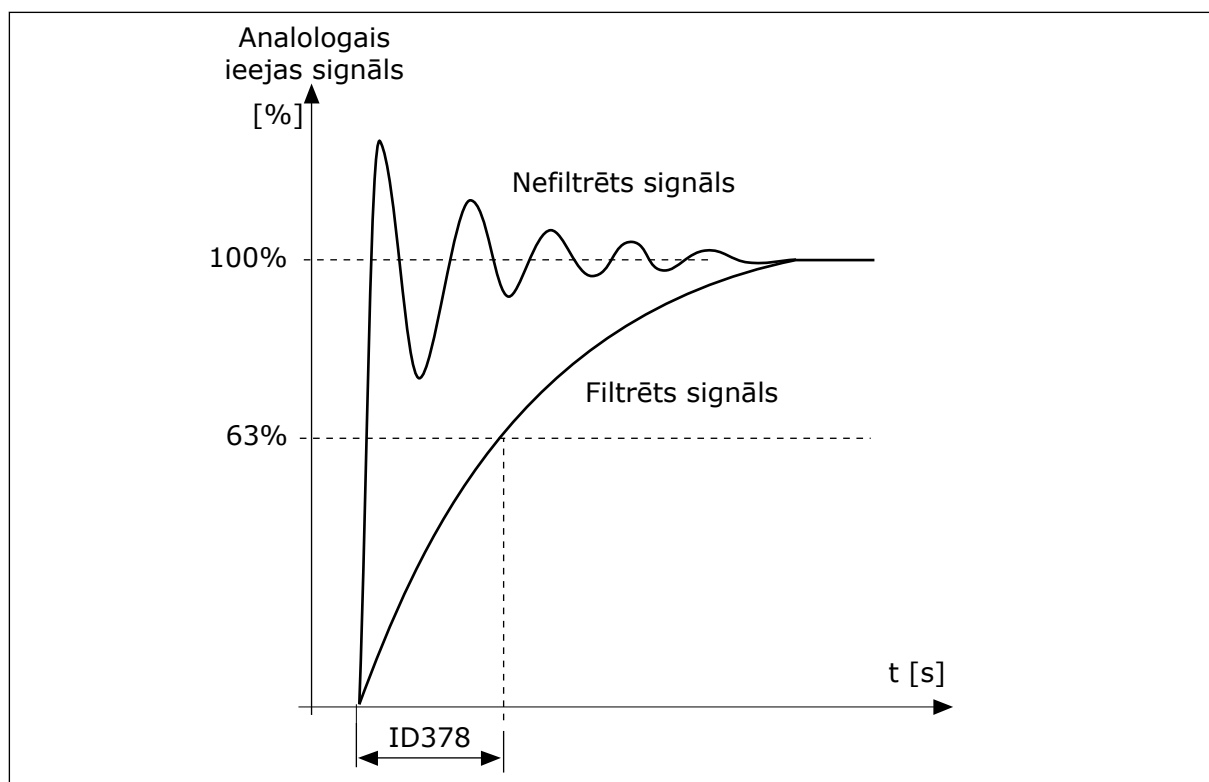
Att. 56: AI1 signāla filtrēšana
