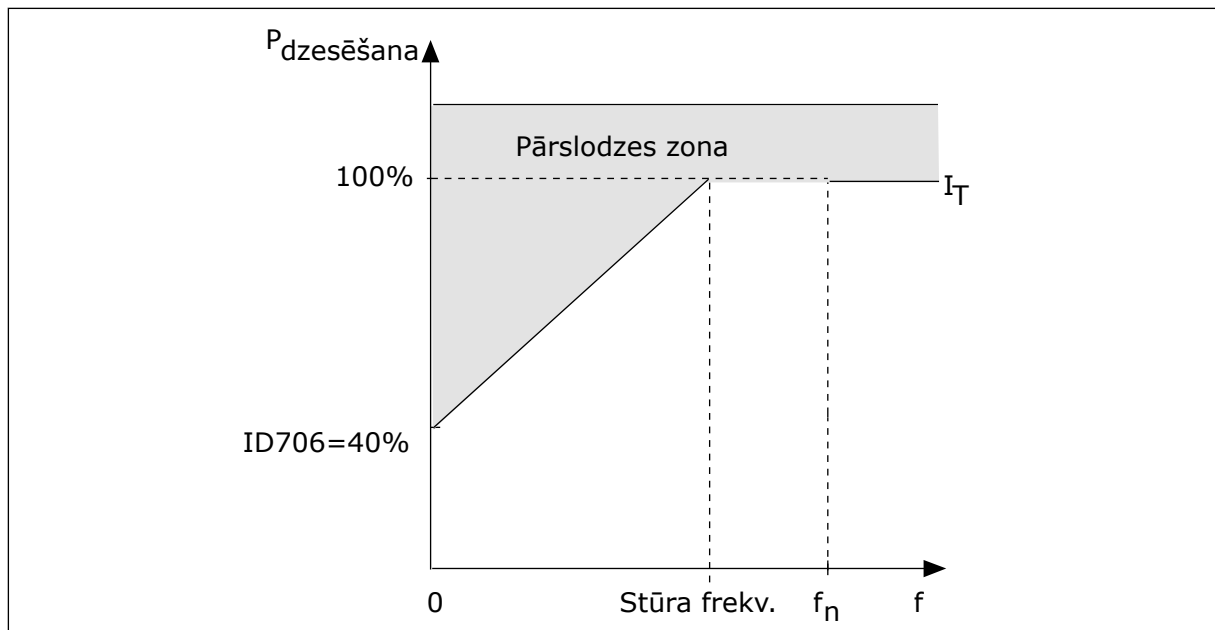
Att. 65: Elektrodzinēja siltuma strāvas I_T līkne
