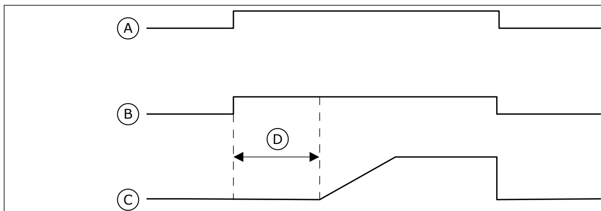
Att. 106: Uzpildīšanas sūkņa funkcija
