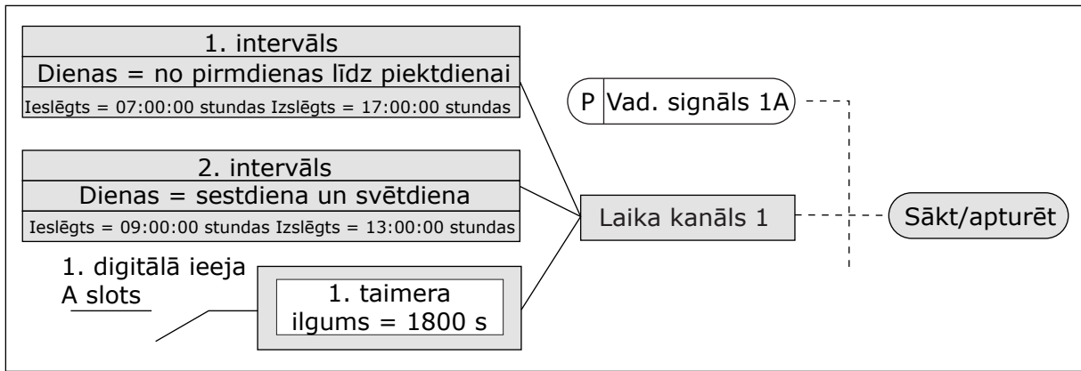
Att. 78: 1. laika kanālu izmanto kā sākšanas komandas vadības signālu digitālās ievades vietā
