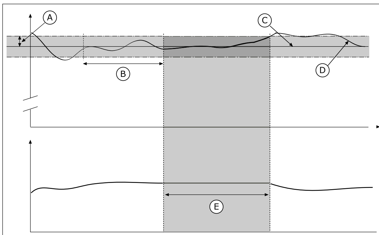
Att. 79: Nejūtības zonas funkcija
