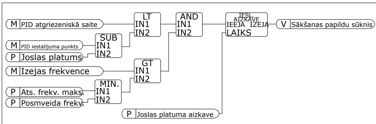
Att. 101: Posmveida frekvence
