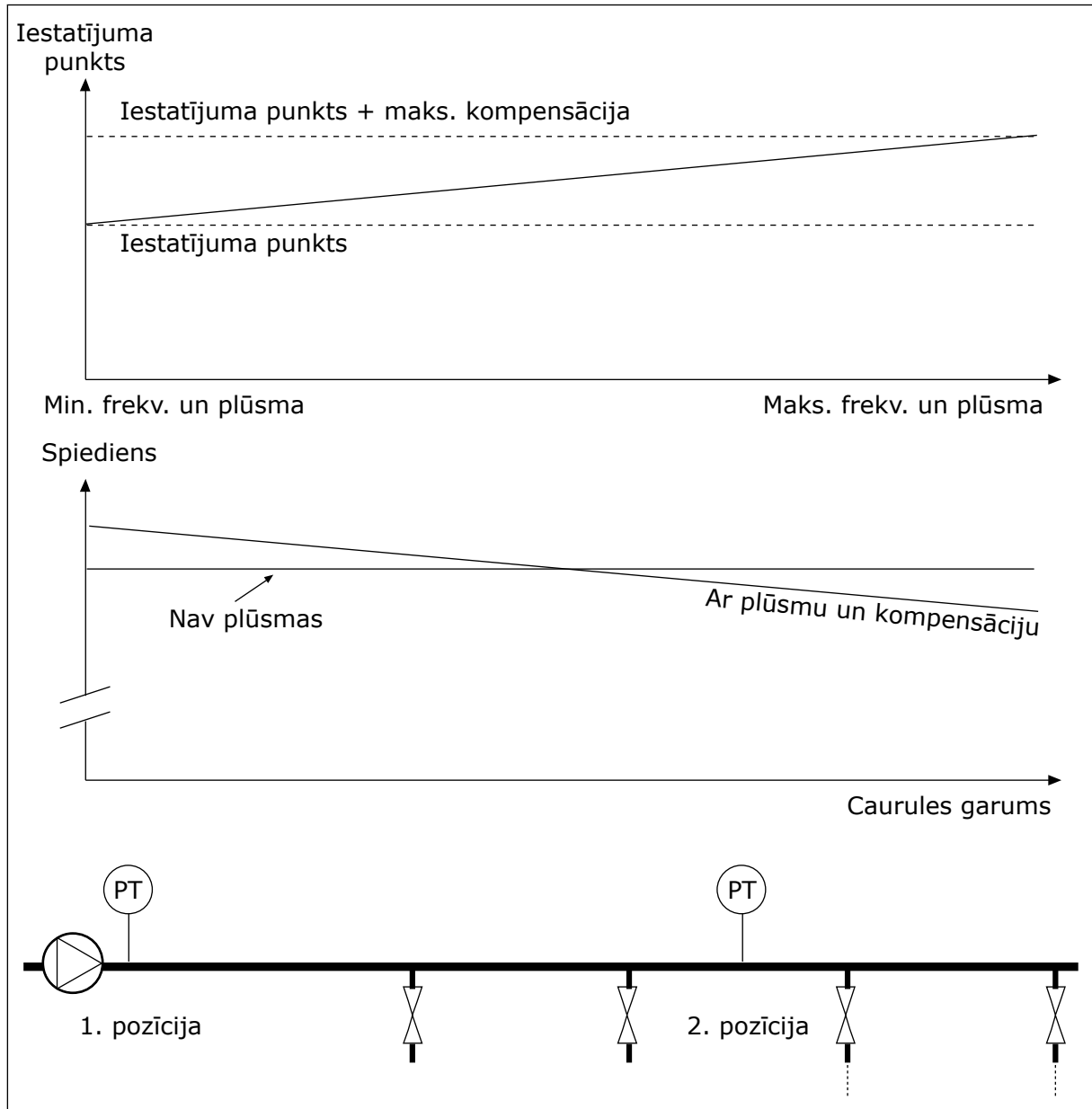
Att. 85: Iespējot spiediena zuduma kompensācijas 1. iestatījuma punktu
