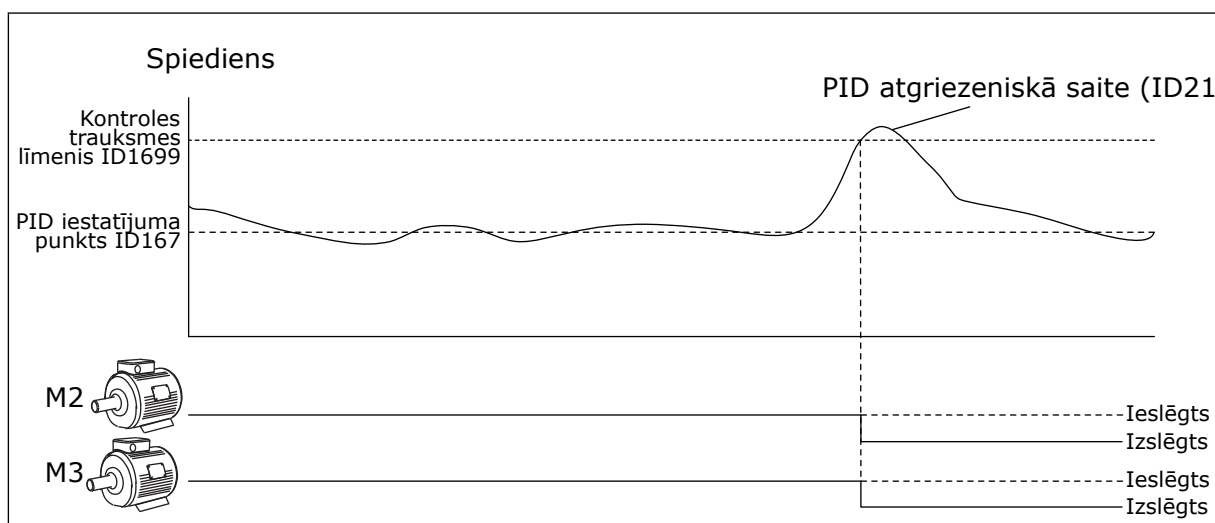
Att. 100: Pārspiediena pārraudzības funkcija
