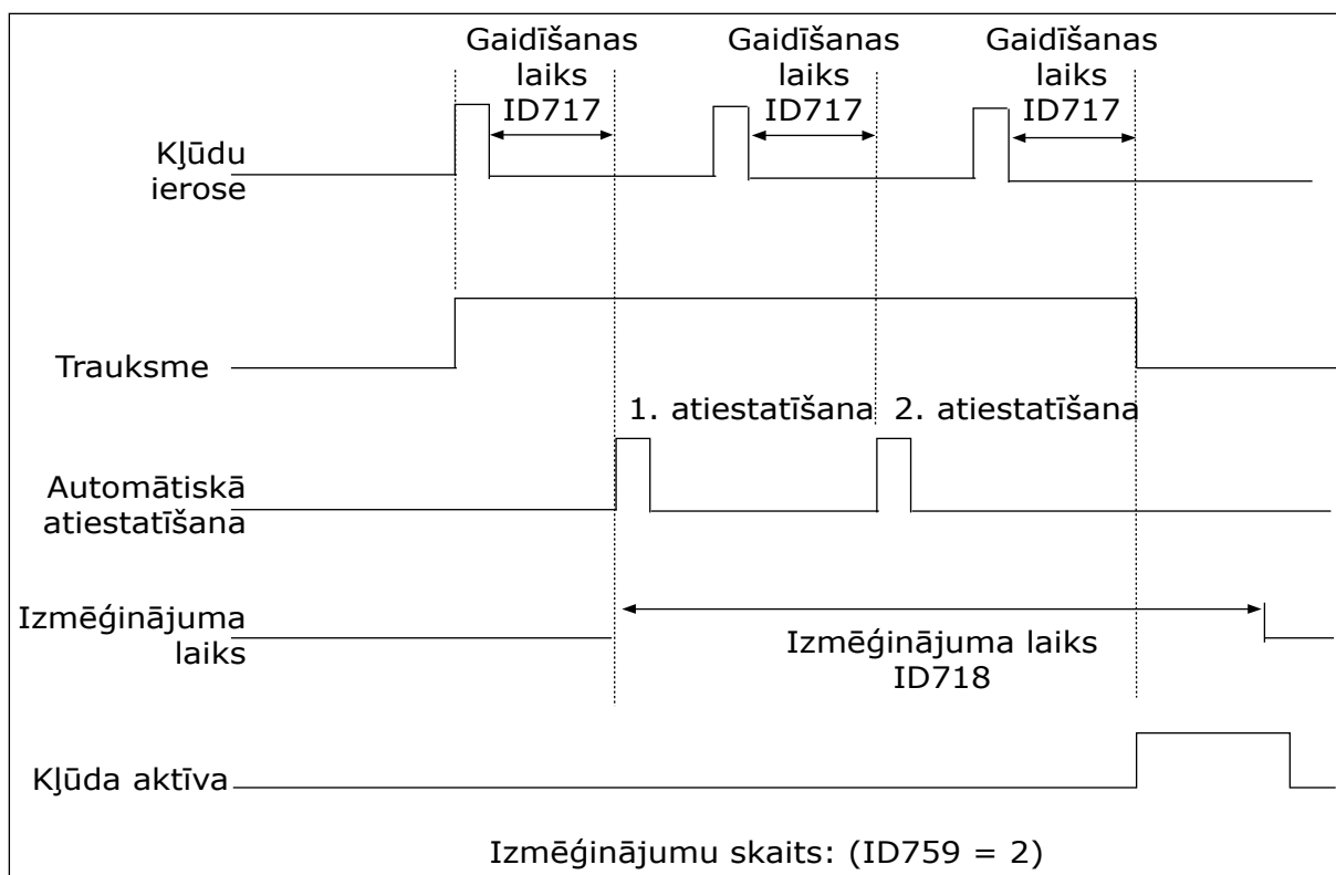
Att. 72: Automātiskās atiestatīšanas funkcija
