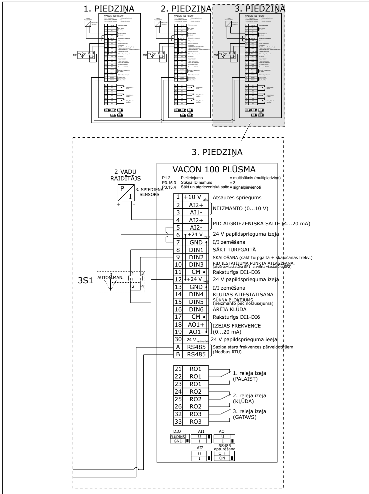
Att. 20: Multisūkņa (multipārveidotāja) sistēmas elektromontāžas shēma, piemērs 1C
