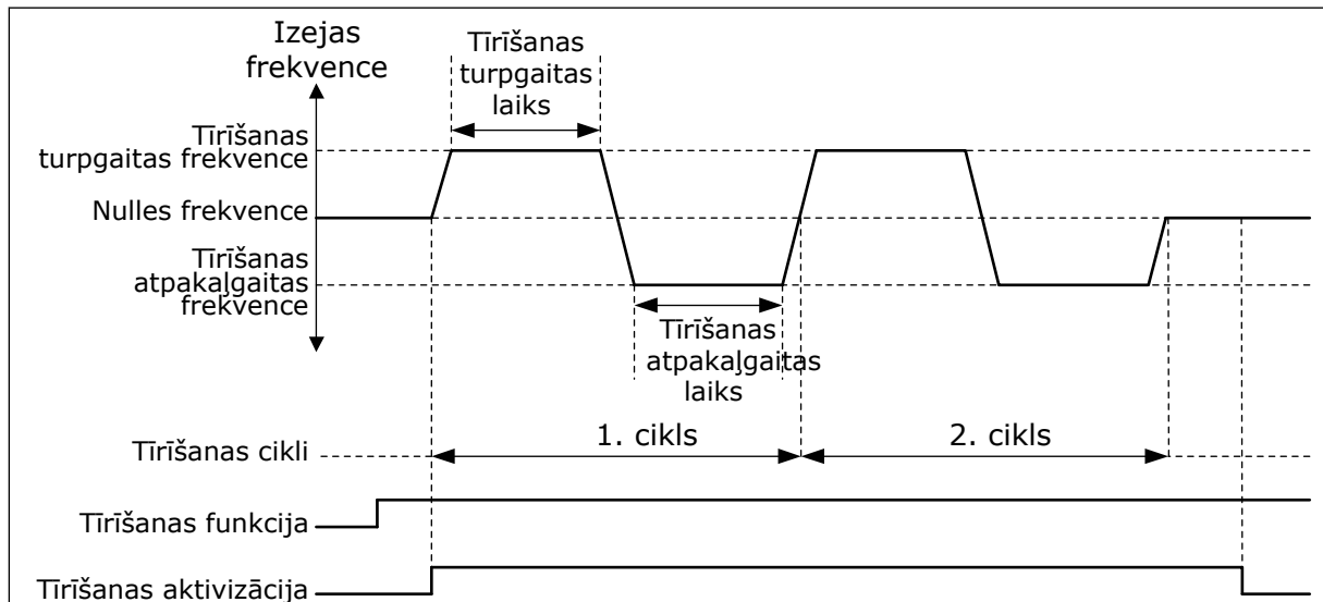
Att. 104: Automātiskās tīrīšanas funkcija
