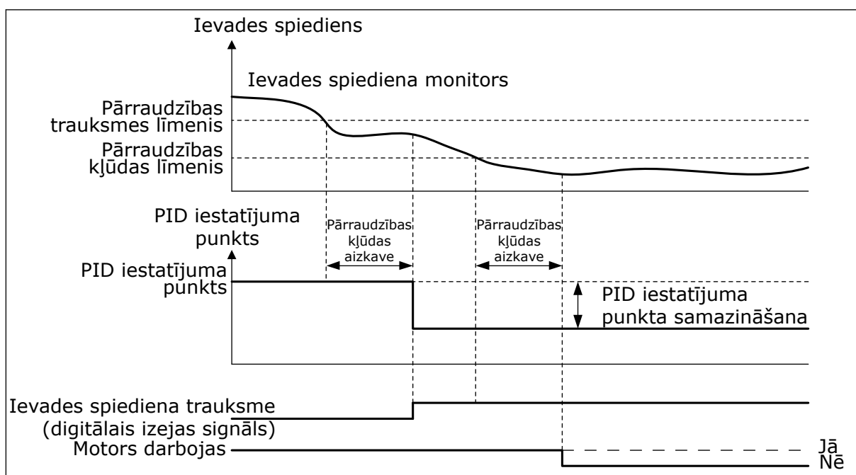
Att. 87: Ievades spiediena pārraudzības funkcija
