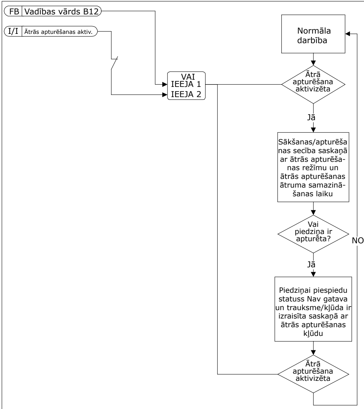
Att. 71: Ātrās apturēšanas loģika
