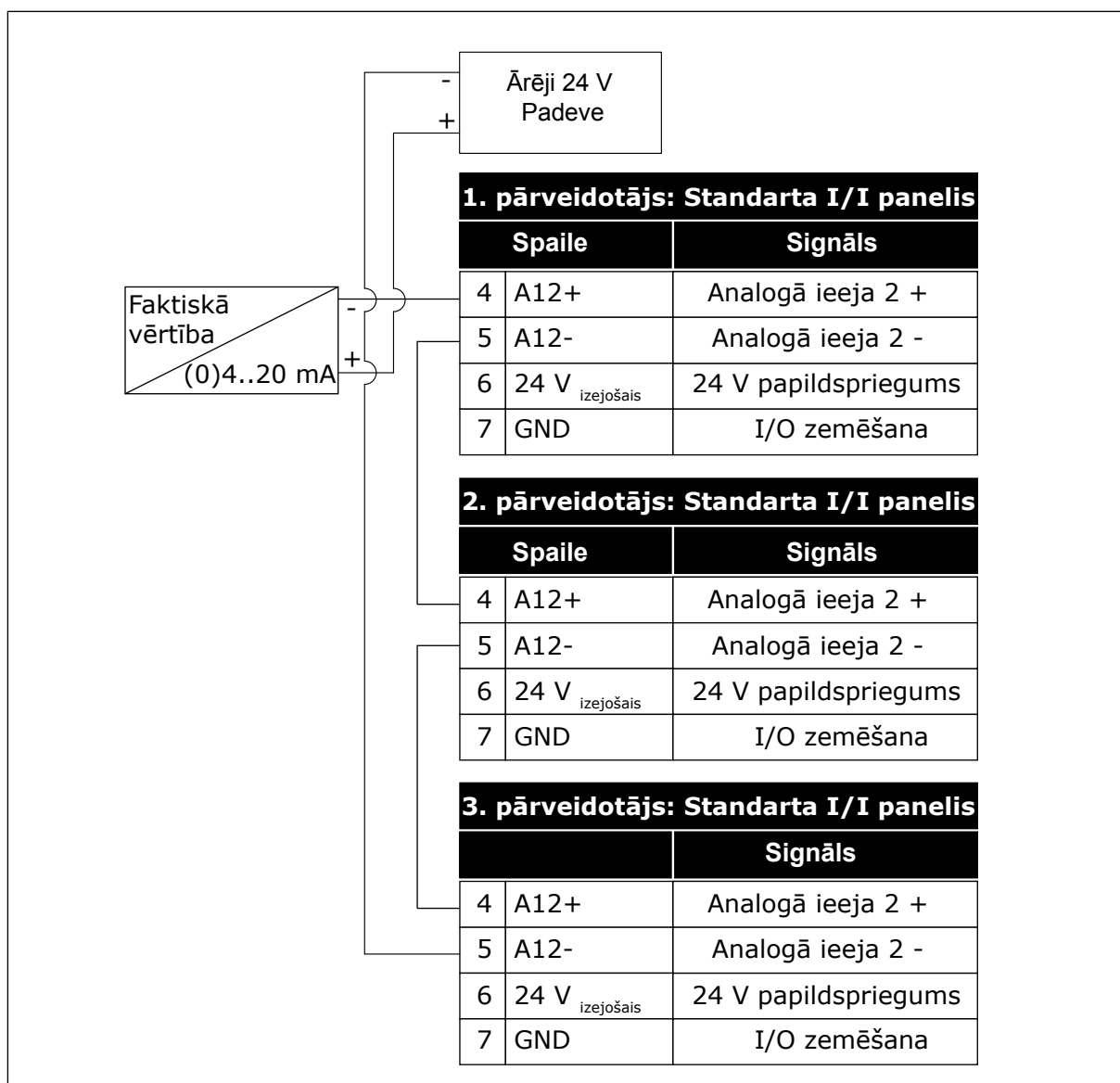
Att. 96: Vadojums, vienu sensoru izmantojot visiem pārveidotājiem (barošana no ārējiem 24 V)
