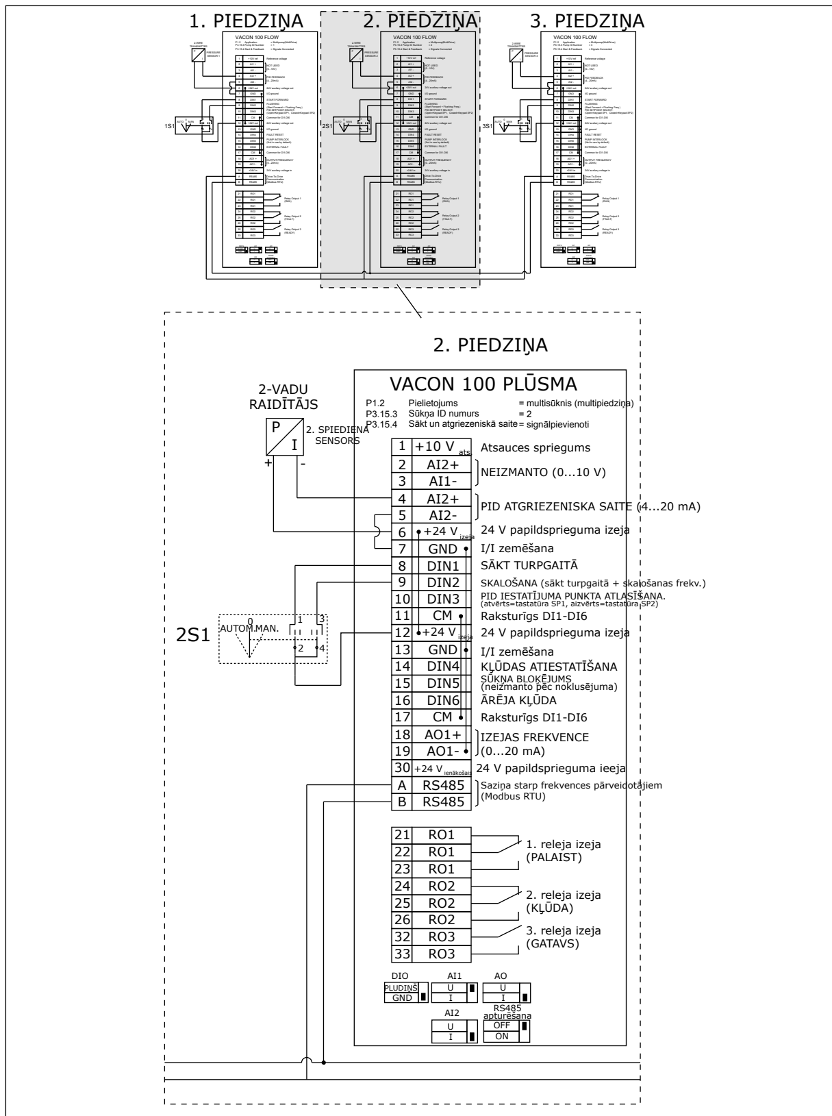
Att. 19: Multisūkņa (multipārveidotāja) sistēmas elektromontāžas shēma, piemērs 1B
