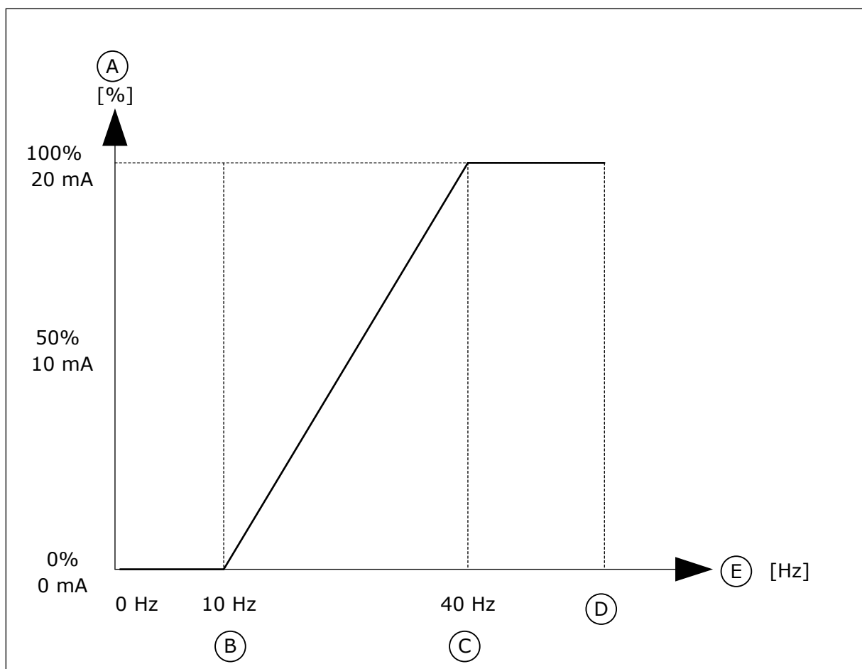
Att. 62: A01 signāla mērogošana
