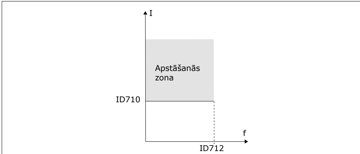
Att. 68: Apstāšanās raksturlielumu iestatījumi
