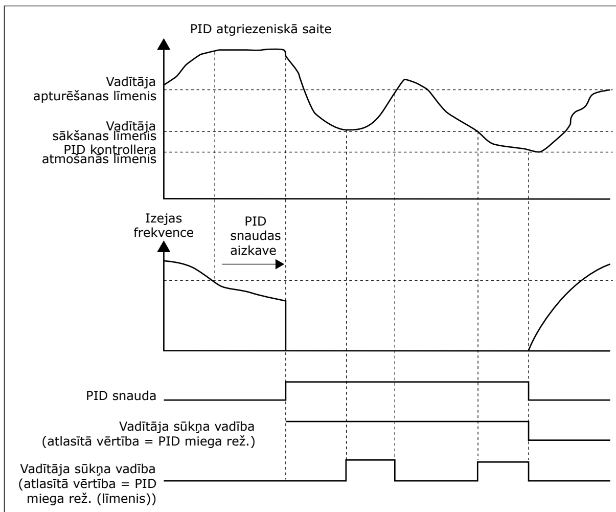
Att. 105: Vadības sūkņa funkcija
