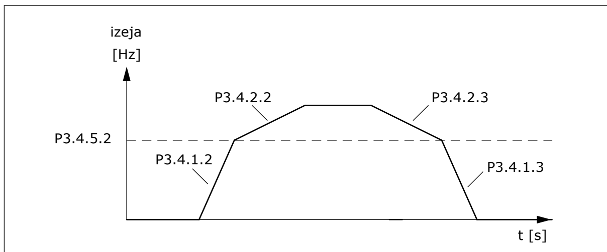
Att. 50: 2. kāpuma aktivizācija, ja izvades frekvence pārsniedz sliekšņa līmeni. (P3.4.5.2 = kāpuma sliekšņa frekvence, P3.4.1.2 = 1. paātrinājuma laiks, P3.4.2.2 = 2. paātrinājuma laiks, P3.4.1.3 = 1. palēninājuma laiks, P3.4.2.3 = 2. palēninājuma laiks)
