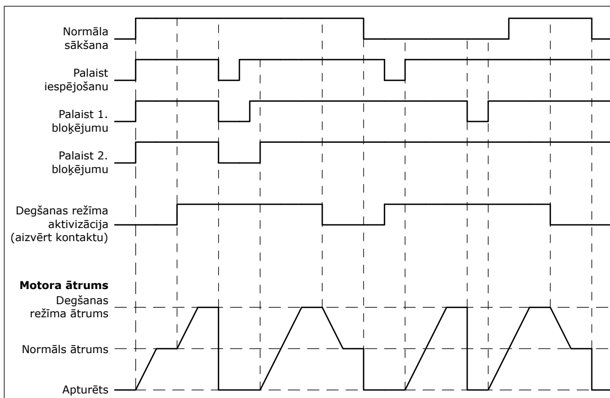
Att. 103: Degšanas režīma funkcija
