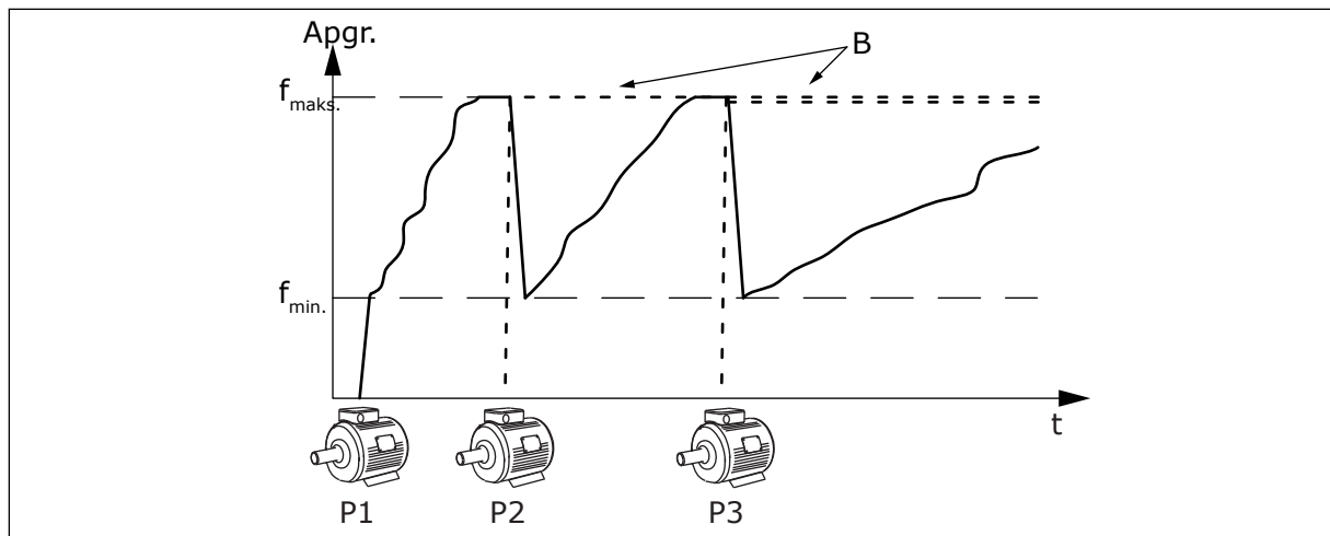
Att. 91: Vadība viena pārveidotāja režīmā
