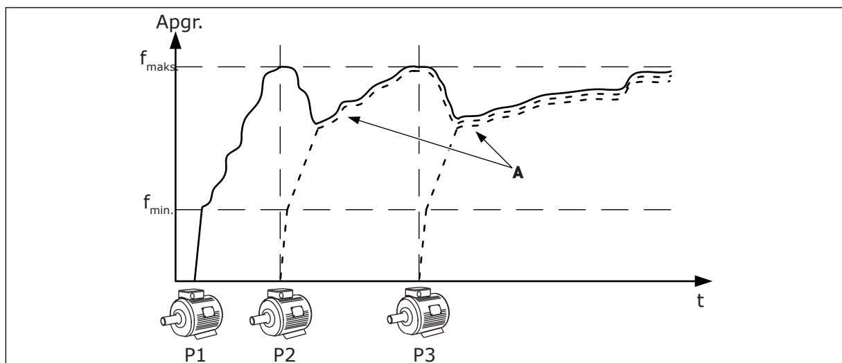
Att. 92: Vadība multisekotāja režīmā
