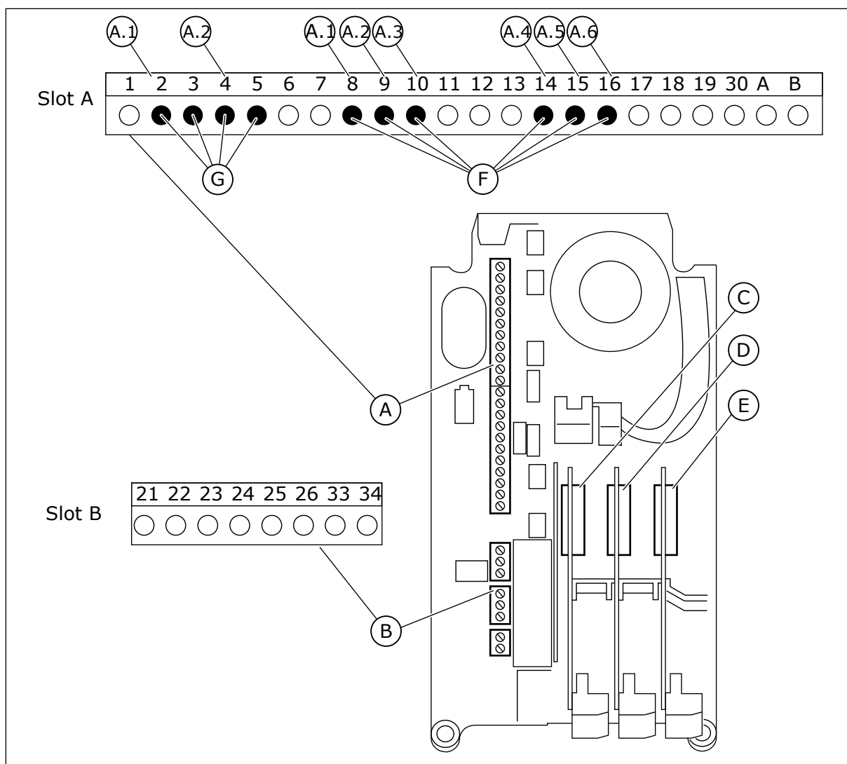
Att. 51: Papildu plates sloti un programmējamās ievades
