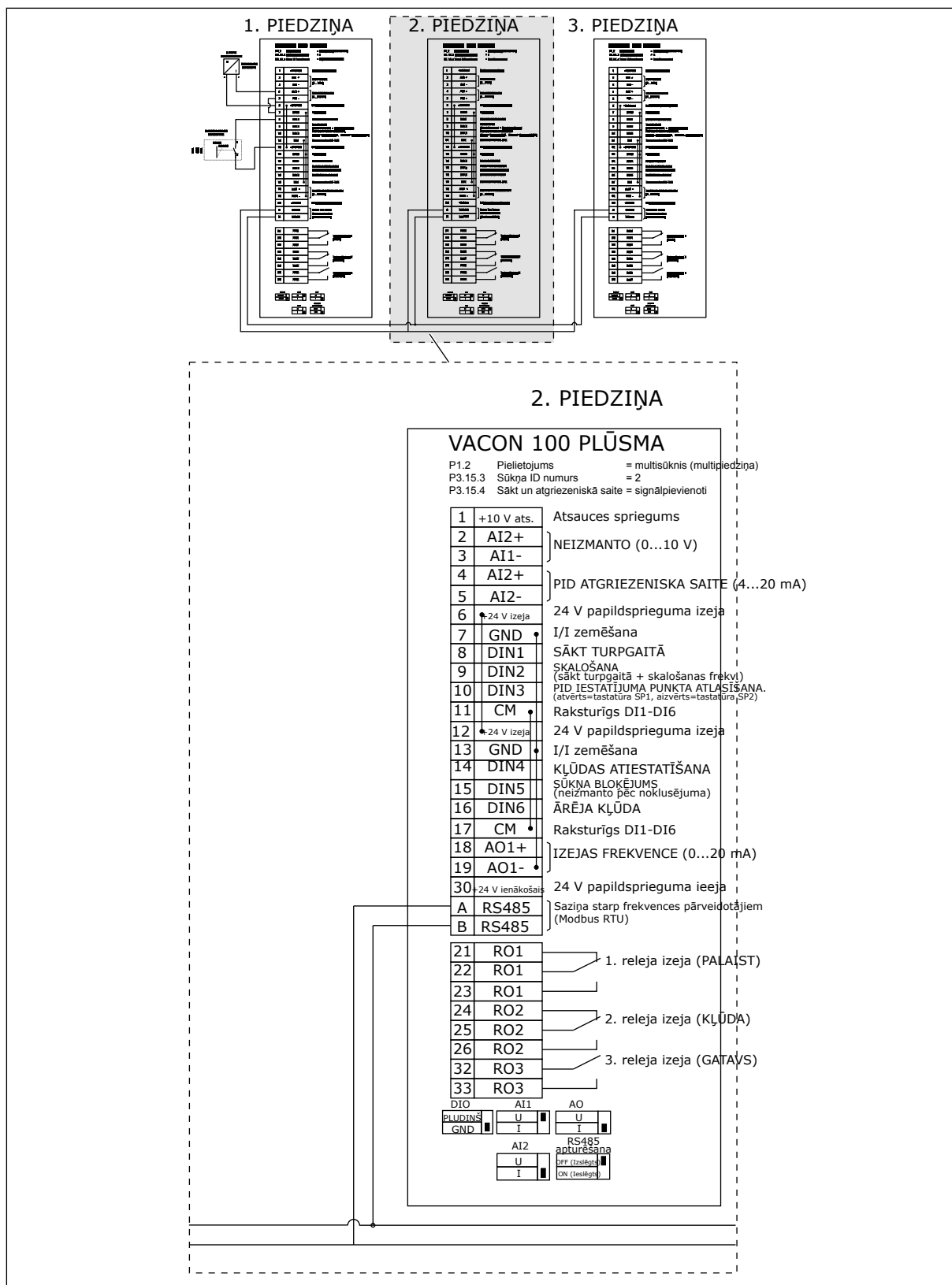
Att. 31: Multisūkņa (multipārveidotāja) sistēmas elektromontāžas shēma, piemērs 5B
