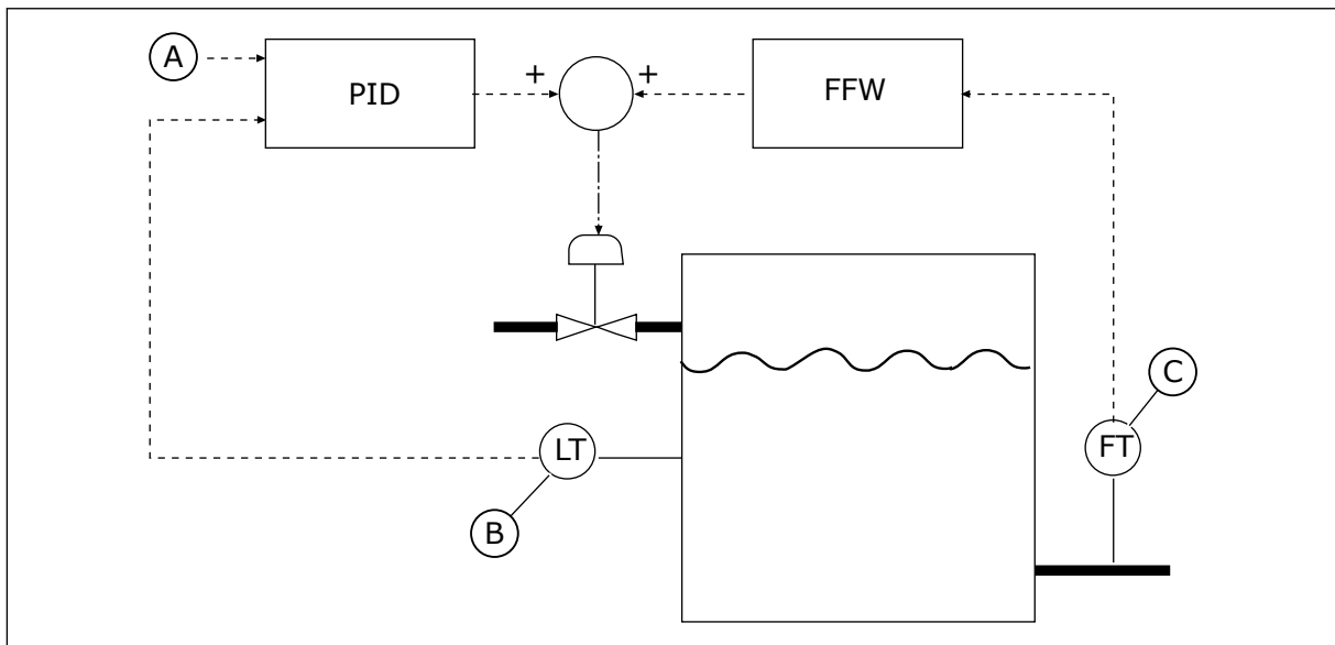
Slika 80: Nadzor FeedForward
