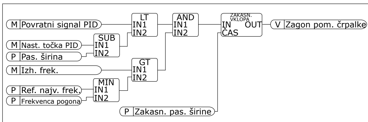
Slika 101: Frekvenca pogona
