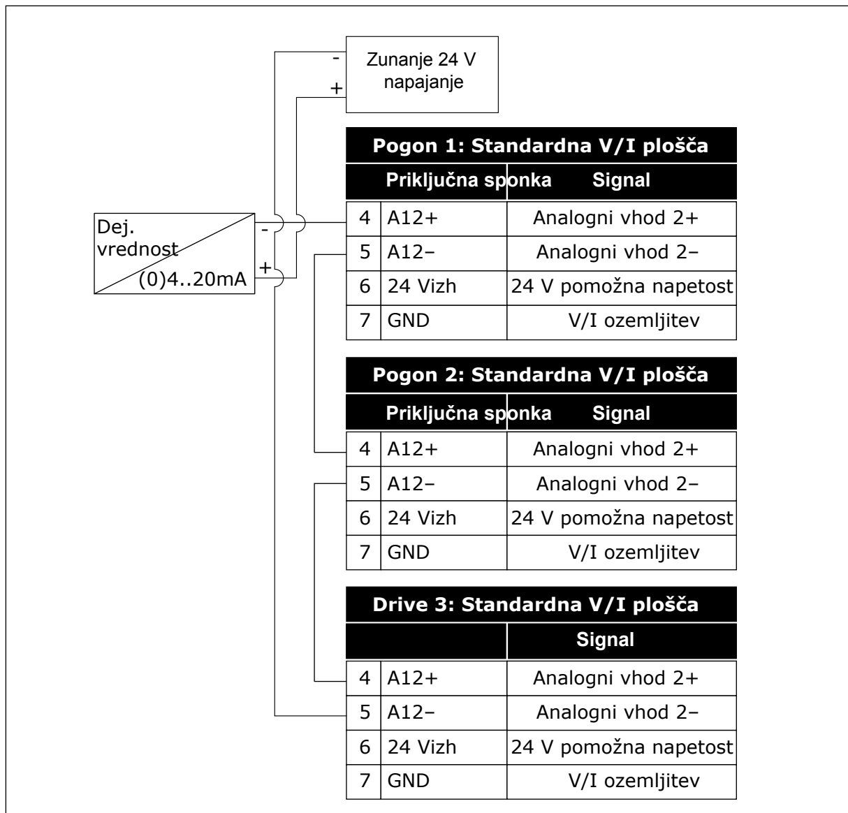
Slika 96: Ožičenje istega senzora za vse pretvornike (z zunanjim virom 24-voltnega napajanja)
