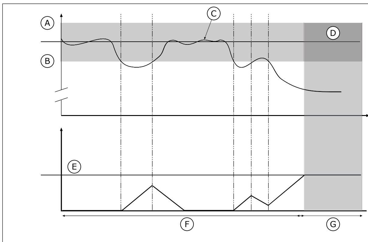
Ábra 83: Az Ellenőrzőjel-felügyelet funkció
