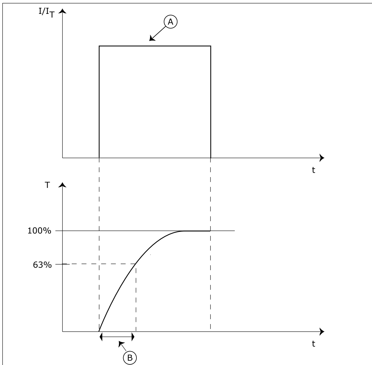
Ábra 66: A motor termikus időállandója
