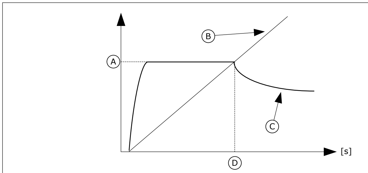
Ábra 40: Az I/f-indítás paramétere
