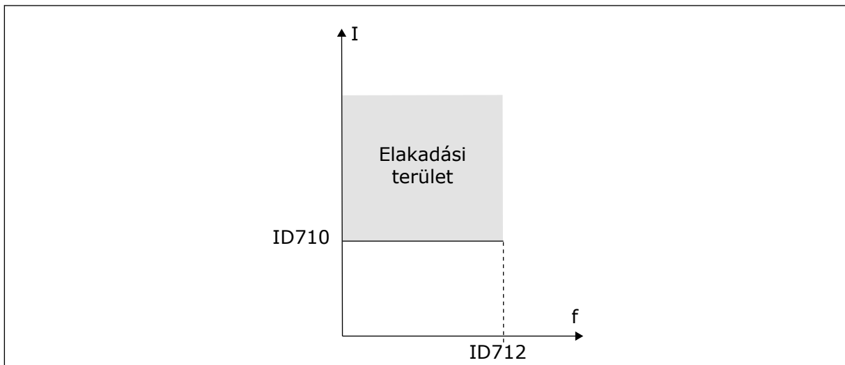
Ábra 68: Elakadási beállítások
