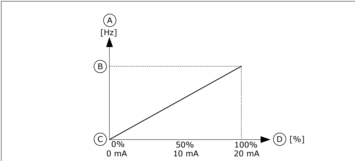
Ábra 60: A11 jel invertálása, 0 beállítva
