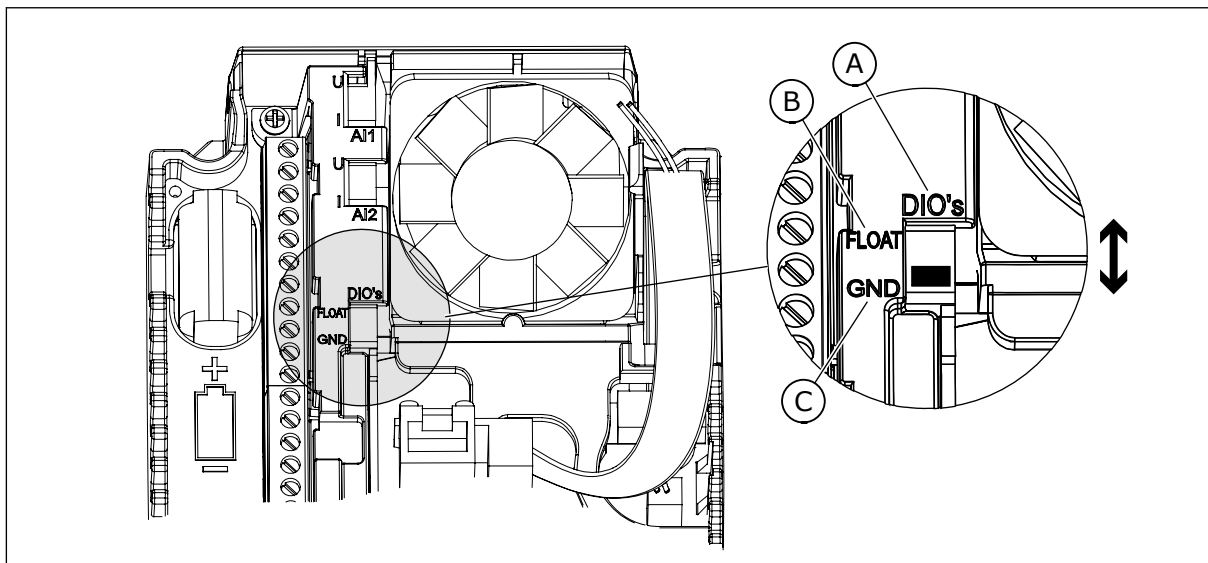
Ábra 17: DIP-kapcsoló
