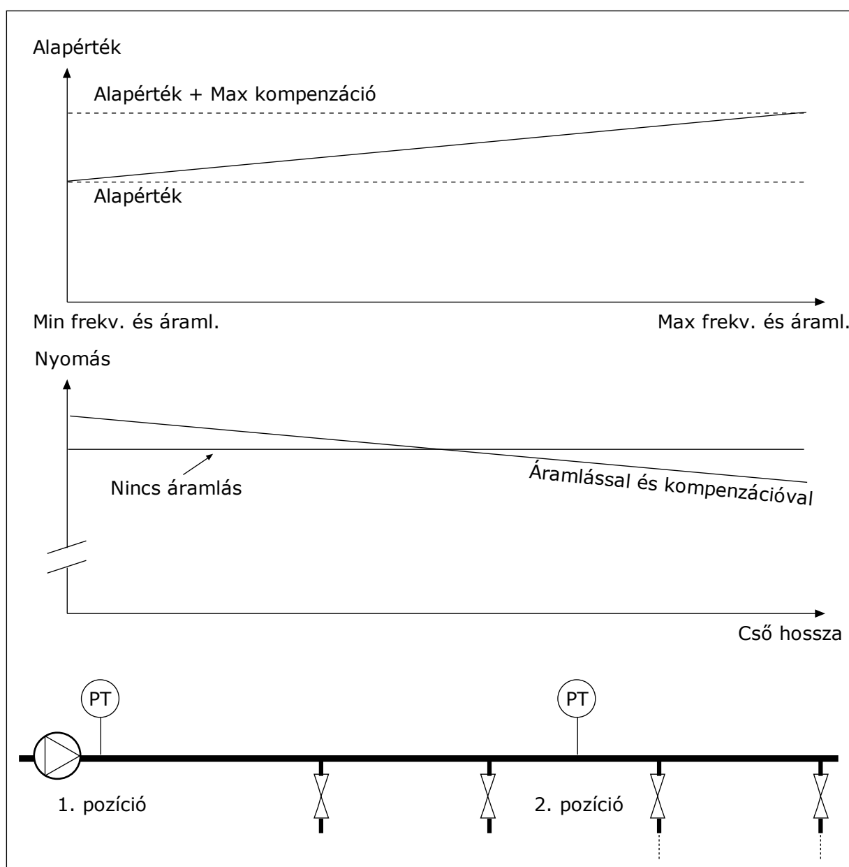
Ábra 85: 1. alapérték nyomásvesztés-kompenzációjának engedélyezése
