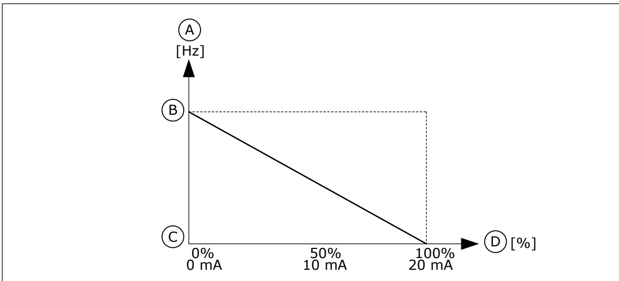
Ábra 61: A11 jel invertálása, 1 beállítva
