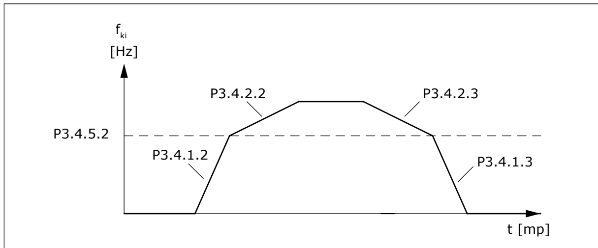
Ábra 50: A 2. rámpa aktiválása, amikor a kimeneti frekvencia a küszöb szintje felé emelkedik. (P3.4.5.2 = Rámpa küszöbfrekv., P3.4.1.2 = 1. indulási idő, P3.4.2.2 = 2. indulási idő, P3.4.1.3 = 1. leállási idő, P3.4.2.3 = 2. leállási idő)
